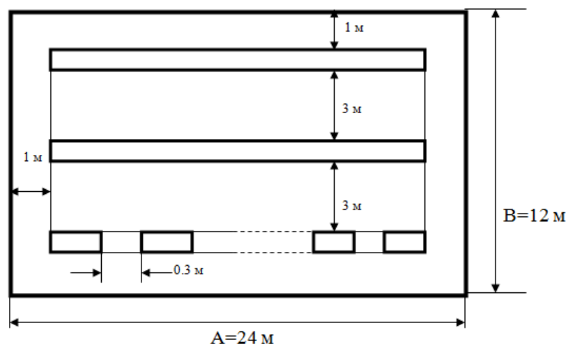
Рисунок 39 – План производственного помещения
