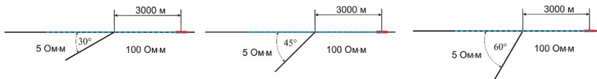
Рис. 1. Модели среды с наклонной границей
