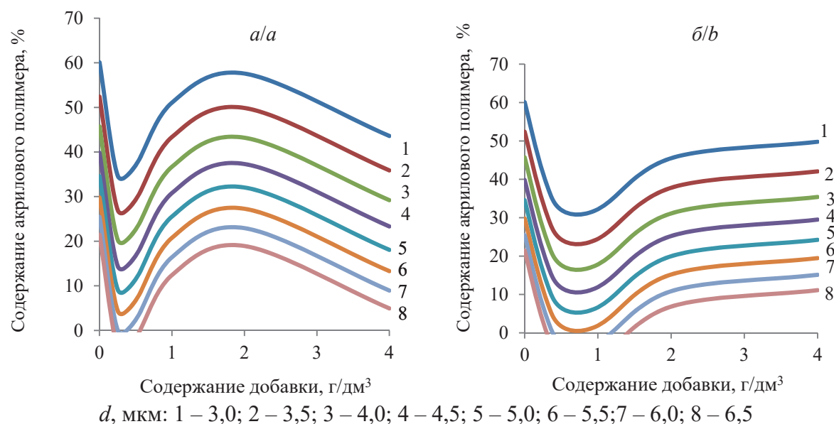
Рис. 5. Влияние содержания акрилового полимера и добавок: Glide 100 (а) и Dispers 715w (б) на среднестатистический диаметр частиц пигмента
