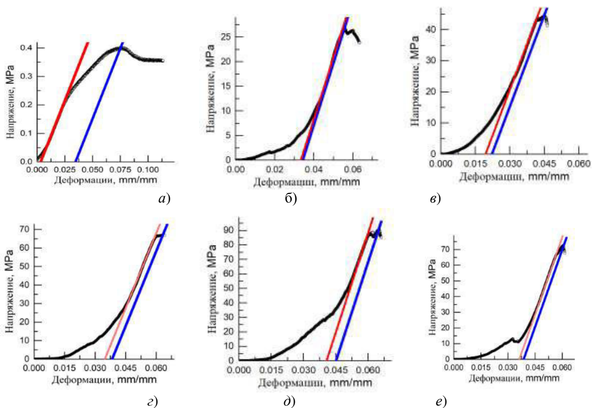
Рис. 1. Деформационные кривые напряжение-деформация ( \sigma - \epsilon ) после 4 часов (а), 1 суток (б), трех суток (в), 7 дней (г), 14 (д) и 28 (е) дней твердения. Красная линия – оценка модуля упругости, проходящая через предел текучести, синяя – через предел прочности
