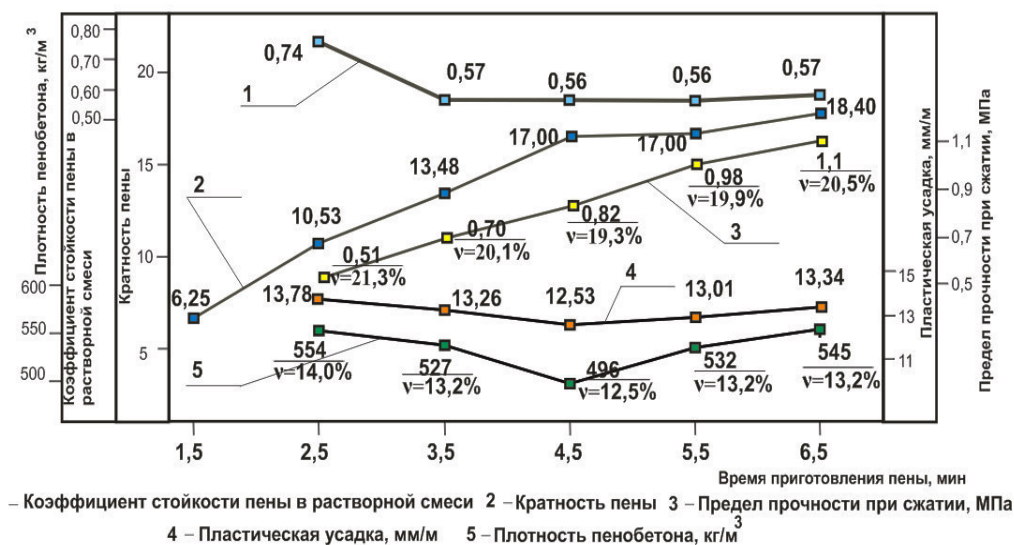
Рис. 2. Влияние времени приготовления пены на свойства пены и пенобетона
