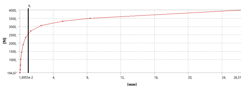
Рис. 3. Зависимость прилагаемой силы от деформации до и после потери устойчивости
