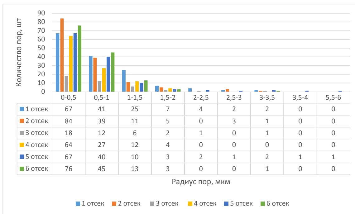
Рис. 3. Гистограмма количественного содержания пор каждого образца-куба
