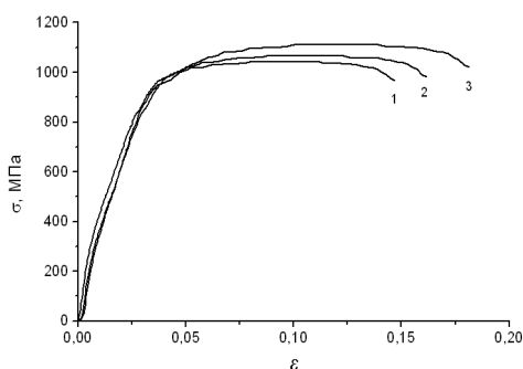
Рис.1. Диаграммы растяжения в координатах «напряжение–пластическая деформация» поликристаллов сплавов ВТ16 при 300 К: 1 – образцы без водорода, кривые 2 - наводороженные образцы при постоянном потенциале в течение 8 ч, кривые 3 - наводороженные образцы при постоянном потенциале в течение 24 ч
