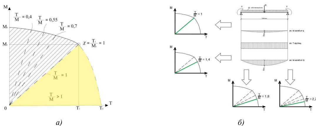
Рис. 4. а) график отношения крутящего момента к изгибающему, б) программа эксперимента
