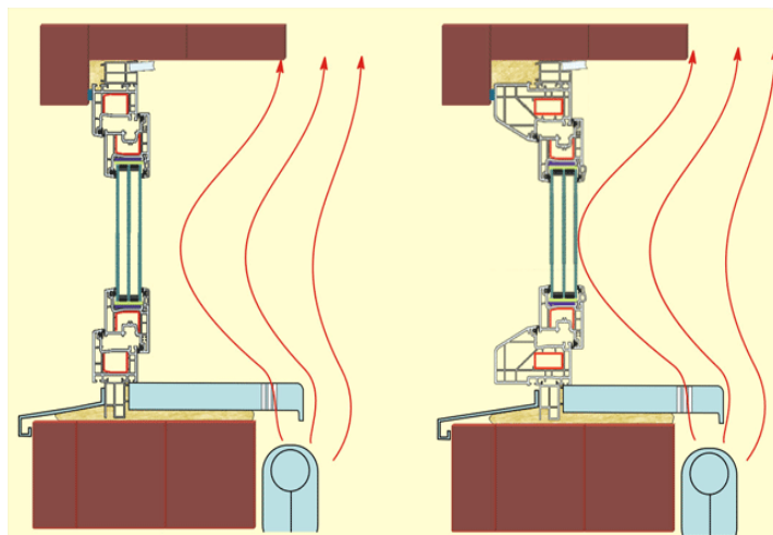
Рис. 2. Сравнение стандартной оконной системы и оконной системы с более широкой оконной коробкой
