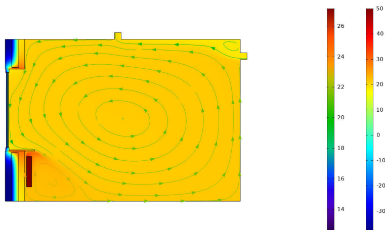
Рис.3. Температурное состояние модели при свободной конвекции с прогревом оконного пространства.
