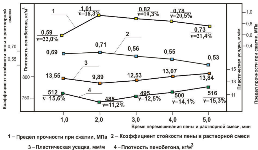
Рис. 3. Влияние времени перемешивания пены и растворяющей смеси на свойства пены и пенобетона
