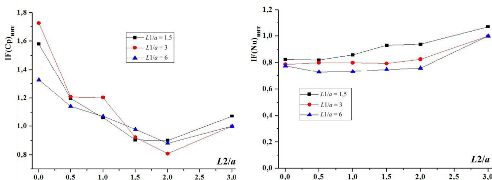
Рис. 2. Фактор динамической (а) и тепловой (б) интерференции, определенный по интегральным значениям коэффициентов давления C_p и чисел Нуссельта Nu
