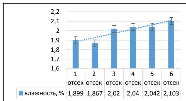
Рис. 1. График распределения влажности по длине модели-балки
