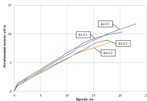
Рис. 3. Зависимость прогиба от величины изгибающего момента
