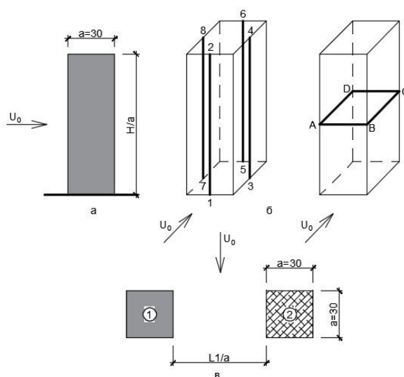
Рис. 2. Схема расположения моделей относительно ветрового потока и обозначение граней модели: а – вид сбоку; б – сечения модели «2» по граням; в – план расположения моделей
