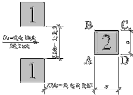
Рис. 1. Схема расположения исследуемой модели «2» относительно моделей «1» при поперечном смещении L1/a и продольном смещении L2/a (угол атаки \varphi = 0^\circ )
