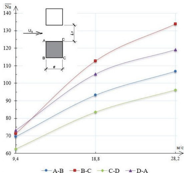
Рис. 3. Средний по граням внешний теплообмен модели «2» с относительной высотой H/a = 5 при \varphi = 0^\circ и L1/a = 2
