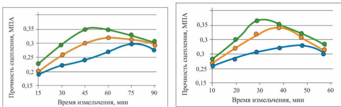
Рис. 1,2. Влияние способа и времени механизации на прочность сцепления торфяного вяжущего (торф низинный): а-измельчение в ШМ; б-измельчение в ПМ: 1-сухой помол; 2-в воде; 3-в воде при температуре 90 С
