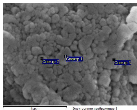
Рис. 3. Структура геополимербетона №2 на шлаке с удельной поверхностью 584 м 2 /г
