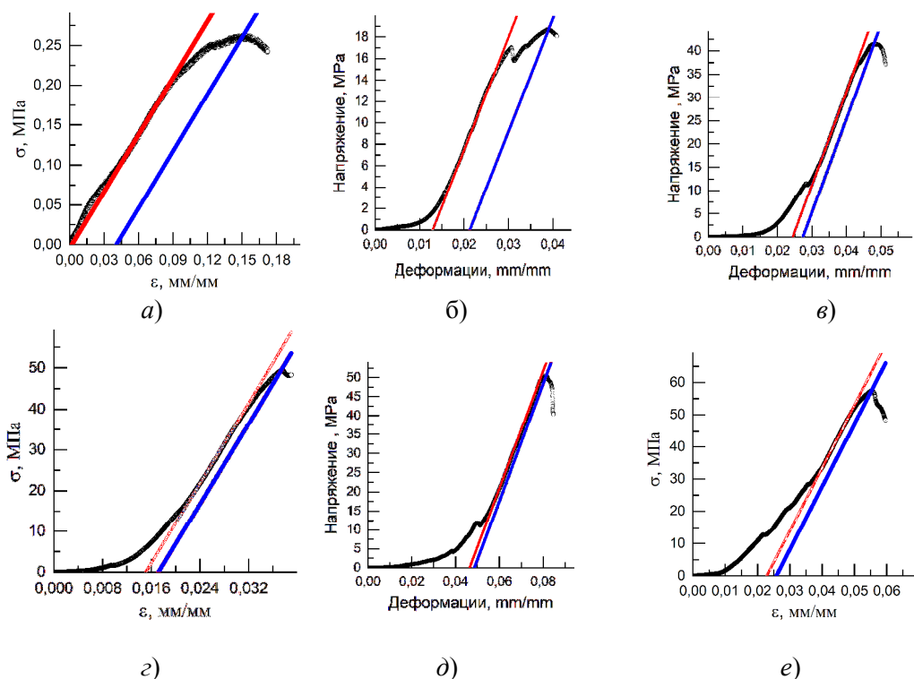
Рис. 1. Деформационные кривые напряжение-деформация ( \sigma - \epsilon ) после 4 часов (а), 1 суток (б), трех суток (в), 7 дней (г), 14 (д) и 28 (е) дней твердения. Красная линия – оценка модуля упругости, проходящая через предел текучести, синяя – через предел прочности
