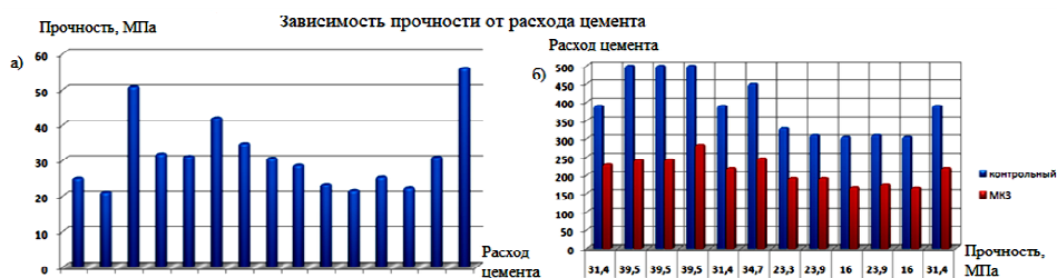
Рис. 2. а) диаграмма зависимости прочности от расхода цемента с микрокремнеземом
