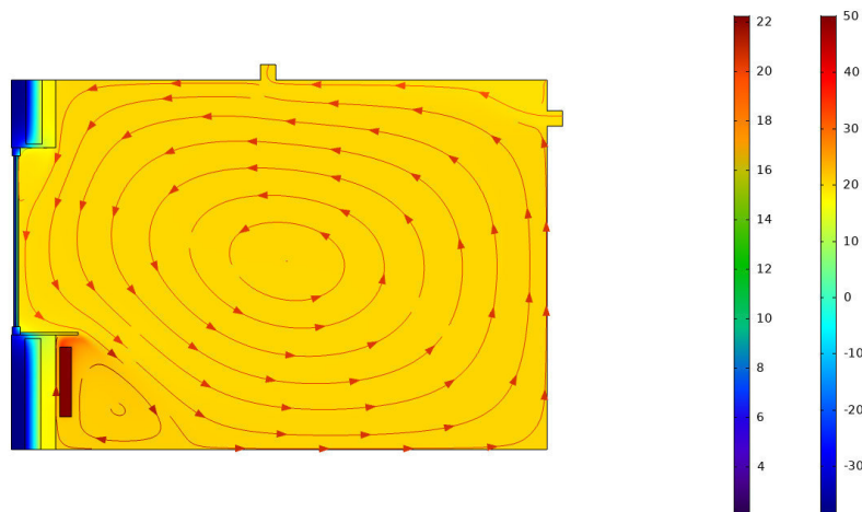
Рис.2. Температурное состояние модели при свободной конвекции без прогрева оконного пространства
