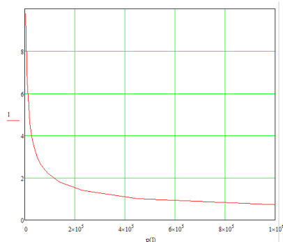
Рис 1. Критические нагрузки стойки, при превышении которых возникают нелинейные деформации
