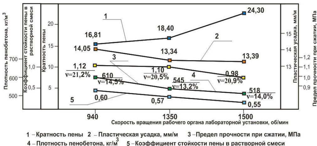
Рис. 1. Влияние скорости вращения лабораторной установки на свойства пены и пенобетона
