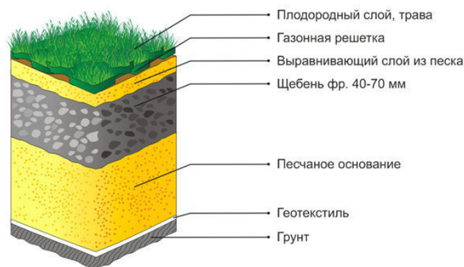
Рис. 1. Строение покрытия экопарковки
