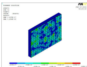
Рис.7 Теплообмен в стене «кирпич и пено-стеклокерамика»
