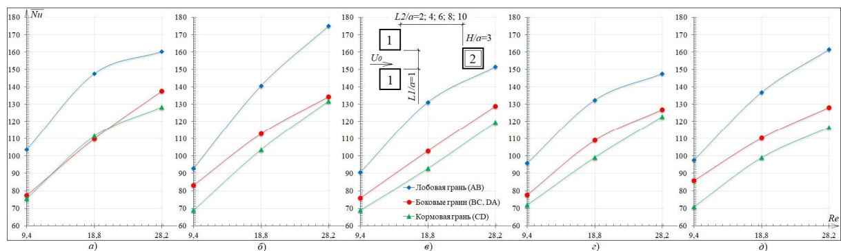
Рис. 2. График влияния скорости воздушного потока и продольного смещения на распределение среднего по граням числа Нуссельта для модели с относительной высотой H/a = 3 ; \angle\varphi = 0^\circ ; L1/a = 1 :
