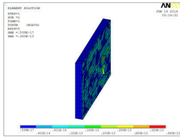
Рис.5 Теплопередача в стене «железобетон и пенобетон»
