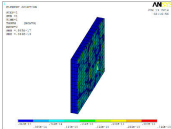
Рис.6 Теплообмен в стене «кирпич и пенобетон»
