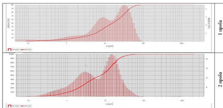
Рис. 1. Интегральные кривые зернового состава шлака
