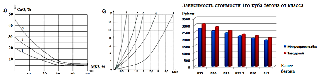
Рис. 3. а) содержание свободной извести в образцах цементного камня с различными дозировками МКЗ. б) цемент без добавок; 2- цемент + 10% МКЗ; 3- цемент + 20% МКЗ; 4- цемент + 30% МКЗ; 5- цемент + 40% МКЗ; в) зависимость стоимости 1 куба бетона от класса
