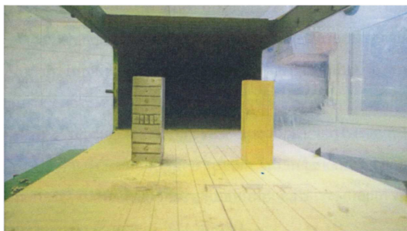
Рис. 1. Общий вид расположения моделей в рабочей камера аэродинамической трубы: слева – измерительная модель «2», справа – модель «1»
