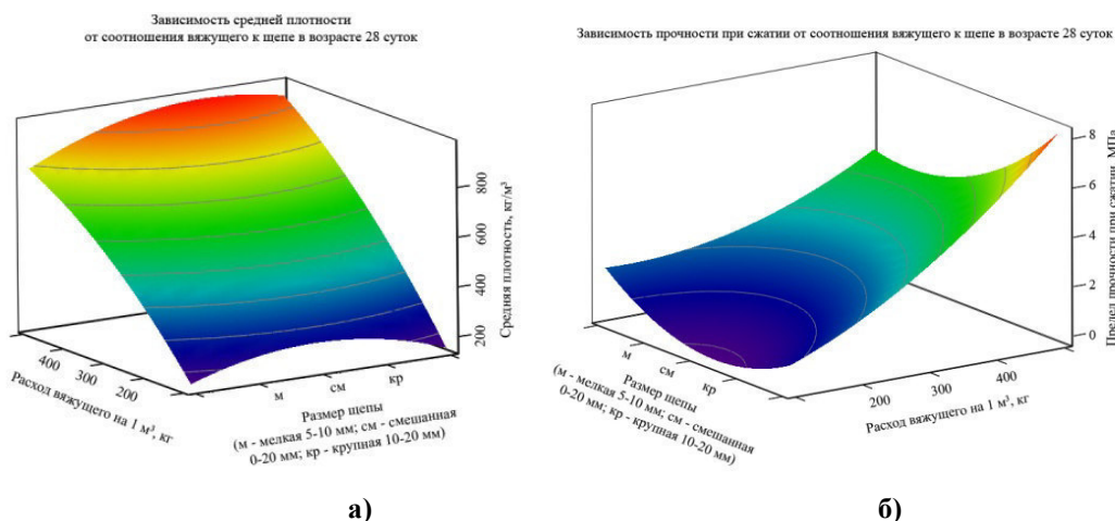
Рис.2. Зависимость средней плотности(а) и прочности на сжатие(б) соотношением вяжущего(ГИЦВ) к щепе в возрасте 28 суток
