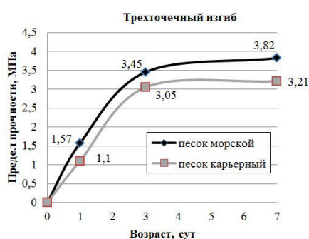
Рис. 3. Прочность на трехточечный изгиб
