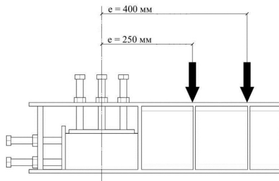
Рис. 2. Приложение нагрузки на захваты
