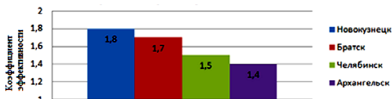
Рис. 1. Эффективность микрокремнезема разных заводов
