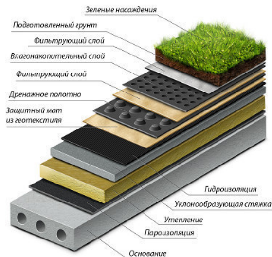
Рис. 2. Устройство зелёной кровли
