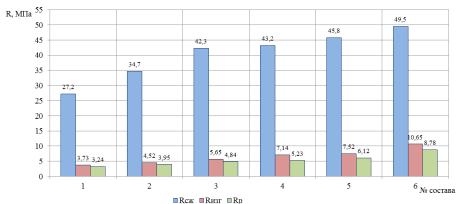
Рис. 1. Диаграмма показателей предела прочности на сжатие, растяжение при изгибе, растяжение при раскалывании
