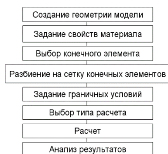
Рис.1 Основные этапы расчета в ANSYS
