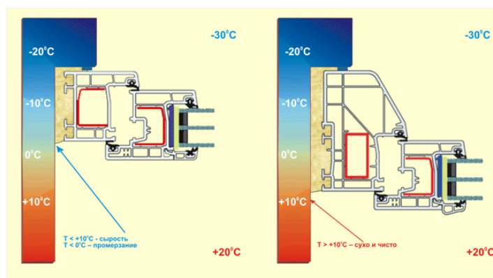
Рис. 1. Температурные поля при стандартной и широкой оконной коробке
