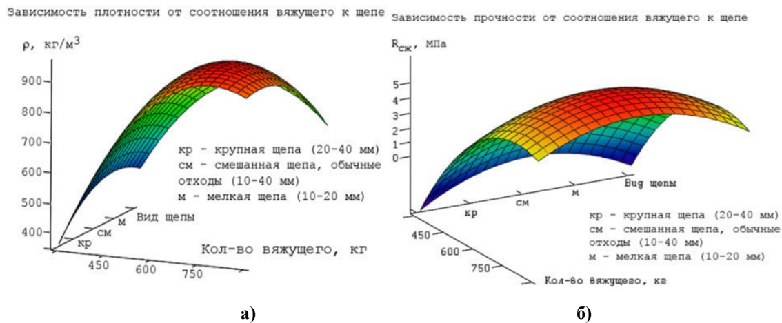
Рис.1. Зависимость средней плотности(а) и прочности на сжатие(б) соотношением вяжущего(ГИЦВ) к щепе в возрасте 28 суток
