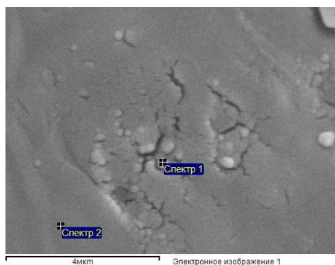
Рис. 2. Структура геополимербетона № 1 на шлаке с удельной поверхностью 285 м 2 /г
