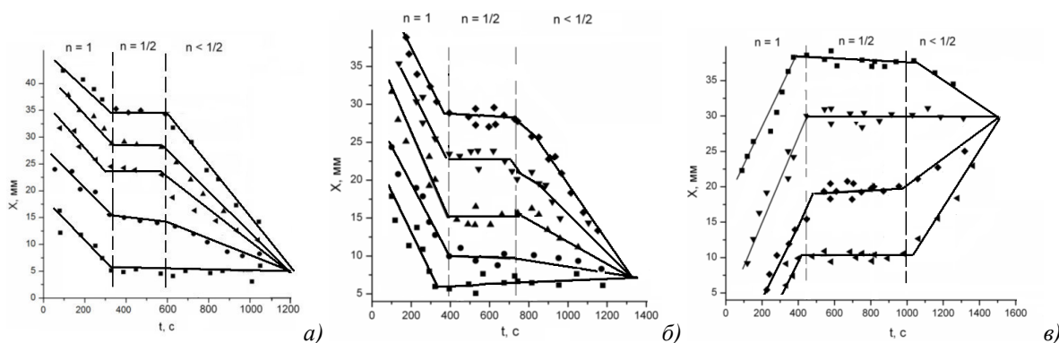
Рис.2. Диаграмма пространственно-временной эволюции очагов локализованной деформации \epsilon_{xx} при растяжении образца сплава ВТ16 без водорода (а), при насыщении водородом в течение 8 часов (б) и 24 часов (в)
