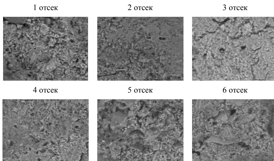
Рис. 2. Структура цементного камня по отрезкам, увеличенная в 2000 раз
