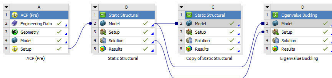
Рис. 2. Структура передачи данных для нелинейного расчета
