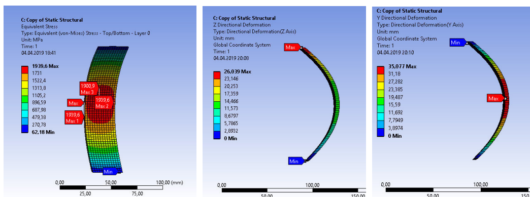
Рис. 4. а) напряжения по von-Mises, б) продольная и поперечная деформация при сжатии 4000 Н
