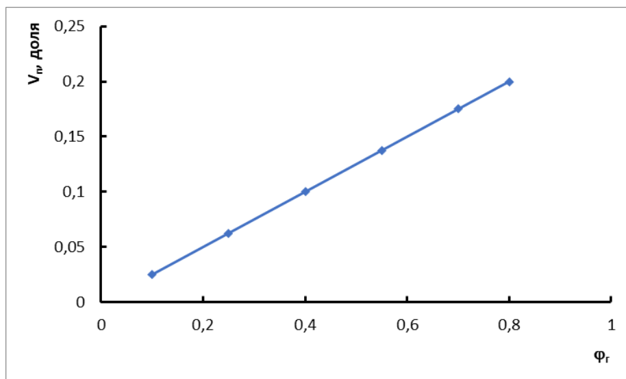
Рисунок 3.31 – Теоретический график зависимости доли жидкости в пограничном слое от газосодержания в барботажном реакторе
