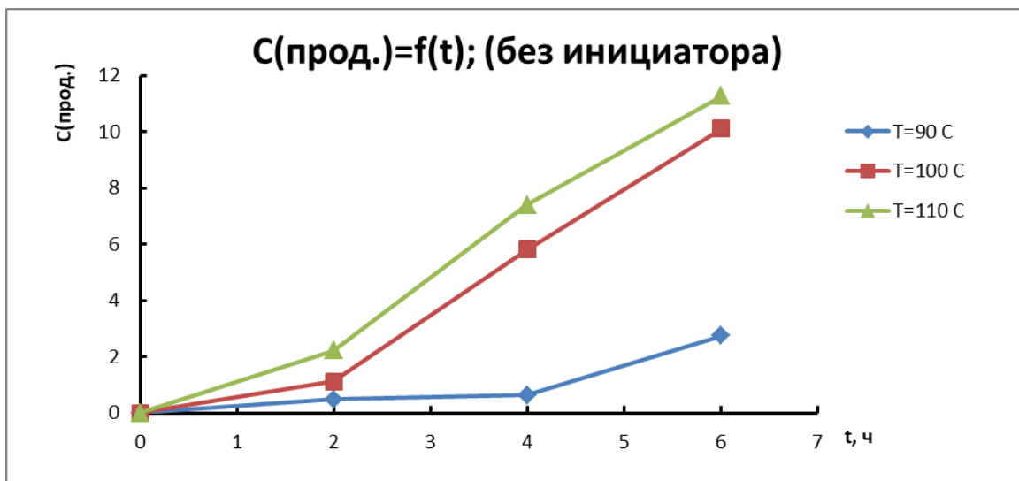
Рисунок 3.3 – Образование эпоксидов при низком расходе без инициатора
