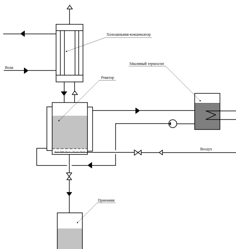
Рисунок 2.1 – Схема установки
