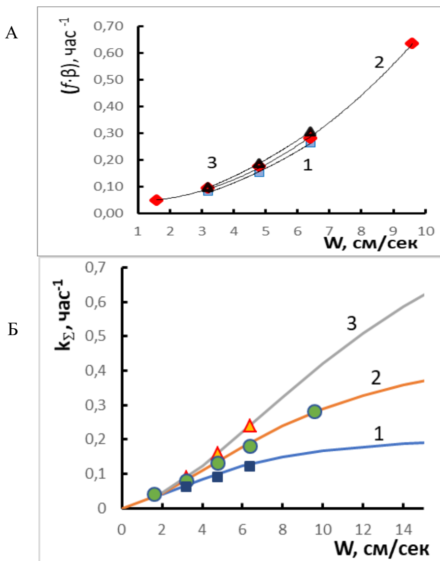
Рисунок 3.15 – Изменение коэффициента массоотдачи ( f \cdot \beta ) (символы) и полиномиальные линии тренда (А) и зависимости суммарной константы скорости ( k_{\Sigma} ) (символы) и расчетные кривые по уравнению (2) (Б) в зависимости от приведенной линейной скорости барботируемого воздуха при температурах 100, 110 и 120 °С (кривые 1, 2 и 3, соответственно)
