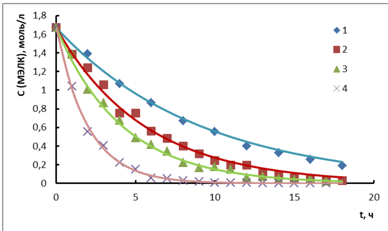
Рисунок 3.13 – Влияние различных режимов барботирования. Экспериментальные точки и аппроксимирующие кривые расходования МЭЖК при T = 110\text{ }^{\circ}\text{C} : полая колонна, подача воздуха в пузырьковом режиме, 5 мл/с, (кривая 1); колонна с насадкой с подачей воздуха 10 мл/с (кривая 2); режим динамической ячеистой пены (30 мл/с) (кривая 3); расходование МЭЖК в реакторе с мешалкой (кинетическая область, кривая 4)
