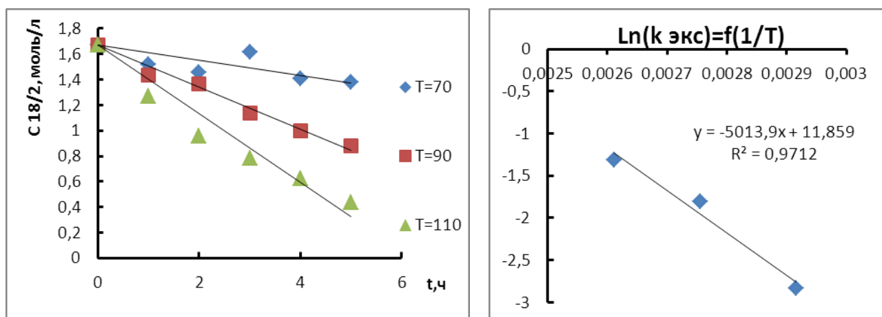
Рисунок 3.11 – Зависимость концентрации исходных компонентов сырья от времени (слева) и температурная зависимость константы скорости в Аррениусовских координатах (справа)
