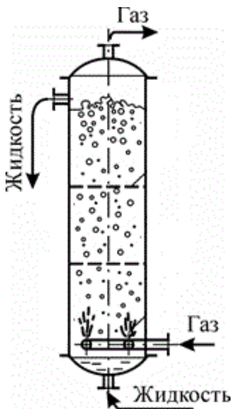
Рисунок 3.32 – Эскиз барботажного реактора
