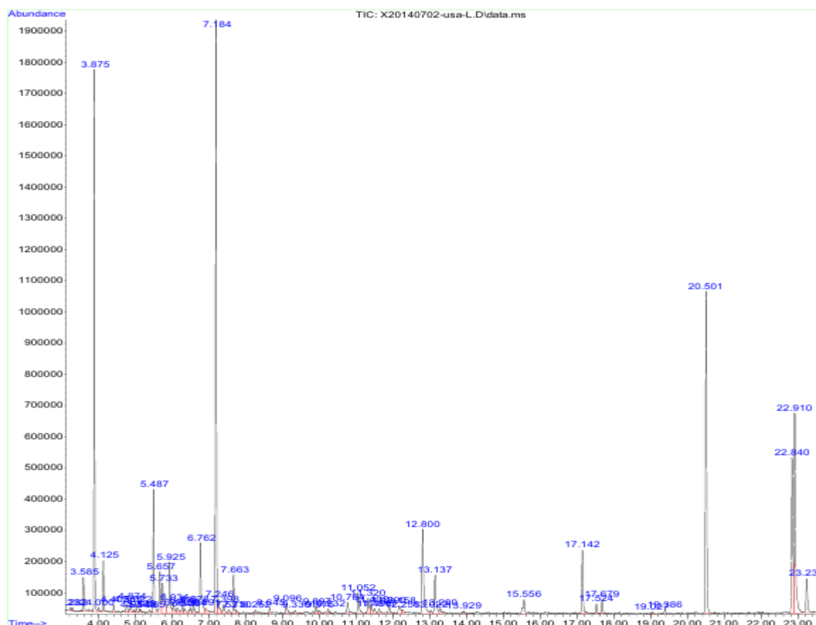
Рисунок 3.19 – Хроматограмма потока, уносимого воздухом при барбатаже
