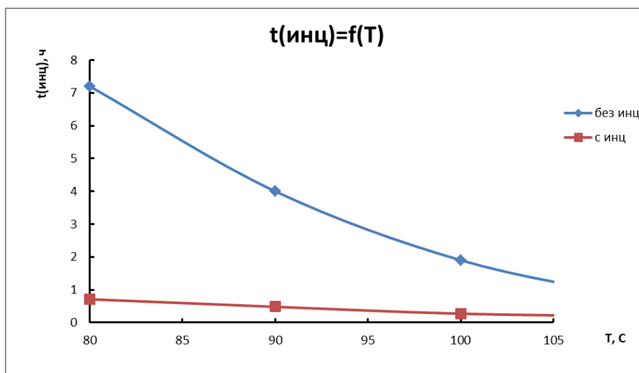
Рисунок 3.6 – Время инициации с инициатором H_2O_2 и без него при температурах 80-100 ^{\circ}\text{C} при низком расходе воздуха
