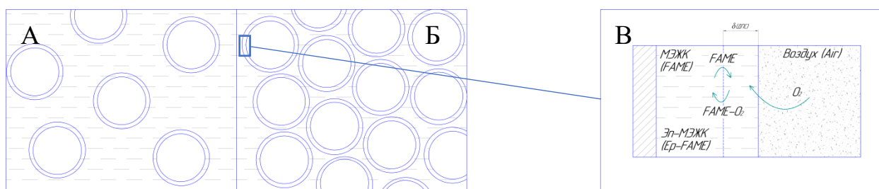
Рисунок 3.30 – Схематическое изображение: А – газосодержание \phi_r < 0,6 ; Б – газосодержание \phi_r > 0,6 ; В – процессы, протекающие на границе раздела фаз и в пограничном слое
