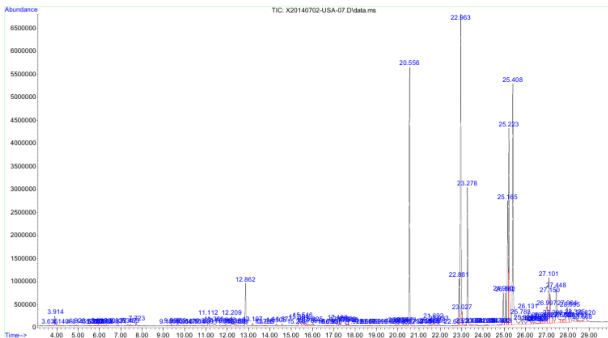
Рисунок 3.18 – Типичная хроматограмма конечной реакционной массы
