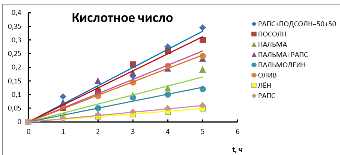
Рисунок 3.10 Б – График зависимости КЧ от времени проведения процесса
