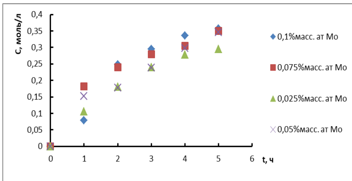
Рисунок 3.1 – Накопление в реакционной массе эпоксидных соединений в зависимости от концентрации катализатора на МЭЖК подсолнечного масла
