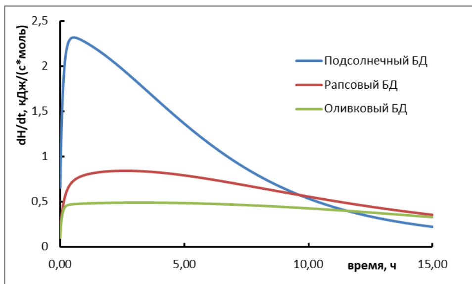
Рисунок 3.28 – Дифференциальное тепловыделение в процессе эпоксидирования биодизеля, полученного из подсолнечного, оливкового и рапсового масла
