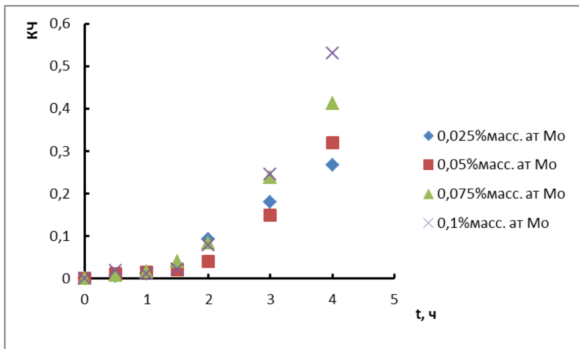
Рисунок 3.2 – Изменение кислотного числа реакционной массы при окислении МЭЖК подсолнечного масла
