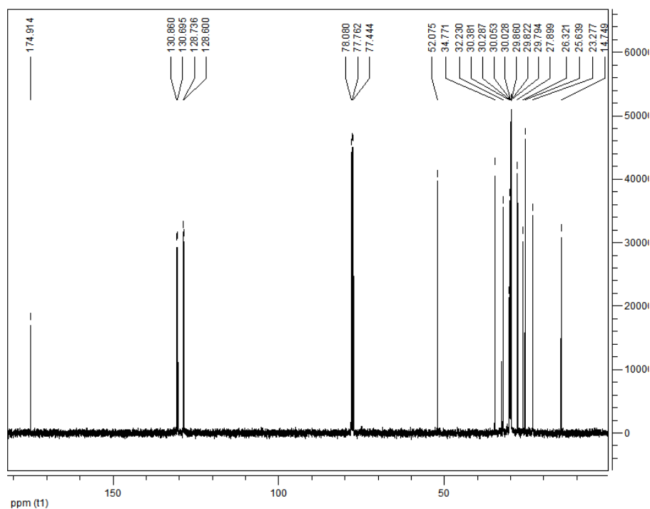
Рисунок 3.23 – ЯМР ^{13}\text{C} -спектр МЭЖК
