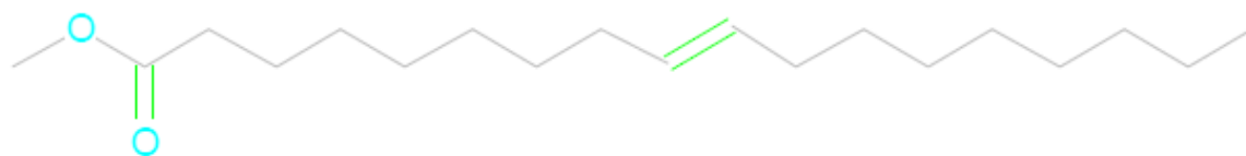
Масс-спектр метилолеата (C 18/1 )
