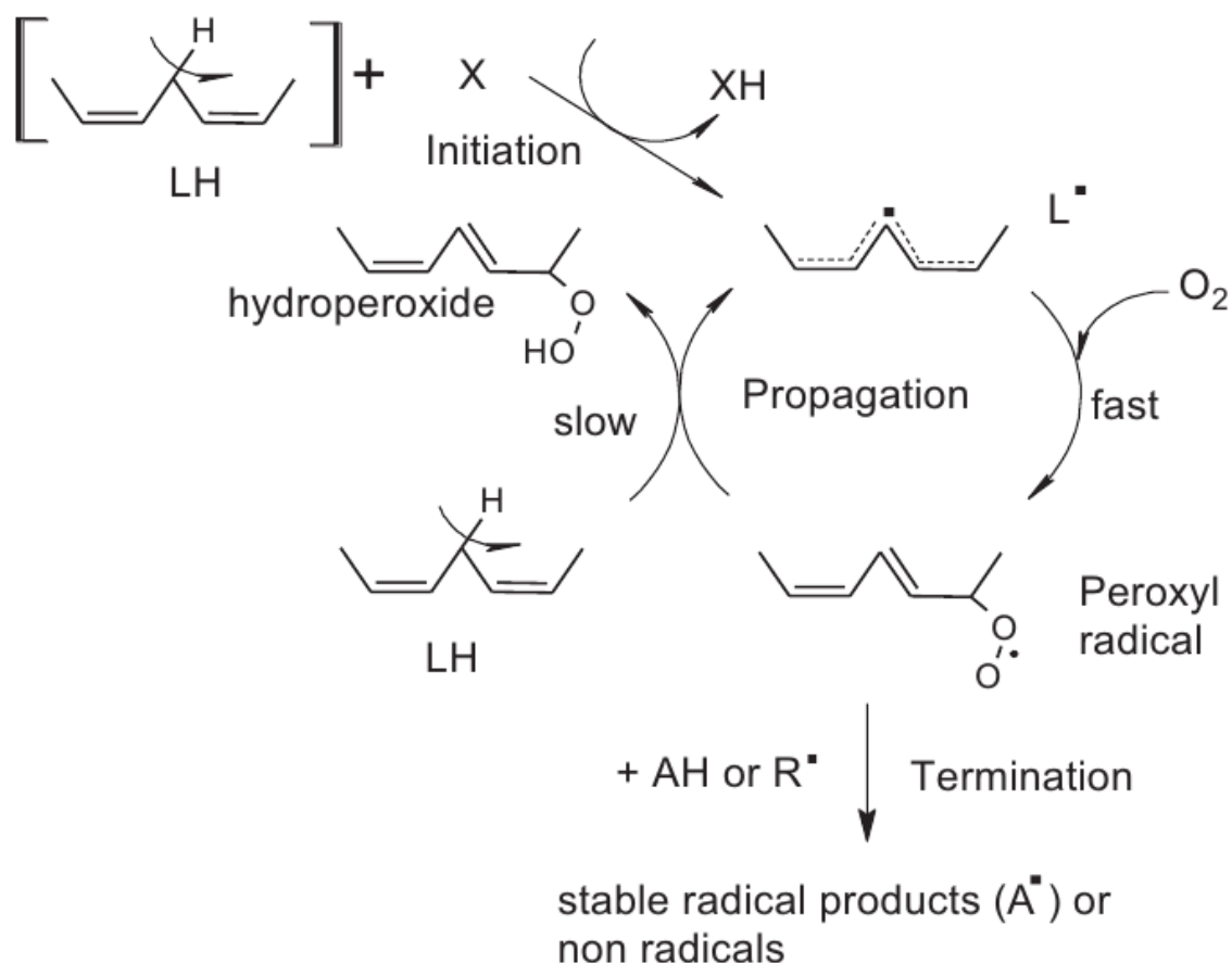
Рисунок 1.1 – Механизм образования ГП[8]
