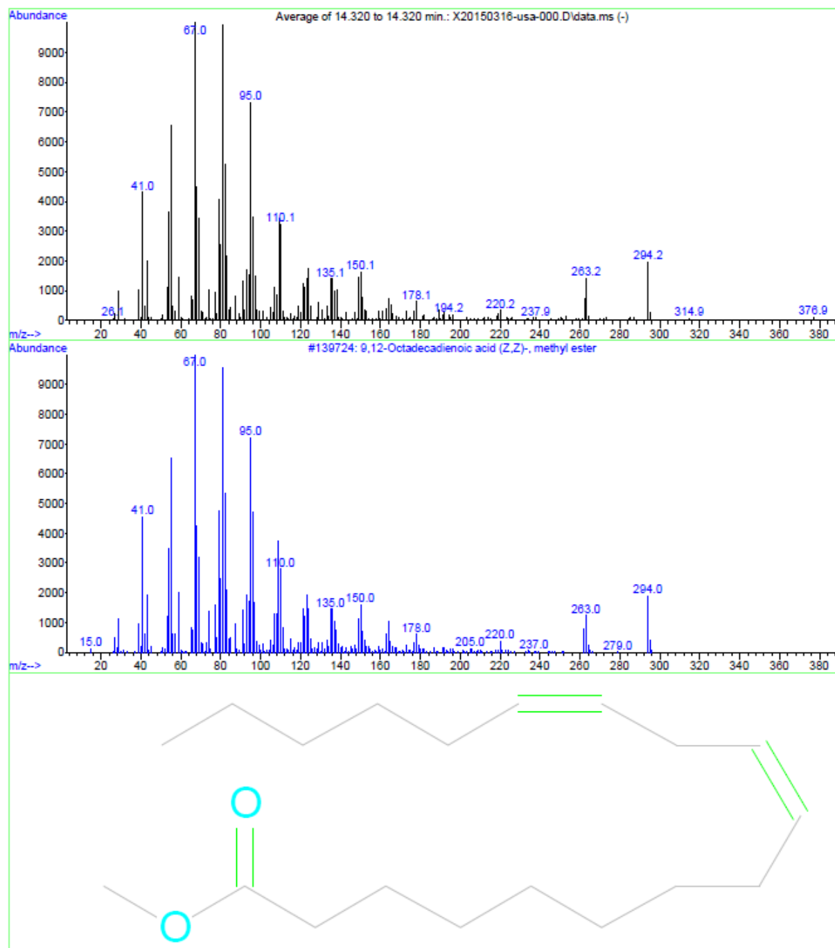
Масс-спектр метиллинолята (C 18/2 )
