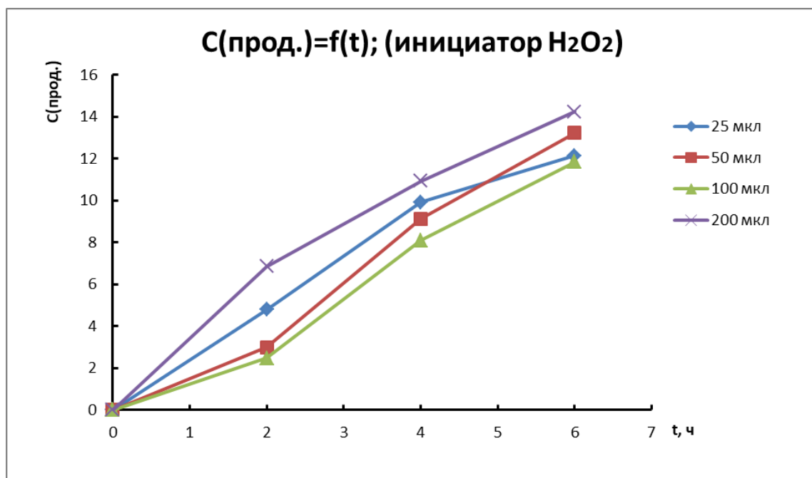
Рисунок 3.4 – Образование эпоксидов при низком расходе с инициатором
