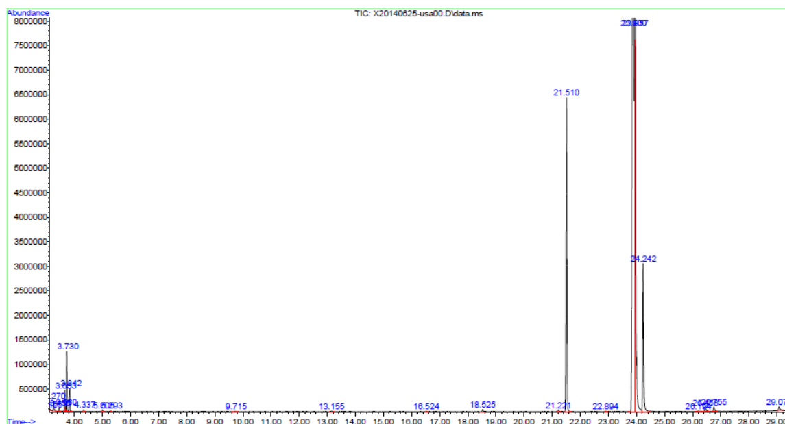
Рисунок 3.17 – Типичная хроматограмма исходного БД
