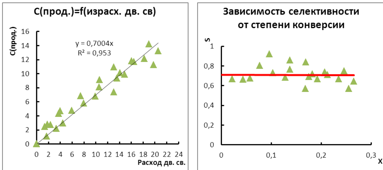
Рисунок 3.12 – Селективность процесса при низком расходе воздуха
