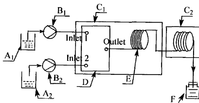
Рисунок 1.2 – Технологическая схема микроструктурированного реакторов, A1, A2-резервуар для сырья B1, B2-насосы; стекло микро-смеситель C1 и C2 находятся в инкубаторе; (T-micromixer, Microglass, Германия); E-микроканальный реактор; F-бутылка сбора продукта (с ледяной водой)[56]
