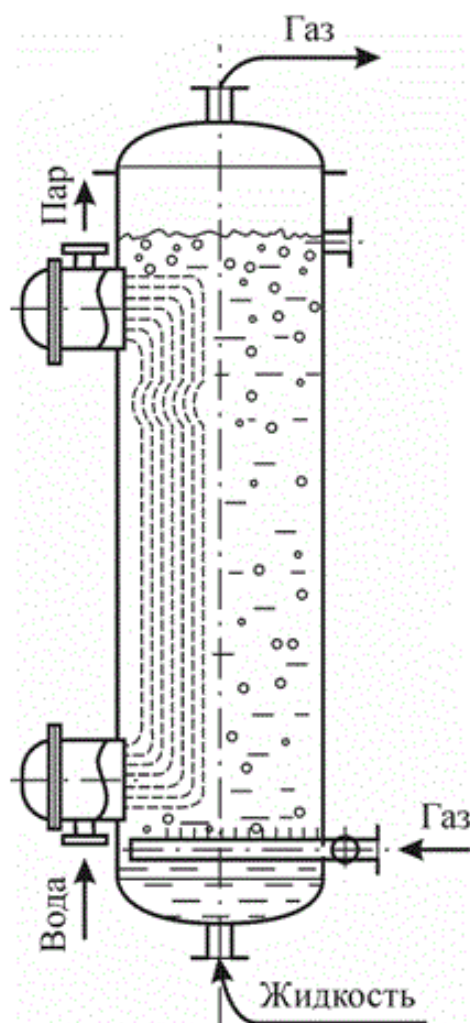
Рисунок 3.34 – Эскиз аппарата барботажного типа с внутренними теплообменными устройствами
