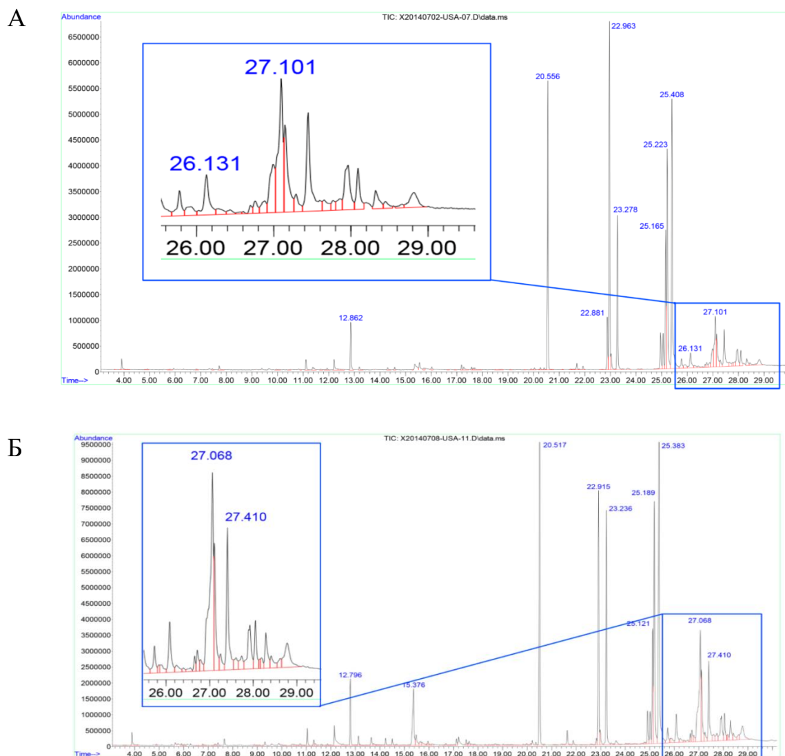
Рисунок 3.16 – Хроматограммы продуктов окисления МЭЖК при их \approx 70\% конверсии. Реакционная масса после окисления в пузырьковом режиме барботажа (А) и в режиме динамической ячеистой пены (Б). Времена удерживания компонентов: менее 20 мин – продукты деструктивного окисления непредельных компонентов МЭЖК; C_{16/0} – 20.5 мин, C_{18/0+1} – 22.9 мин; C_{18/2} – 23.3 мин; эпоксицированные МЭЖК – 24.9-25.5 мин; свыше 26 мин – продукты уплотнения
