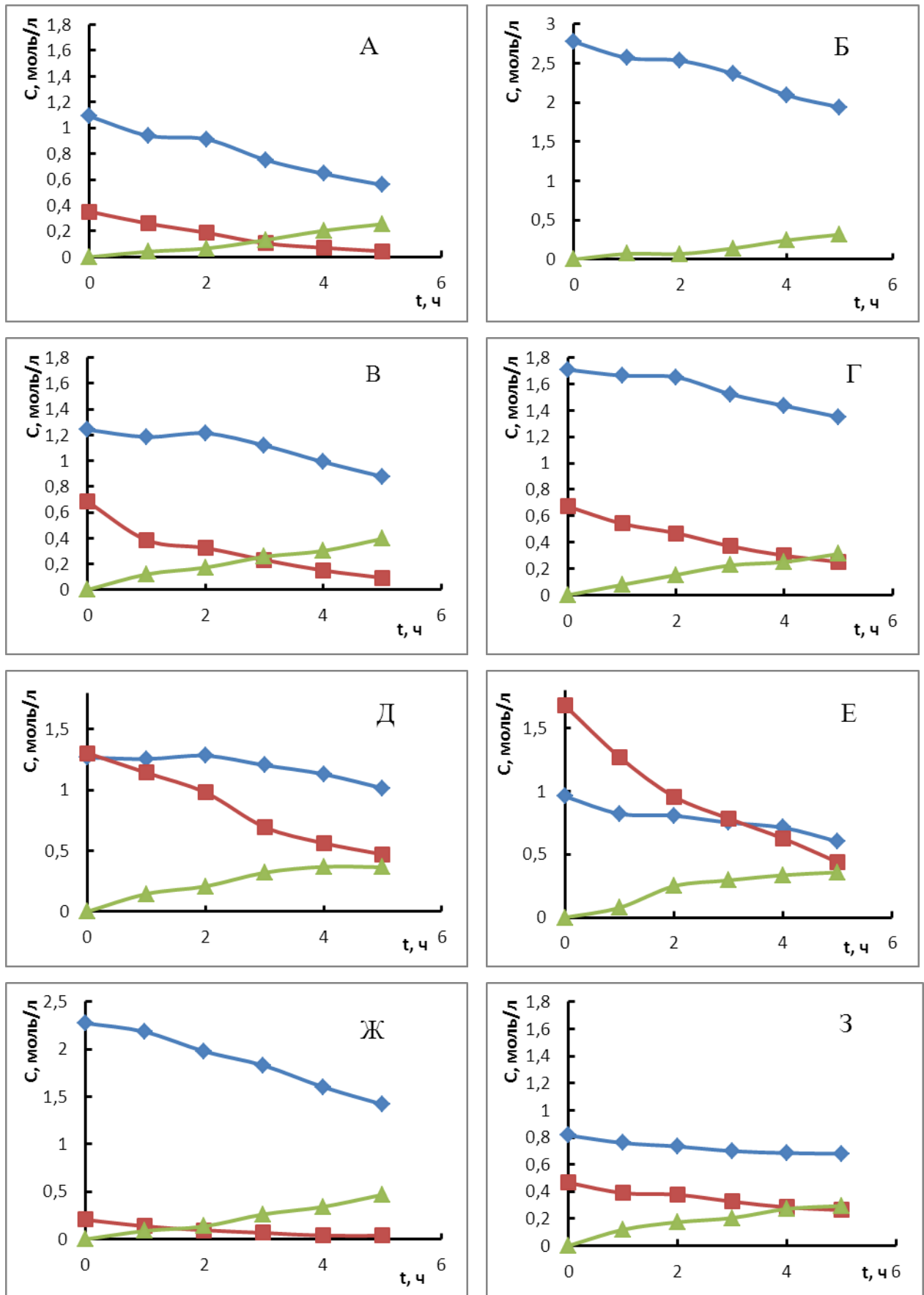
Рисунок 3.7 – Кинетические зависимости эпексидирования МЭЖК, полученных из: А – пальмового масла; Б – пальмолеина; В – смеси
