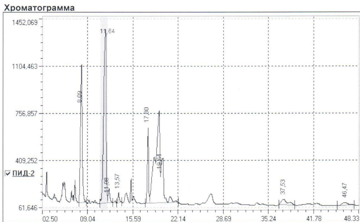
Рисунок 2.3 – Хроматограмма конечной реакционной массы
