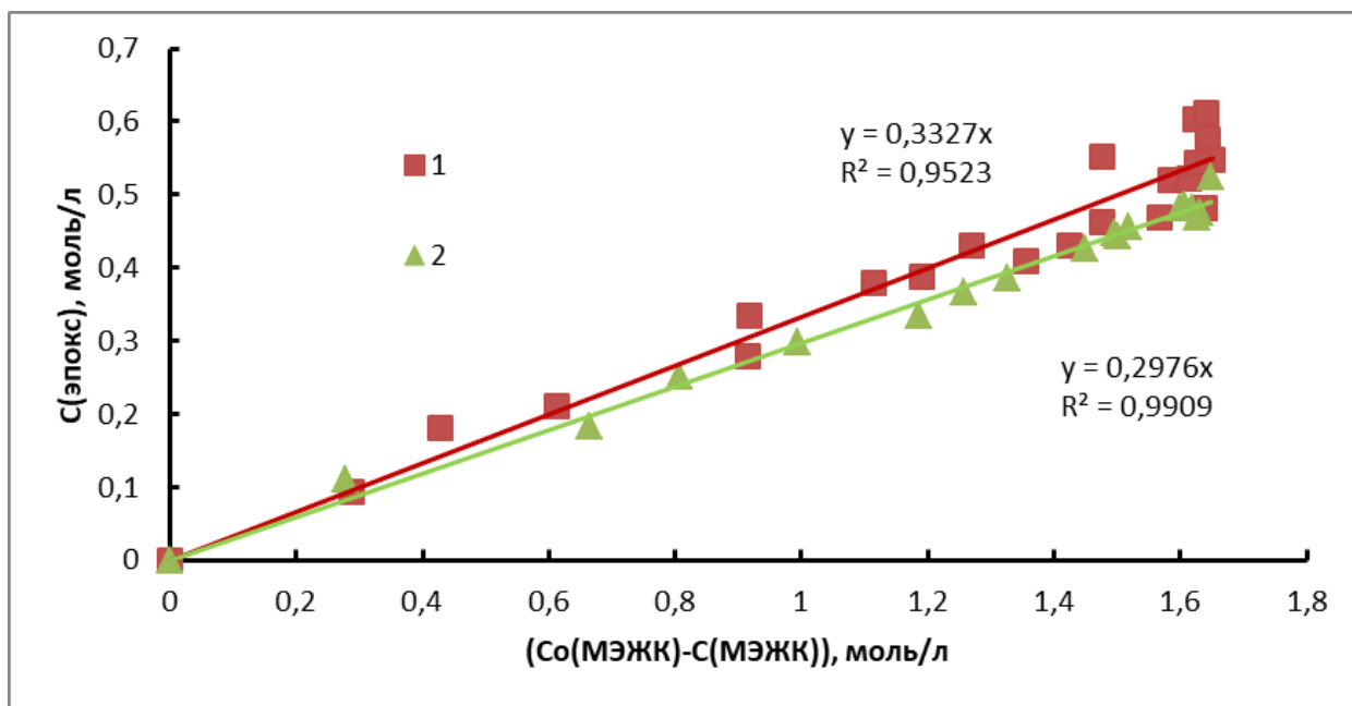
Рисунок 3.14 – Зависимости концентраций эпоксидных соединений от конверсии двойных связей МЭЖК в реакции окисления в разных режимах барботажа при T = 110^{\circ}\text{C} . Кривые: 1 – колонна с насадкой (подача воздуха 10 мл/с), 2 – колонна в режиме динамической ячеистой пены (подача воздуха 30 мл/с)
