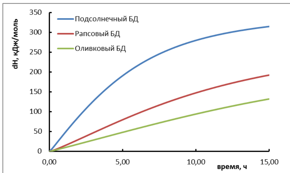
Рисунок 3.29 – Интегральное тепловыделение в процессе эпексидирования биодизеля, полученного из подсолнечного, оливкового и рапсового масла
