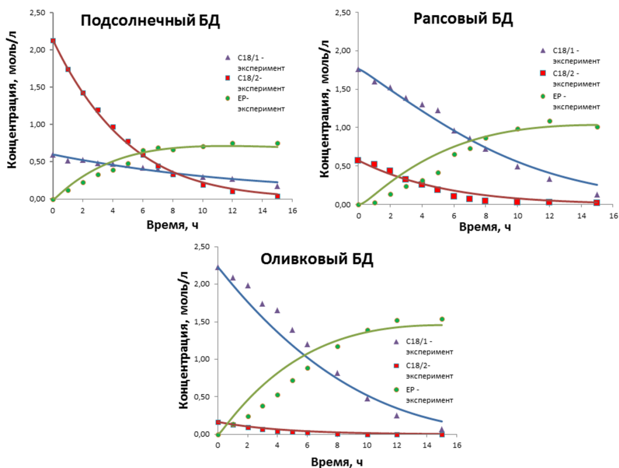
Рисунок 3.26 – Экспериментальные точки и расчетные кривые изменения концентрации исходных веществ и целевого продукта во времени для разных видов сырья
