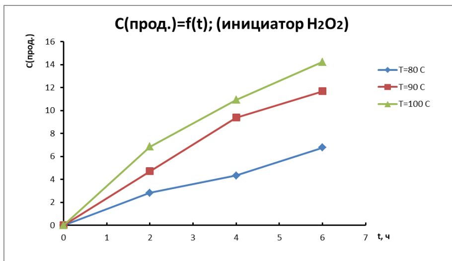
Рисунок 3.5 – Образование эпоксидов при низком расходе воздуха с инициатором H_2O_2 при температурах 80-100 ^{\circ}\text{C}
