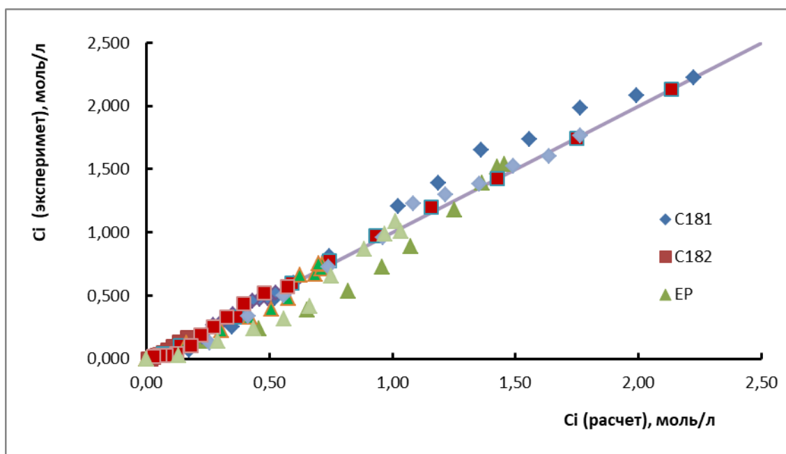
Рисунок 3.27 – Корреляция экспериментальных и расчетных значений концентраций компонентов биодизеля
