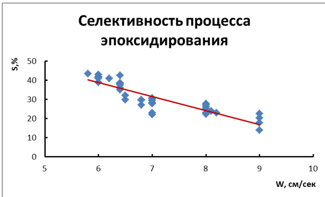
Рисунок 3.16.1 – Зависимость селективность образования эпоксидных соединений от линейной скорости барботажа
