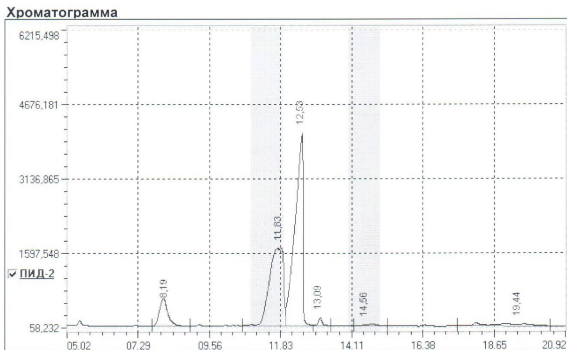
Рисунок 2.2 – Хроматограмма исходного БД
