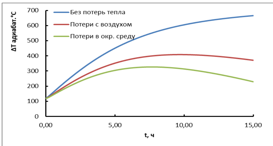
Рисунок 3.33 – Зависимость величины адиабатического разогрева от времени синтеза
