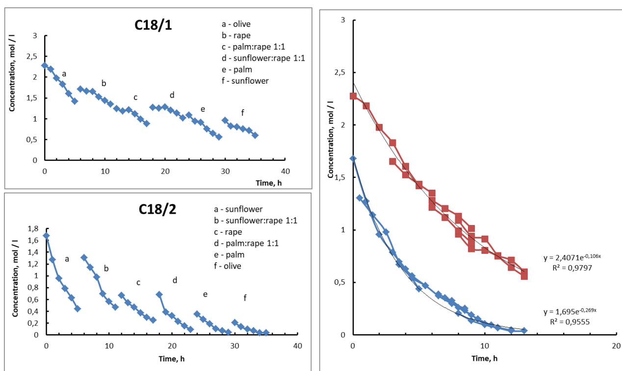
Рисунок 3.9 Б – зависимость концентрации исходных компонентов сырья от времени проведения синтеза
