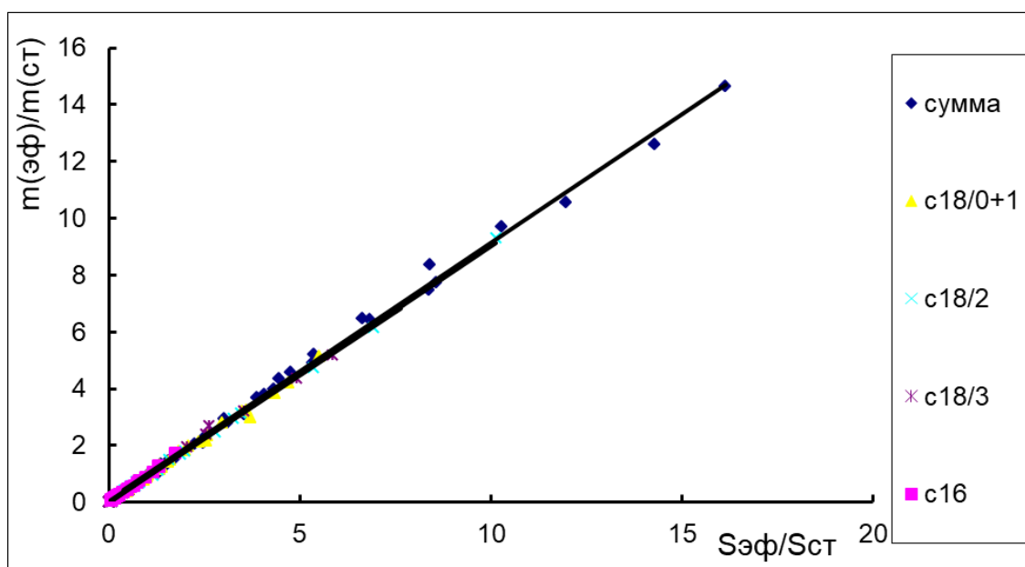
Рисунок 2.4 – Калибровочная кривая МЭЖК
