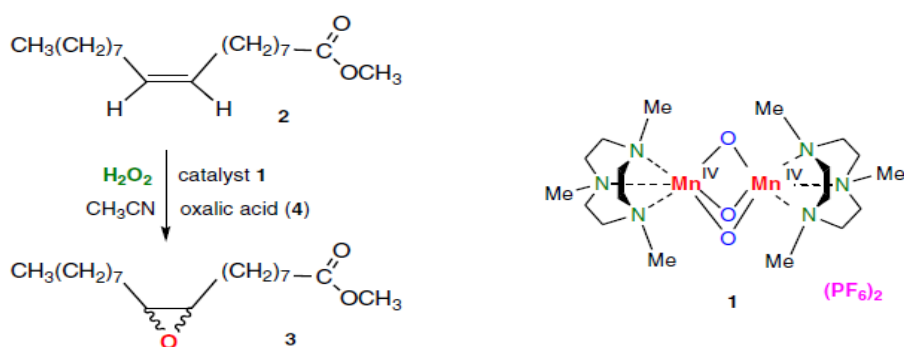
Рисунок. 1.3 – Схема реакции и строение используемого комплекса[64]
