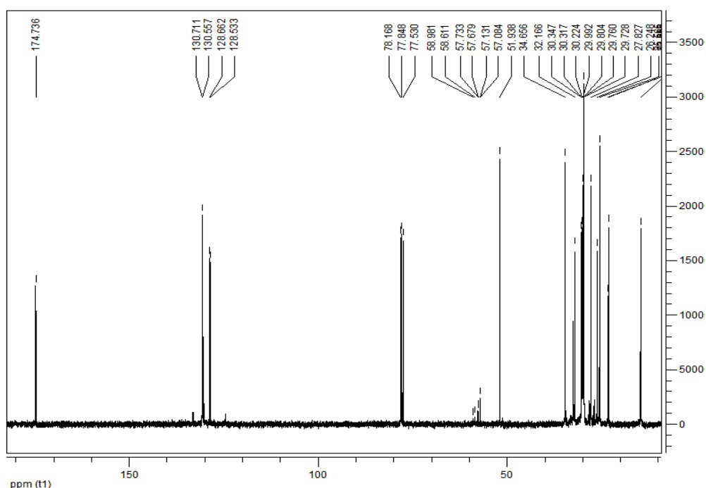
Рисунок 3.25 – ЯМР ^{13}\text{C} -спектр ЭМЭЖК
