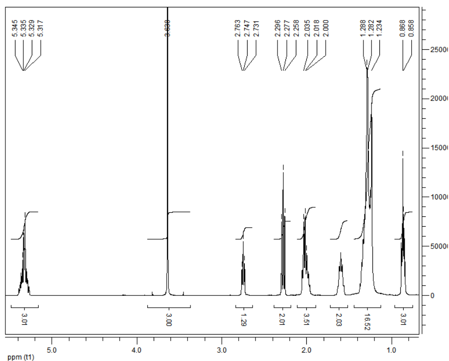
Рисунок 3.22 – ЯМР ^1\text{H} -спектр МЭЖК
