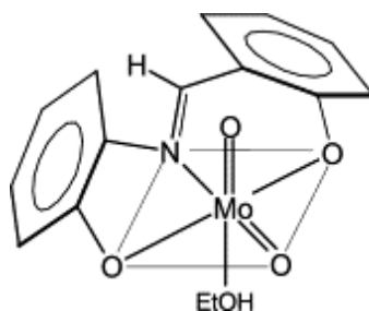
Рисунок 1.4 – структура комплекса [\text{Mo}(\text{O})_2(\text{SAP})(\text{EtOH})] [65]
