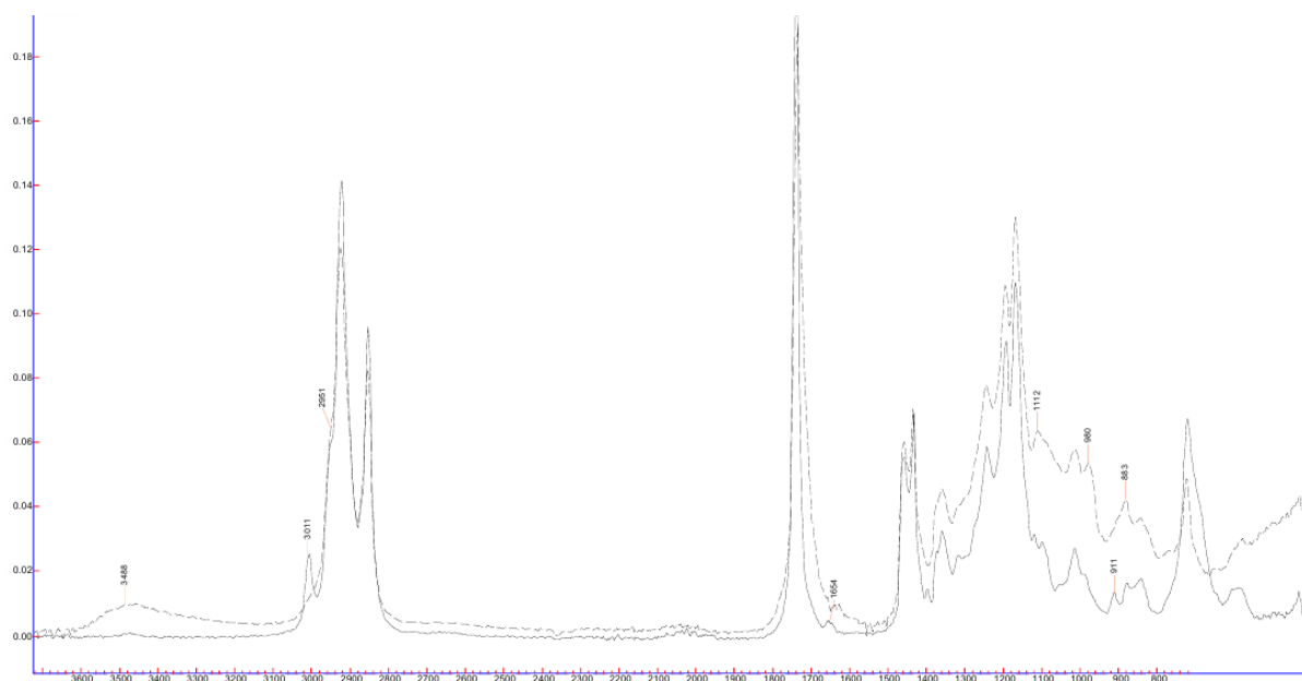
Рисунок 3.21 – ИК-спектр реакционной массы после проведения процесса
