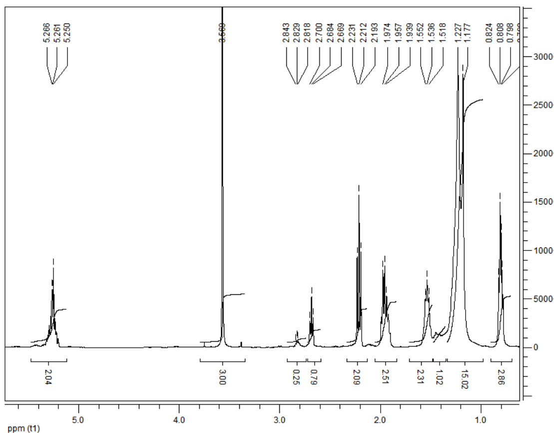
Рисунок 3.24 – ЯМР ^1\text{H} -спектр ЭМЭЖК
