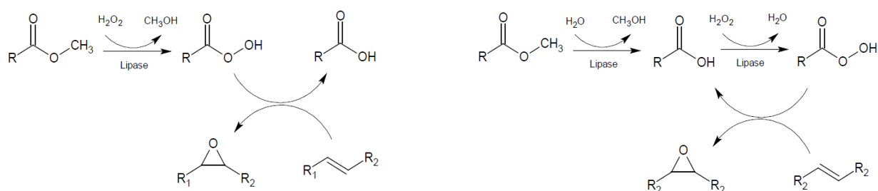
Рисунок 1.6 – Реакции, протекающие при эпоксидировании МЭЖК, катализируемом ферментами[66]
