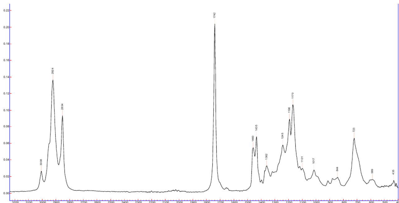
Рисунок 3.20 – ИК-спектр МЭЖК
