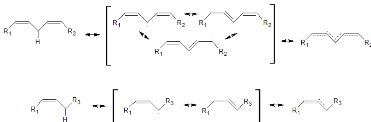
Рисунок 3.10 А – Стабильность радикалов C_{18/2} и C_{18/1} .
