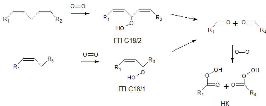
Рисунок 3.9 А – Схема окисления
