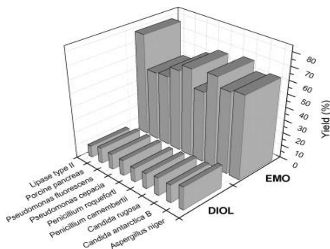
Рисунок 1.7 – Выходы эпоксидированных метиловых эфиров и диолов
