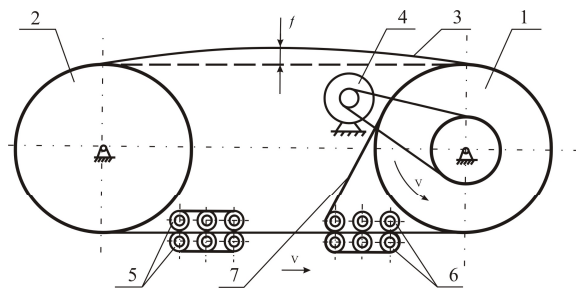
Рис. 2. Компоновочная схема механизма резания горизонтального ЛПС на основе длинных контактов трения относительного покоя, и "слабонатянутой" ЛП: 1, 2) ведущий и ведомый шкивы, 3) ЛП, 4) электродвигатель привода, 5, 6) тормозное и приводное направляющие устройства, 7) промежуточный гибкий тяговый рабочий орган, f — стрела прогиба от перераспределения усилия натяжения в соответствии с соотношением Ж. Понселе
