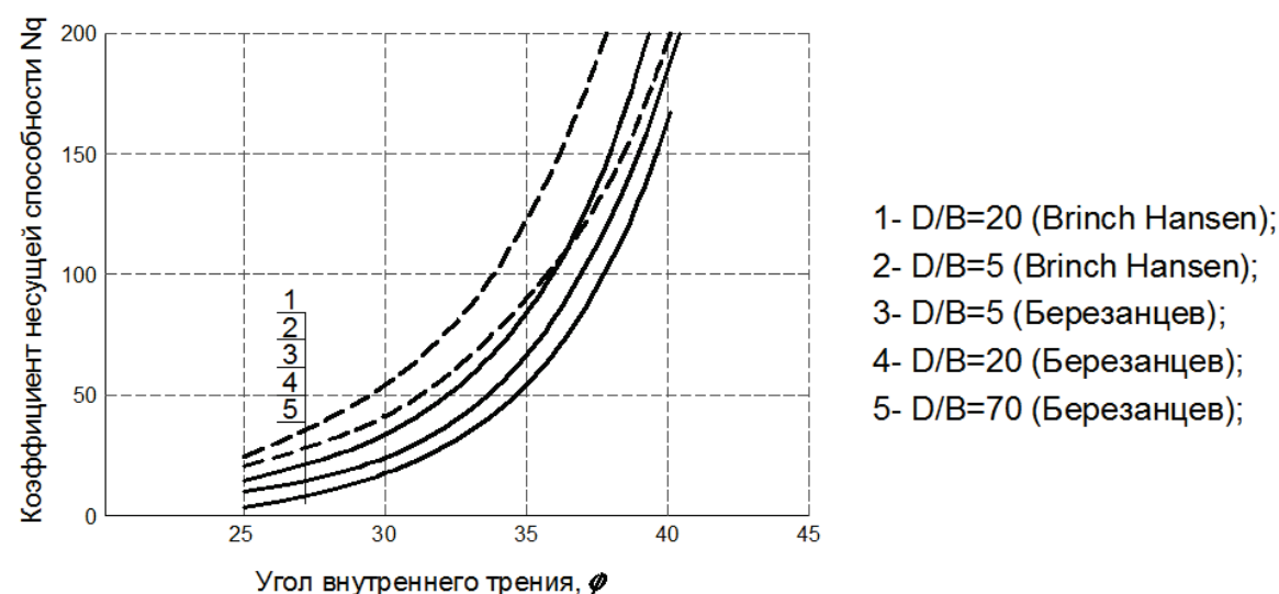
Рис. 10. Диаграммы зависимости коэффициента несущей способности от соотношения длины сваи к ее диаметру (по В.Г. Березанцеву и Brinch Hansen)
