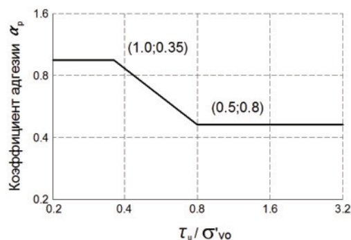
Рис. 8. Зависимость коэффициента адгезии от уровня переуплотнения грунта
