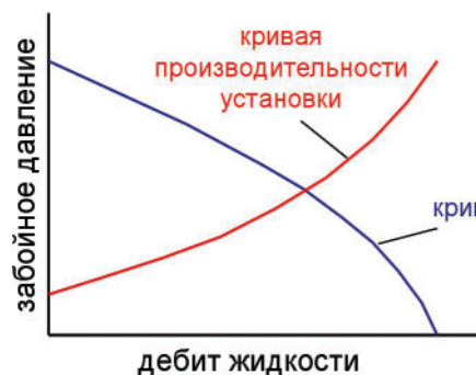
Рис. 2. Графические зависимости погружной установки
