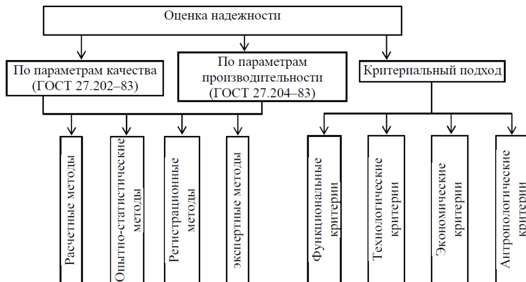
Рисунок 1 – Методы оценки надежности технических объектов, технических систем и технологических систем
