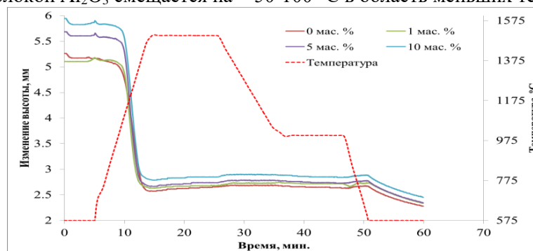
Рисунок 1 - Динамика линейной усадки PSZ-керамики армированной 1 - 10 мас. % нановолокнами \text{Al}_2\text{O}_3
