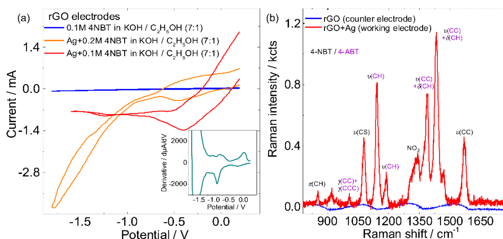
Рисунок 2 – (a) – Вольтамперограммы разных концентраций 4-NBT до и после осаждения серебра на рабочий электрод, вставка – вольтамперограмма (производная) образца, приготовленного для SERS, (b) – детектирование 4-NBT с помощью SERS
