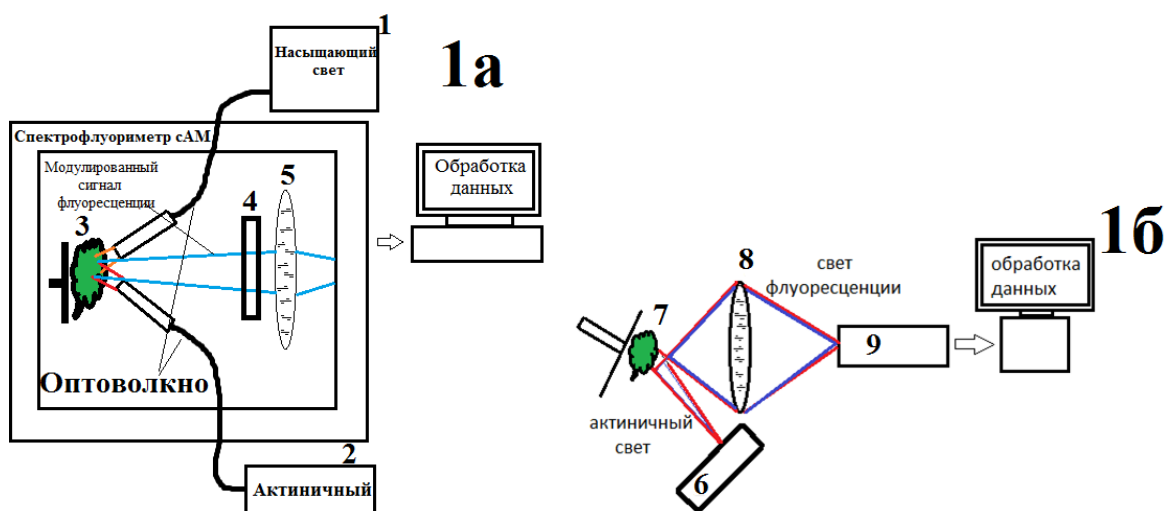
Рисунок 1 – Схема экспериментальных установок измерения параметров флуоресценции хлорофилла методом амплитудной модуляции (1а) и прямым способом (1б) – источник насыщающего излучения; 2) – источник актиночного света; 3) – образец растения; 4) – фильтр монохроматора; 5) – собирающая линза 6) источник света; 7) исследуемый образец; 8) собирающая линза; 9) монохроматор
