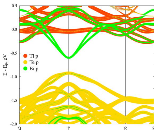
Рисунок 2 – Зонный спектр тонкой нестехиометрической пленки [\text{TlBiTe}_2]/[\text{TlGdTe}_2] , рассчитанный для антиферромагнитной неколлинеарной магнитной конфигурации вдоль симметричных направлений поверхностной зоны Бриллюэна
