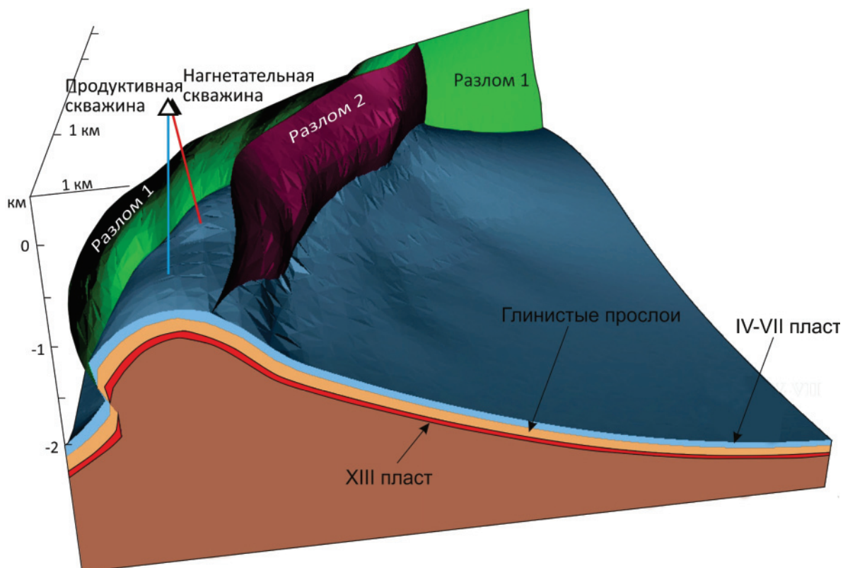
Рис. 3. Трехмерная геологическая модель Ханкальского месторождения
