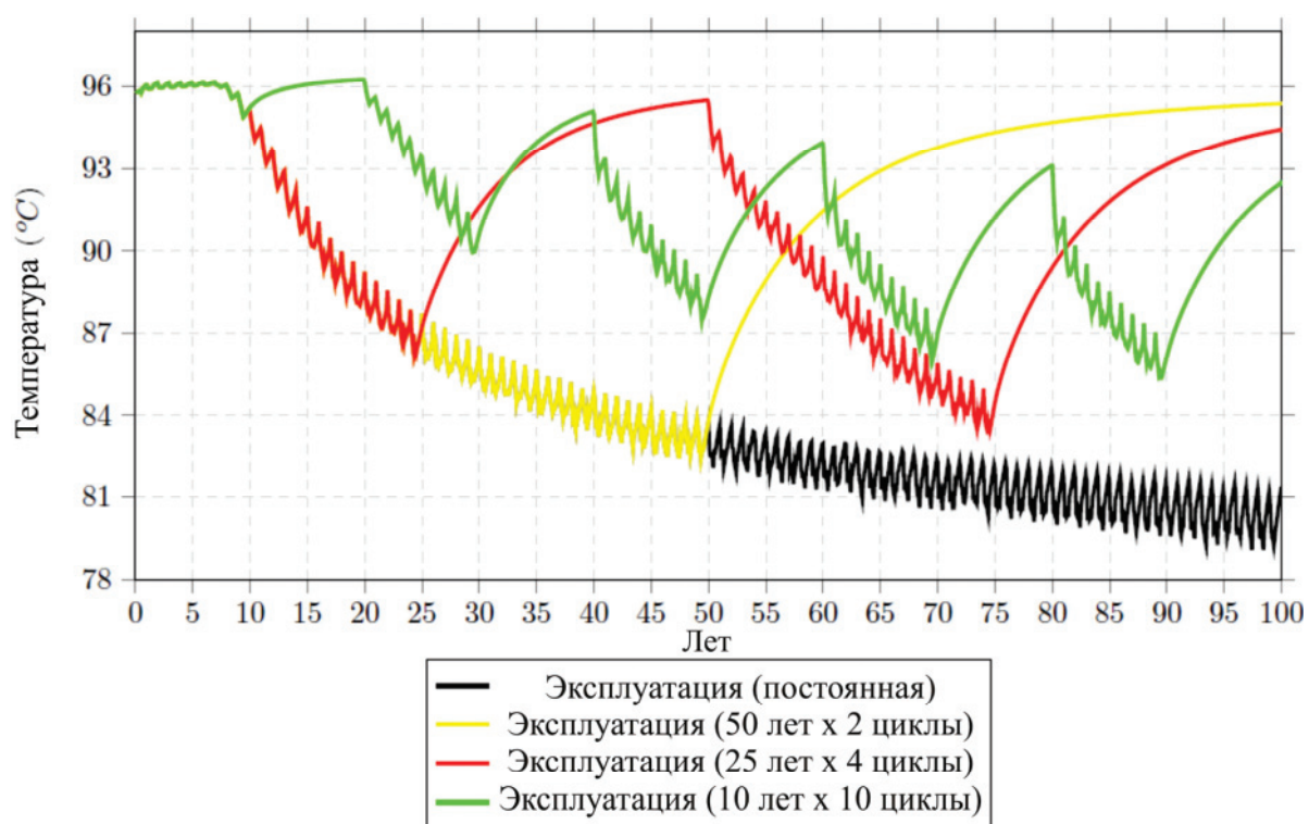
Рис. 8. Результаты моделирования: изменение температуры в эксплуатационной скважине для различных сценариев эксплуатации Fig. 8. Modeling results: production well temperature change in case of different exploitation scenarios
