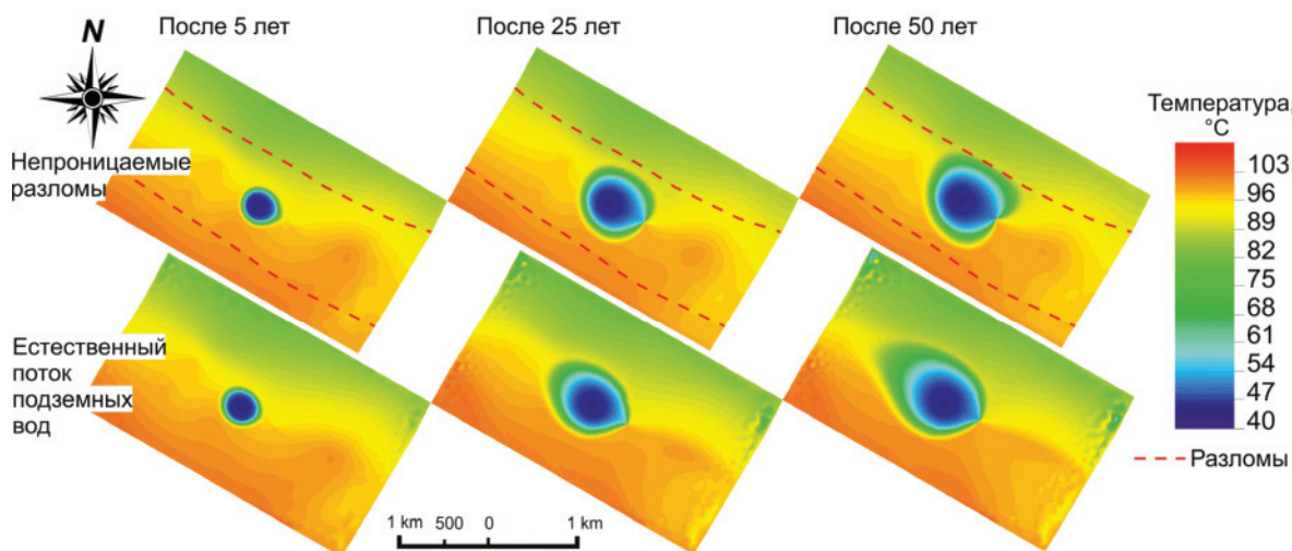
Рис. 7. Результаты моделирования: изменение температуры в XIII пласте
