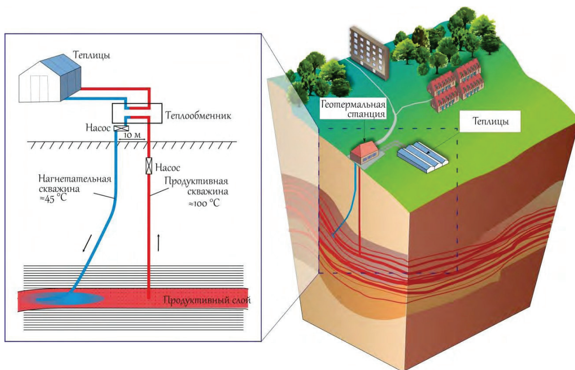
Рис. 4. «Дублетная» циркуляционная система Ханкальского месторождения
