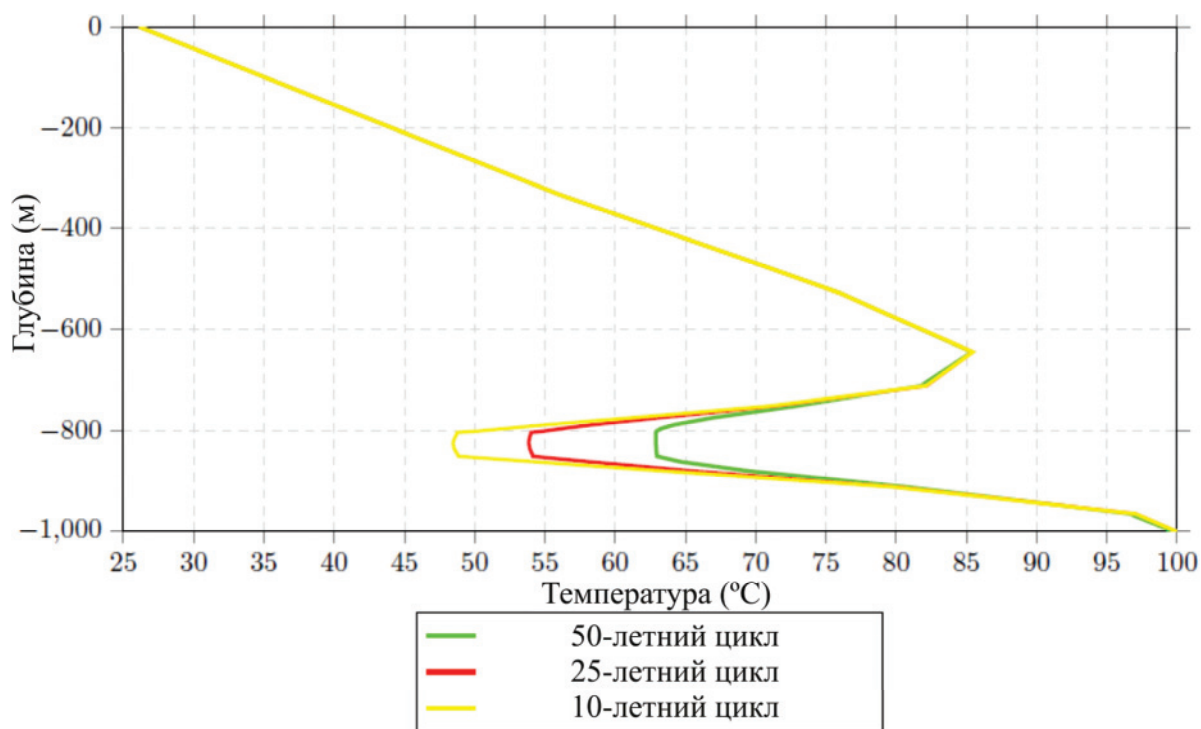
Рис. 9. Температурный профиль на продуктивной скважине после 100 лет эксплуатации Fig. 9. Temperature section at the production well after 100 years of exploitation
