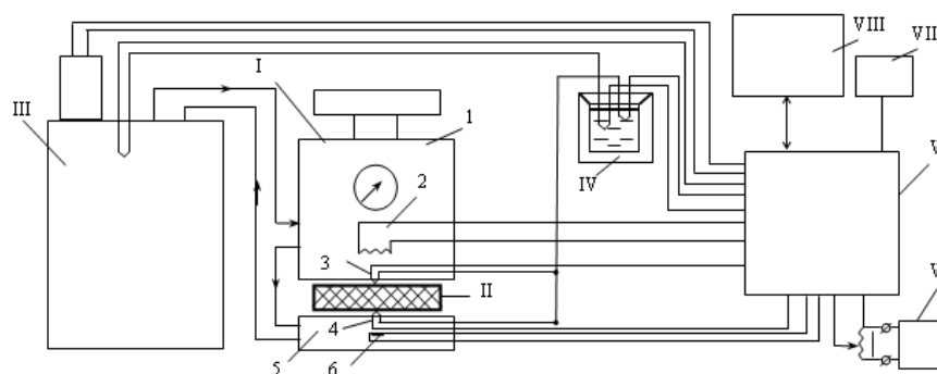
Рисунок 1 – Структурная схема автоматизированной системы: I – измерительная ячейка; II – образец испытуемый; III – термостат; IV – сосуд Дьюара; V – блок управления и измерений; VI – лабораторный автотрансформатор; VII – стабилизированный источник постоянного тока; VIII – стабилизатор; 1 – механизм перемещения; 2 – электрический нагреватель; 3, 4 – термопары; 5 – холодильник; 6 – датчик теплового потока
