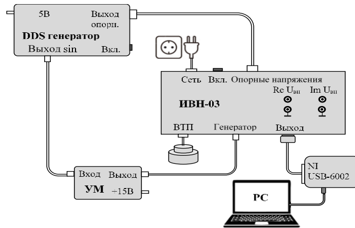
Рисунок 3 – Схема электрических соединений системы вихретокового контроля СВК-03
