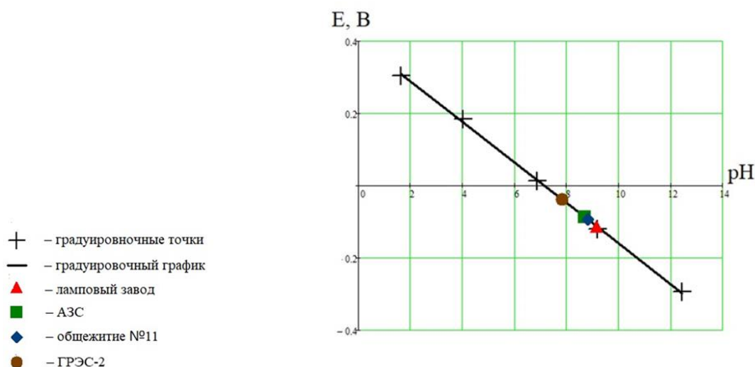
Рисунок – График зависимости ЭДС электродной системы от кислотности среды E(\text{pH})
