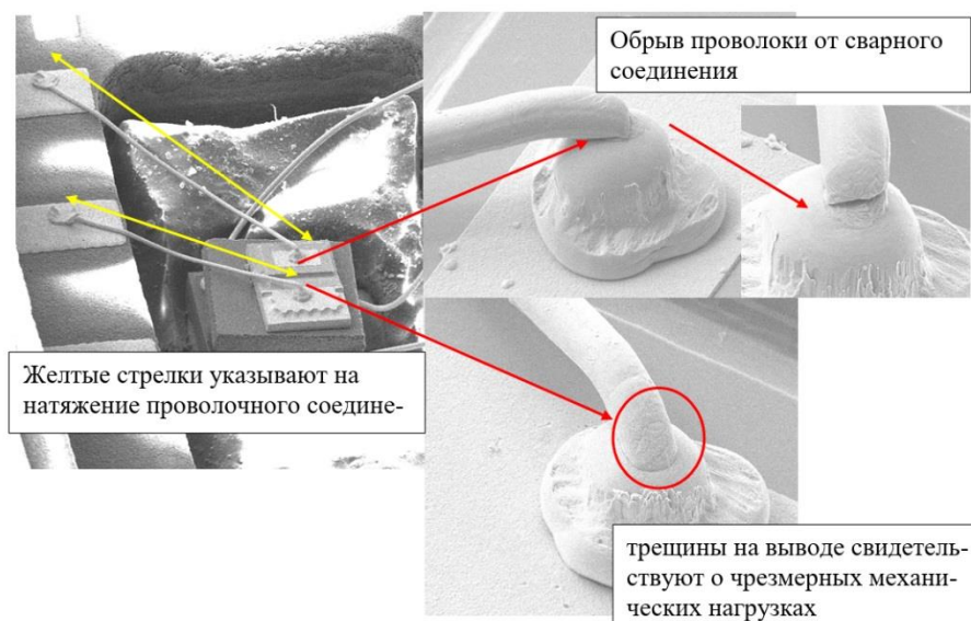
Рисунок 2 – Натяжение внутренних выводов, обрыв золотой проволоки от сварного соединения
