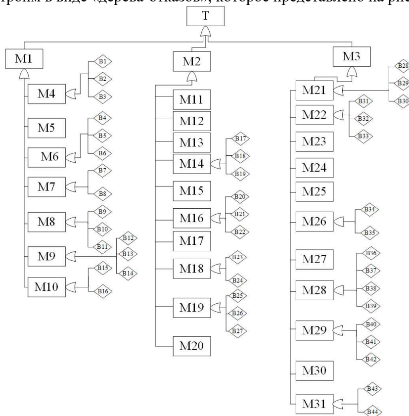
Рисунок 2 – Вариационная модель взрыва на трансформаторной подстанции
