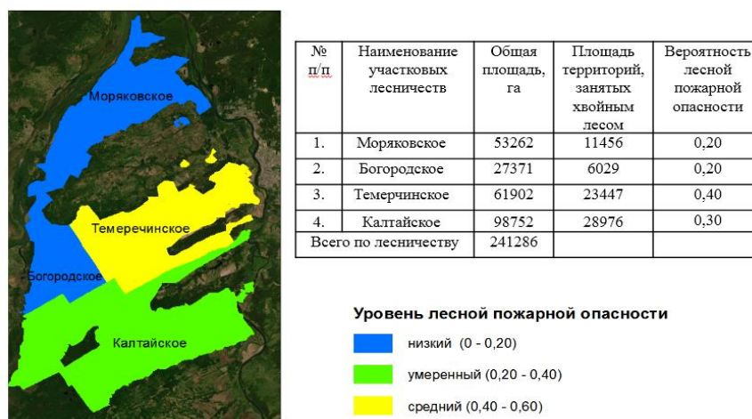
Рисунок 6 – Схема лесной пожарной опасности территории Тимирязевского по лесорастительным условиям
