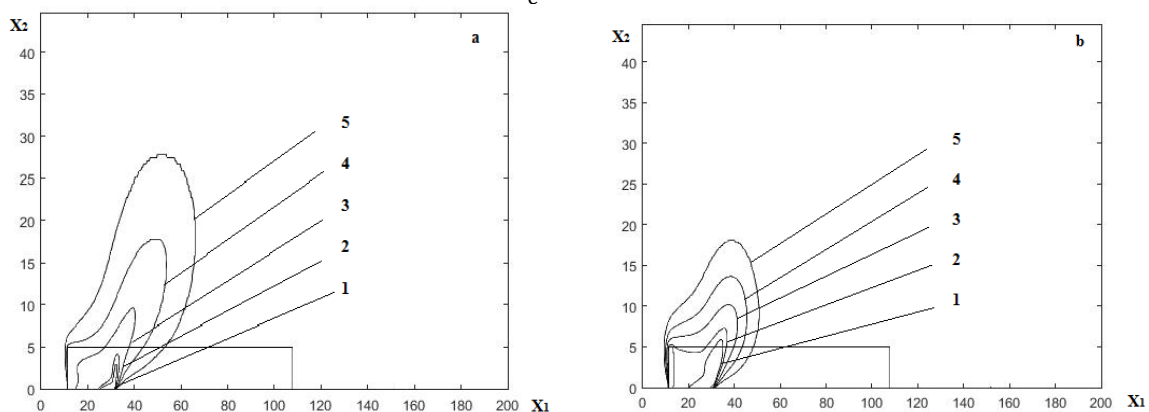
Рисунок 2 – Распространение лесного пожара при скорости ветра 6 м/с в момент времени а)10, б)15 сек
