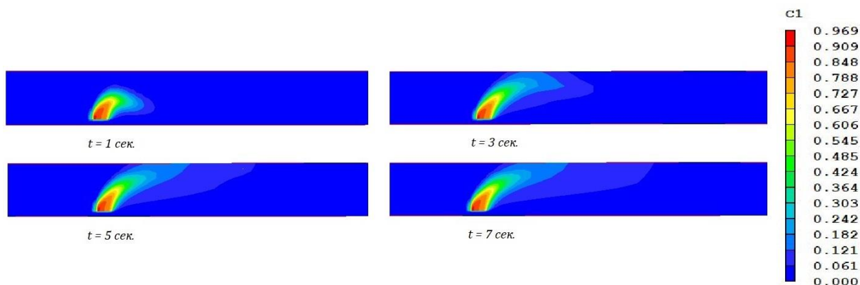
Рисунок 3 – Распределение концентрации C_1 в разные моменты времени
