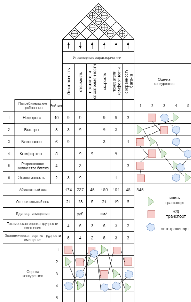
Рисунок 3 – Домик качества
