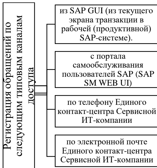
Рисунок 2 – Каналы доступа
