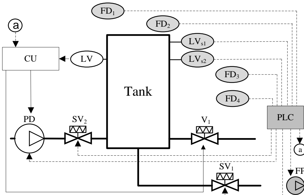
Рисунок 1 – Подсистема подачи горючих материалов, (белым цветом представлены элементы, связанные с основным выполнением технологии, серым – связанные с обеспечением безопасностью)
