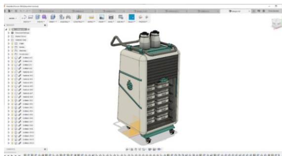
Рисунок 4 – Параметрическое моделирование
