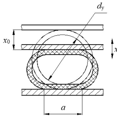
Рисунок 1 – Схема поджатого рукава
