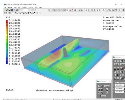
Рисунок 9 – Окно VR-Viewer, запущенное после завершения работы EARTH
