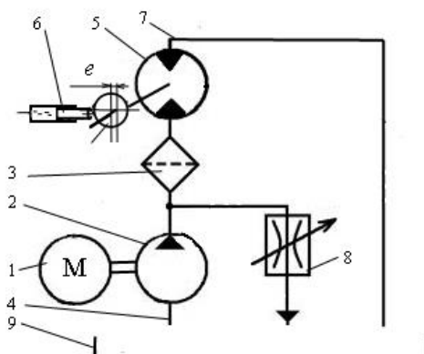
Рисунок 2 – Принципиальная схема гидропривода
