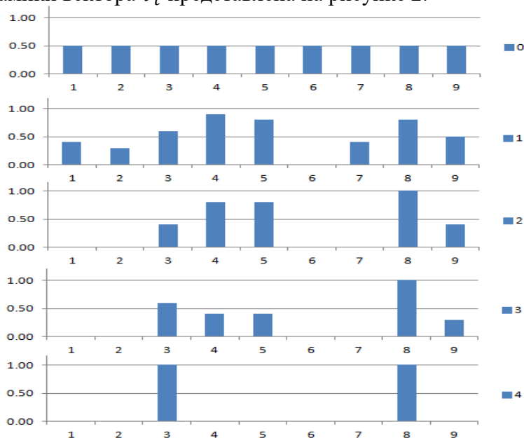
Рисунок 2 – Динамика вероятностного вектора \hat{\mathbf{v}}_t
