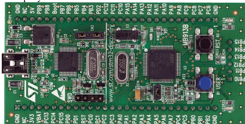
Рисунок 1 – Отладочная плата STM32VLDISCOVERY
