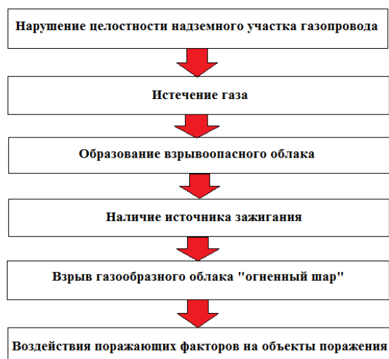
Рисунок 1 – Сценарий развития аварии на магистральном газопроводе
