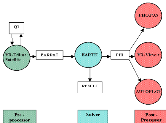
Рисунок 1 – Взаимодействие модулей PHOENICS
