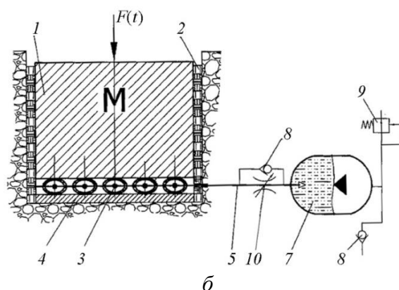
Рисунок 2 – Конструктивная схема виброизолирующего фундамента с гидроневматическим амортизатором и: а – струйным элементом; б – регулируемым дросселем
