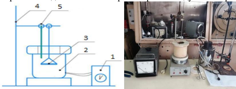
Рисунок 1 – Схема установки для проведения экспериментов с образцами лесной подстилки 1 – автотрансформатор; 2 – тепловая камера; 3 – контейнер с образцом; 4 – штатив; 5 – термопара с прибором регистрации
