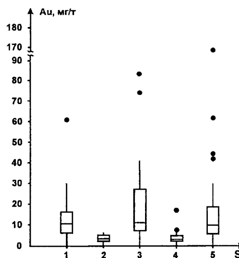
Рис. 2. Диаграмма распределения содержаний золота в зависимости от степени пластической деформации ультрамафитов.
