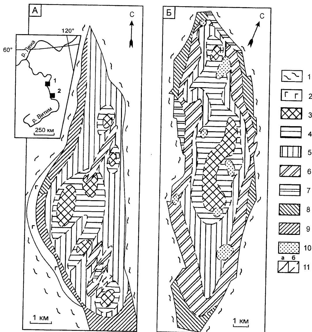
Рис. 1. Схемы динамометаморфической зональности Парамского (А) и Шаманского (Б) ультрамафитовых массивов. 1) кристаллические сланцы; 2) габбро; 3–9 – деформационные типы микроструктур оливина в дунитах и гарцбургитах: 3) протогранулярный, 4) мезогранулярный, 5) порфирокластовый, 6) порфиroleйстовый, 7) мозаично-лейстовый, 8) мозаичный, 9) мозаично-паркетовидный; 10) кляважированные ультрамафиты; 11) границы: а) геологические, б) петрографические. На врезке показано географическое положение ультрамафитовых массивов: 1) Парамский, 2) Шаманский
