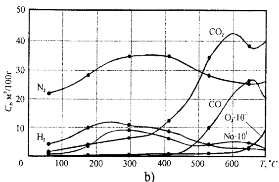
Рисунок. Зависимость концентрации десорбированных газов из УДП от температуры: а) Ni; б) Fe; в) CoO:Al 2 O 3 :ZnO:P 2 O 5 ; д) CoO:NiO:MnO 2 :CeO 2 . Темп нагрева 10 град/мин
