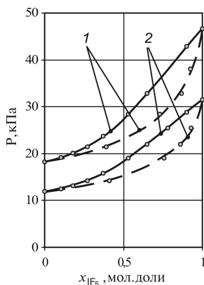
Рис. 3. Зависимость давления пара от состава раствора в системе \text{IF}_5\text{--BrF}_3 : 1) T=353,15\text{ K} ; 2) T=343,15\text{ K} ; — линия жидкости; ---- линия пара; —○— экспериментальные данные
