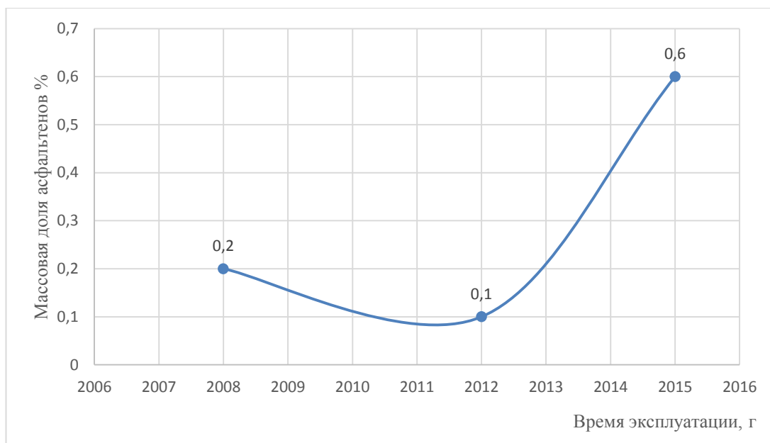
Рисунок 2.4 – Зависимость изменения массовой доли асфальтенов от времени эксплуатации скважины (Скважина № 123)
