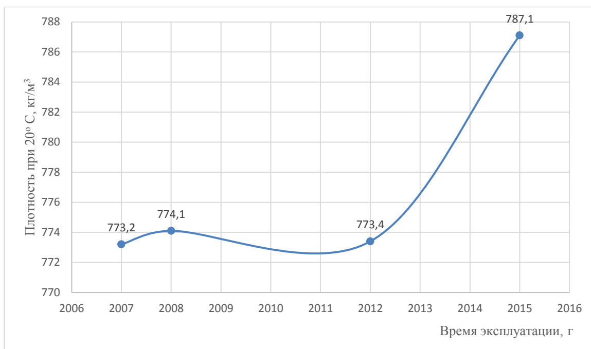
Рисунок 2.1 – Зависимость изменения плотности от времени эксплуатации скважины (Скважина № 123)
