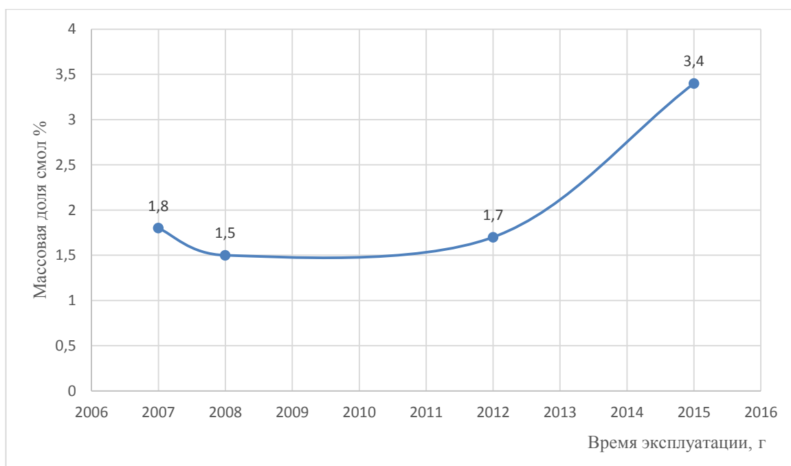
Рисунок 2.5 – Зависимость изменения массовой доли смол от времени эксплуатации скважины (Скважина № 123)
