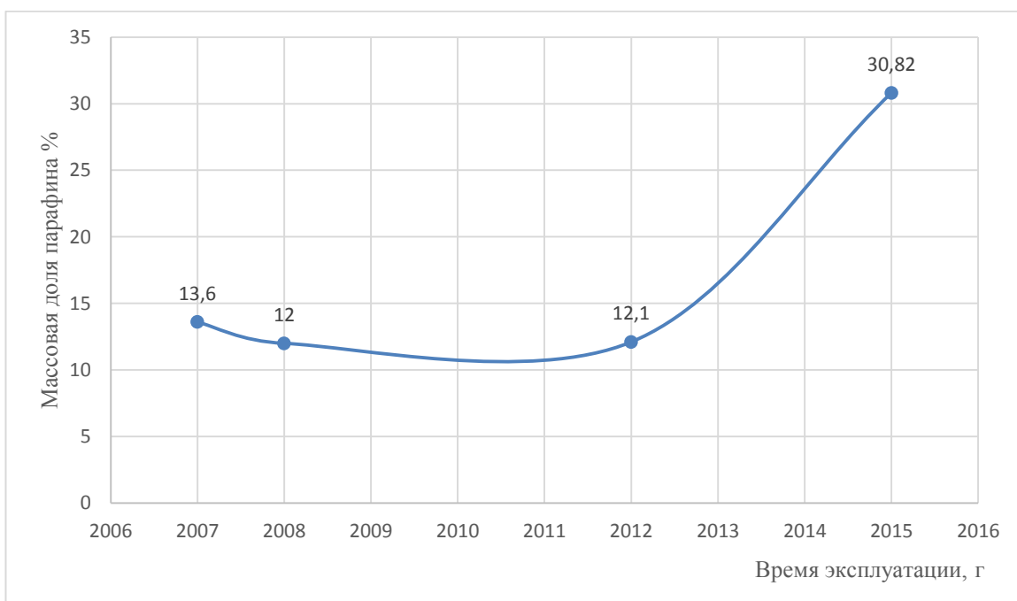
Рисунок 2.3 – Зависимость изменения массовой доли парафина от времени эксплуатации скважины (Скважина № 123)
