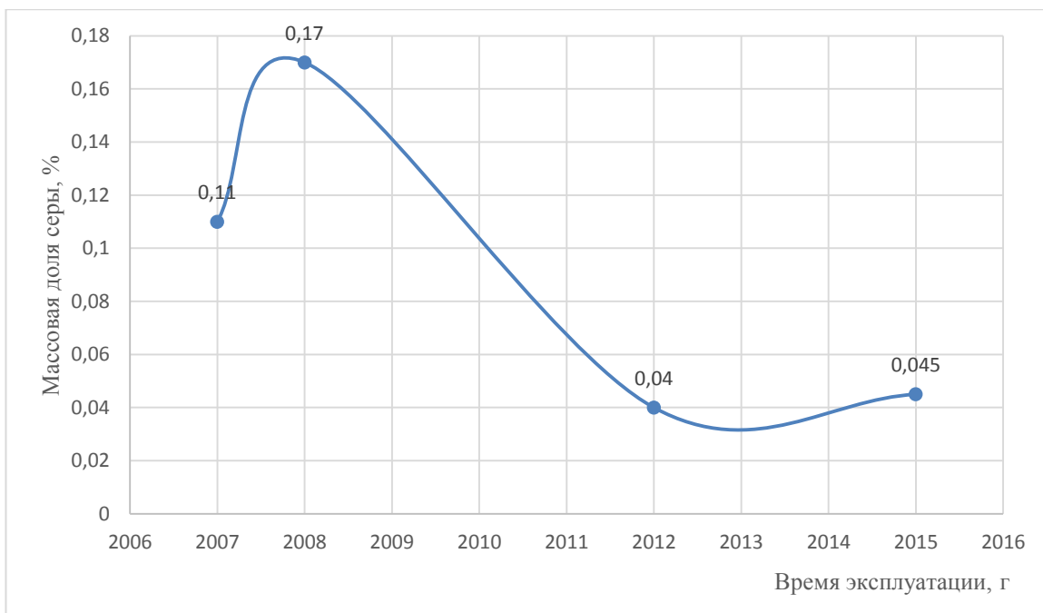
Рисунок 2.2 – Зависимость изменения массовой доли серы от времени эксплуатации скважины (Скважина № 123)
