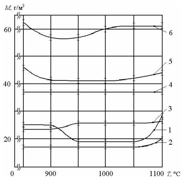
Рис. 1. Зависимость величины НКПР аэровзвеси бензойной кислоты от температуры инициирующего источника зажигания для частиц различных фракций, мкм: 1) 0...63; 2) 63...100; 3) 100...160; 4) 160...200; 5) 200...250; 6) 250...300
