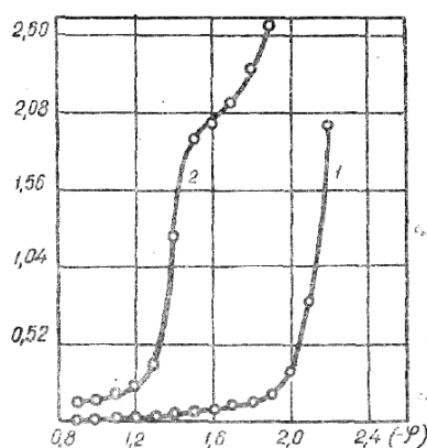
Рис. 1. Полярограмма ZrOCl_2 на фоне 0,1 м LiCl в метаноле. Кривая 1 — остаточный ток, 2 — 10^{-3} М ZrOCl_2
