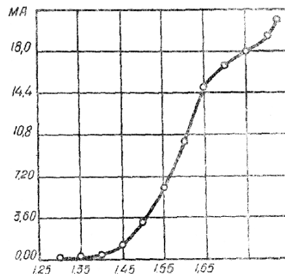
Рис. 6. Полярограмма гафния в водном растворе 0,1 M LiCl
