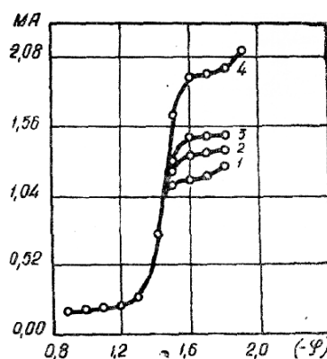
Рис. 2. Полярограмма ZrOCl на фоне 0,1 м LiCl в водно-метанольных смесях: 1 — 20%; 2 — 40%; 3 — 60%; 4 — 80% H_2O
