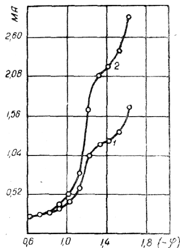
Рис. 4. Полярограммы ZrOCl 2 на фоне 0,1 M LiCl в этаноле
