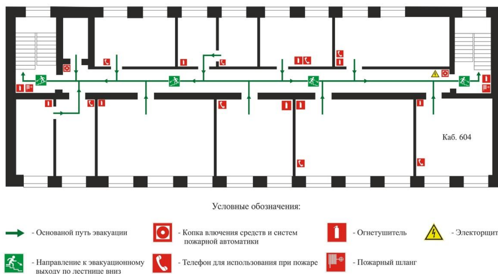
Рисунок 9 – План эвакуации при пожаре из кабинета №604.
