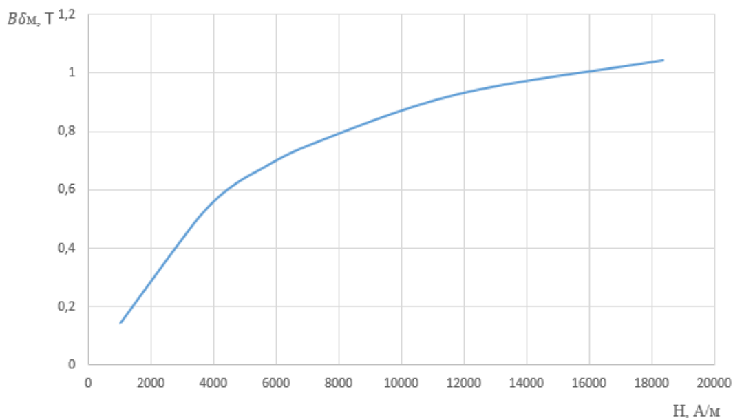
Рисунок 3.5 – Кривая намагничивания
