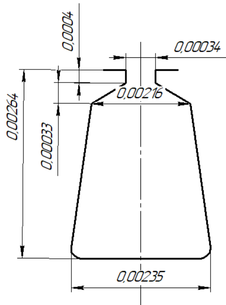
Рисунок 3.3 - Паз якоря
