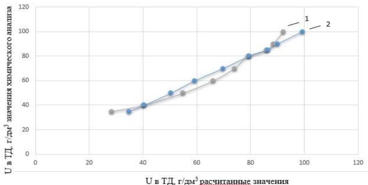
Рисунок 8 – Градуировочные кривые
