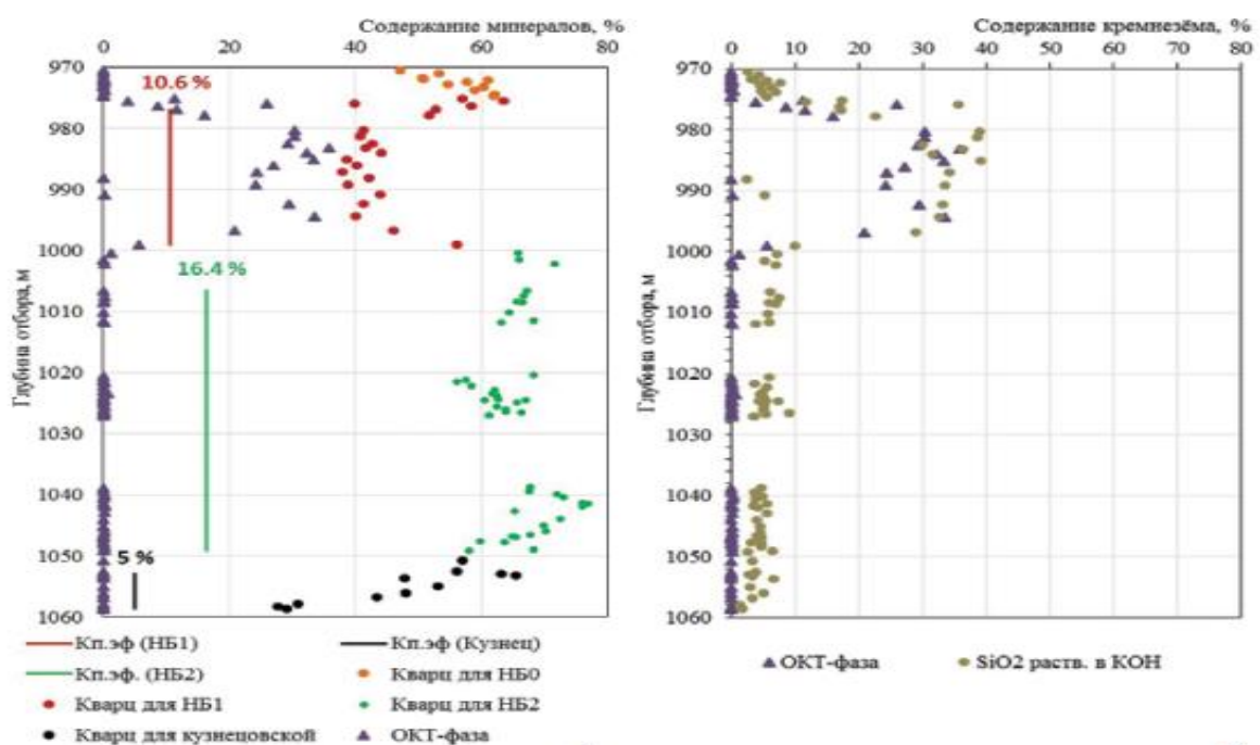
Рисунок 1.7 – Изменчивость минерального состава опок нижеберёзовской подсыты по разрезу: рисунок слева - данные рентгеноструктурного анализа. Рисунок справа - данные анализа растворимости породы в присутствии щелочей [9]
