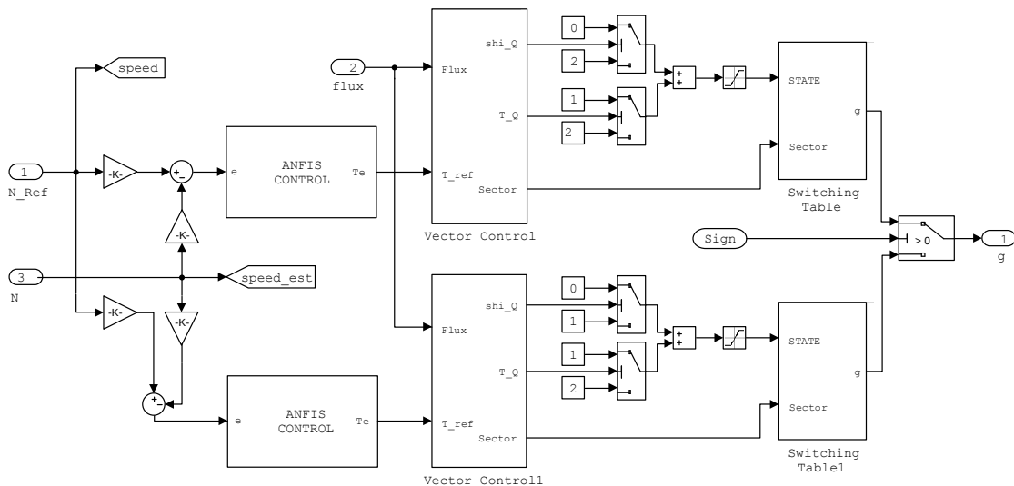
Рис. 5. Структурная схема имитационной модели блока «Векторное управление»
