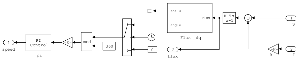
Рис. 7. Структурная схема имитационной модели блока, рассчитывающего текущую скорость и положение ротора
