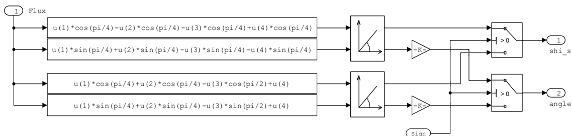
Рис. 6. Структурная схема имитационной модели блока, формирующего вектора потока
