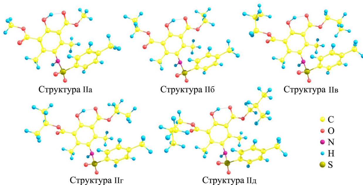
Рис. 2 – Геометрическое строение структур IIа-д
