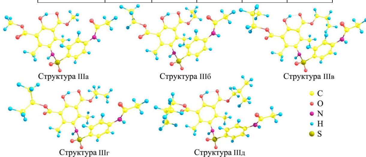
Рис. 3 – Геометрическое строение структур IIIа-д
