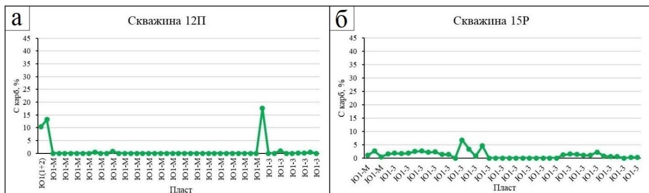
Рисунок 3.3. Карбонатность ( S_{\text{карб.}} ) образцов керна скважин 12П (а) и 15Р (б) Двуреченского месторождения.
