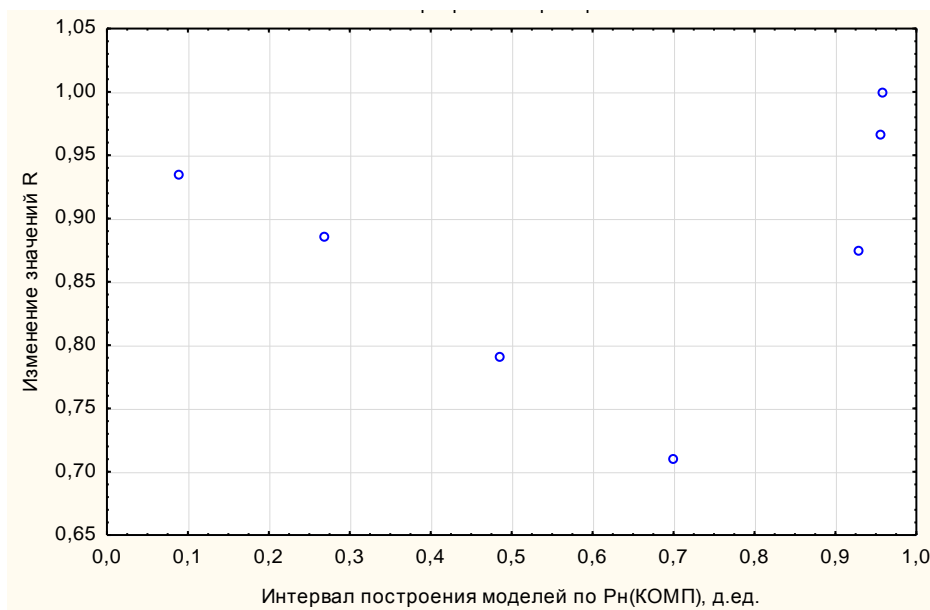
Рис. 3. Изменение коэффициента R от R_{H_{КОМП}} Fig. 3. Change in the coefficient R from R_{H_{КОМП}}
