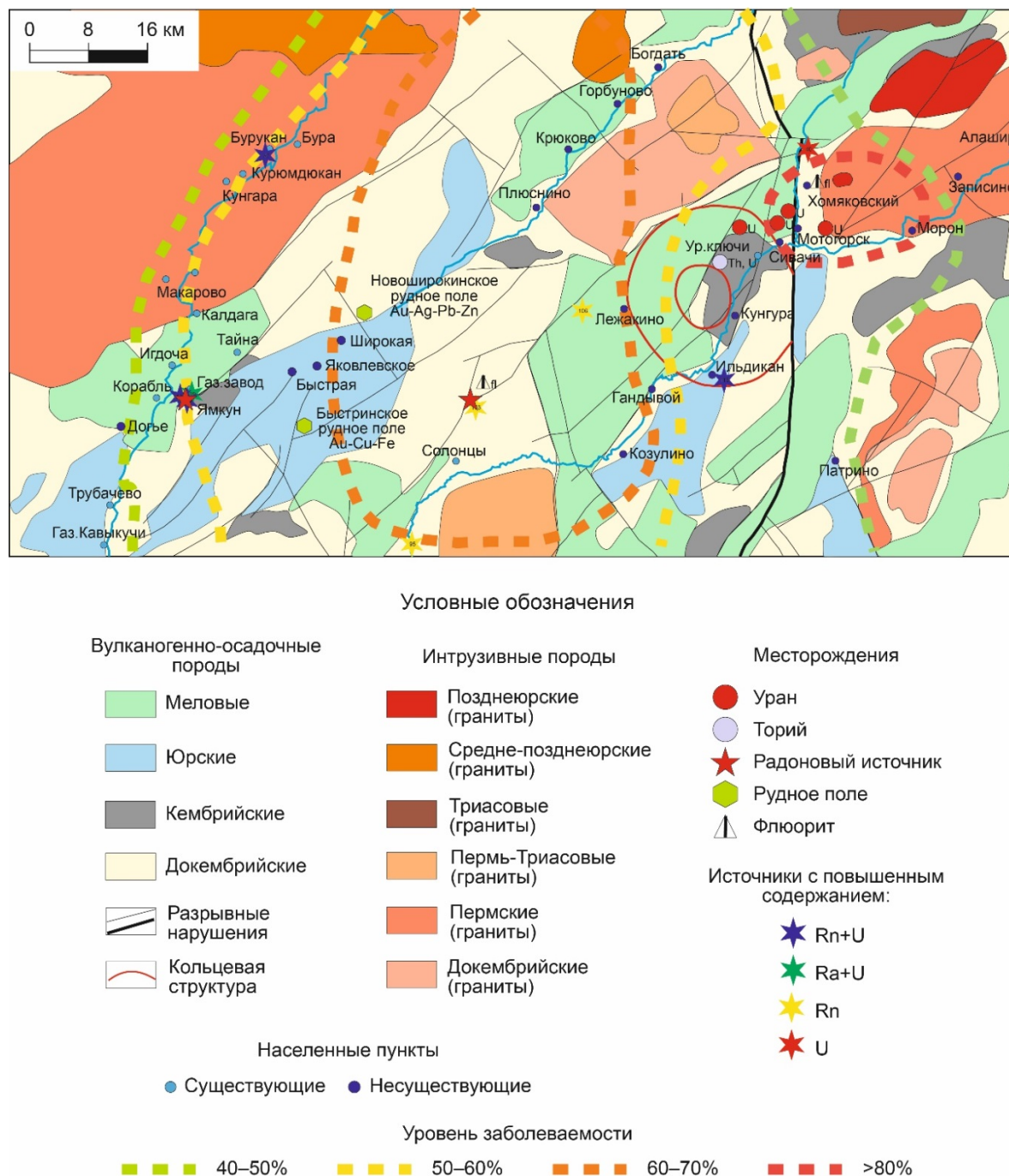
Рис. 2. Схематическая геологическая карта района исследований с элементами металлогении (масштаб 1:500000). Примечание: карта составлена по геологической карте масштаба 1:200000 на основе государственных листов M-50-V, M-50-VI [12]. Уровни заболеваемости приведены по [4]
