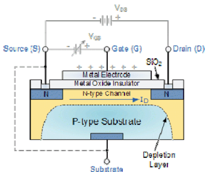
Рисунок 9 – Структура МОП-транзисторов
