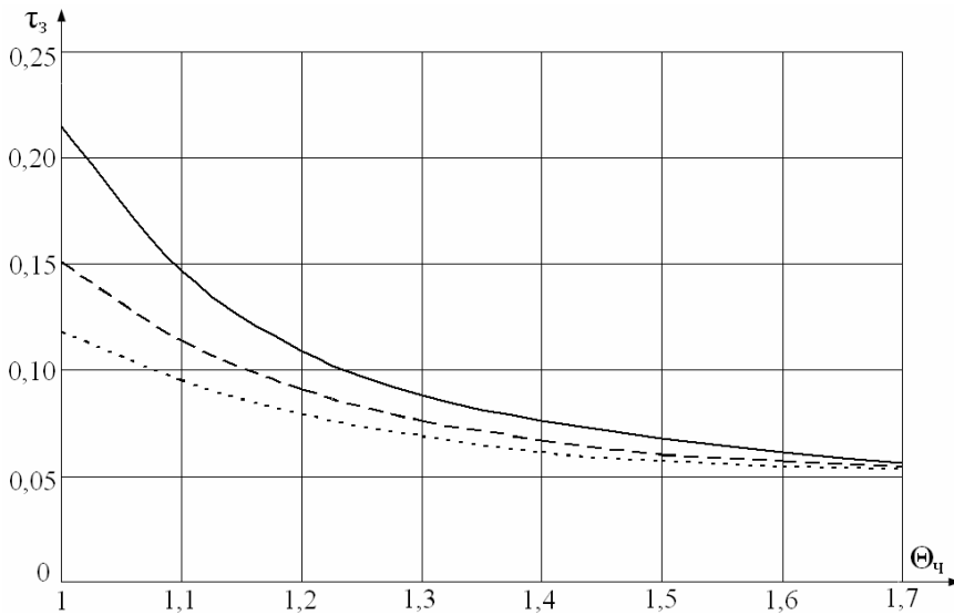
Рис. 7. Зависимость времени задержки зажигания от начальной температуры частицы \Theta_{\text{ч}} (— полусфера радиусом R_{\text{ч}}=0,15 ; — — диск размерами R_{\text{ч}}=Z_{\text{ч}}=0,15 ; - - - параллелепипед размерами H_{\text{ч}}=L_{\text{ч}}=0,15 )
