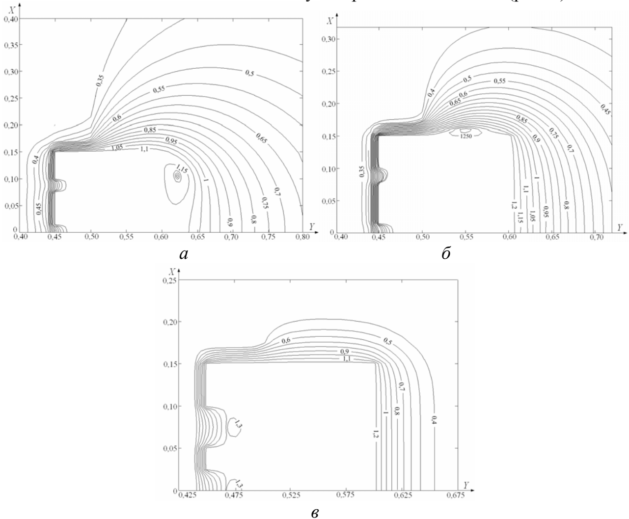
Рис. 5. Изотермы ( \Theta ) системы «жидкое топливо – шероховатая частица – окислитель» в момент воспламенения при \tau_3=0,549 , H_{ш}=0,1 , L_{ш}=0,2 , \Theta_ч=1,15 (а), \tau_3=0,267 , H_{ш}=0,1 , L_{ш}=0,2 , \Theta_ч=1,25 (б), \tau_3=0,126 , H_{ш}=0,2 , L_{ш}=0,4 , \Theta_ч=1,25 (в)
