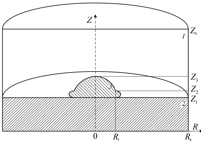
Рис. 13. Схема области решения задачи тепломассопереноса в системе «капля жидкого топлива – металлическая подложка – воздух»: 1 – парогазовая смесь, 2 – стальная подложка, 3 – капля жидкого топлива
