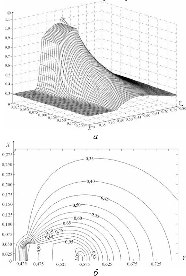
Рис. 2. Распределение температур (а) и положение характерных изотерм (б) в момент воспламенения при H_q=L_q=0,1 , \Theta_q=1
