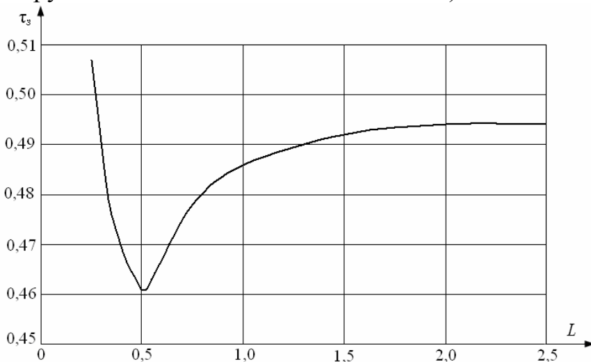
Рис. 9. Зависимость времени задержки зажигания от величины L при \Theta_{\text{ч}}=1
