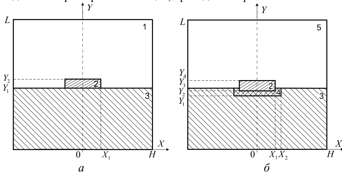
Рис. 1. Схема области решения задачи в начальный ( \tau=0 ) момент времени (а) и при 0 < \tau < \tau_3 (б): 1 – воздух, 2 – частица, 3 – жидкое горючее вещество, 4 – пары горючего, 5 – парогазовая смесь
