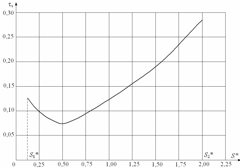
Рис. 8. Зависимость времени задержки зажигания \tau_z от отношения S^* при \Theta_{\text{ч}}=1,2 ( S_1^*=0,125 , S_2^*=2 )
