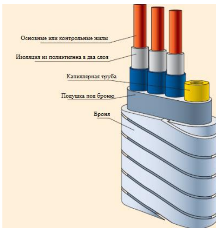
Рисунок 17 – Конструкция специального погружного кабельного устройства
