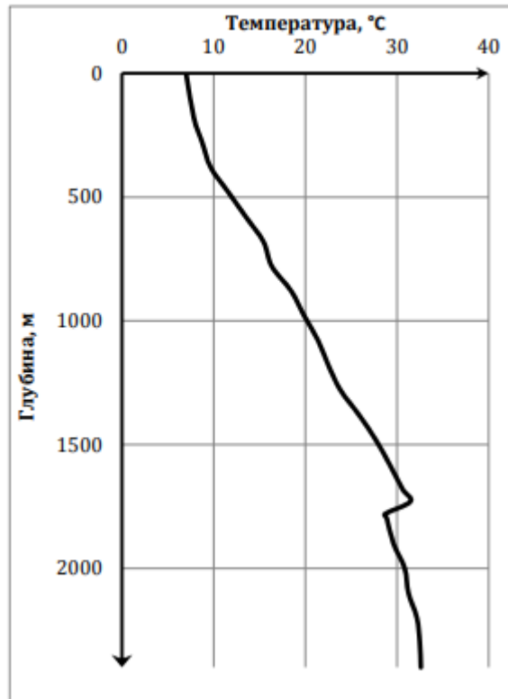
Рисунок 7 - Пример фактической скважинной термограммы
