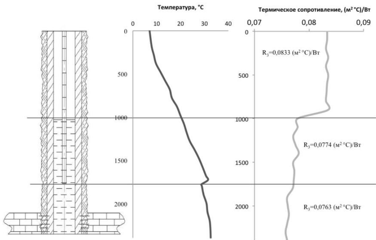
Рисунок 8 – Выделение интервалов скважины при определении термического сопротивления R
