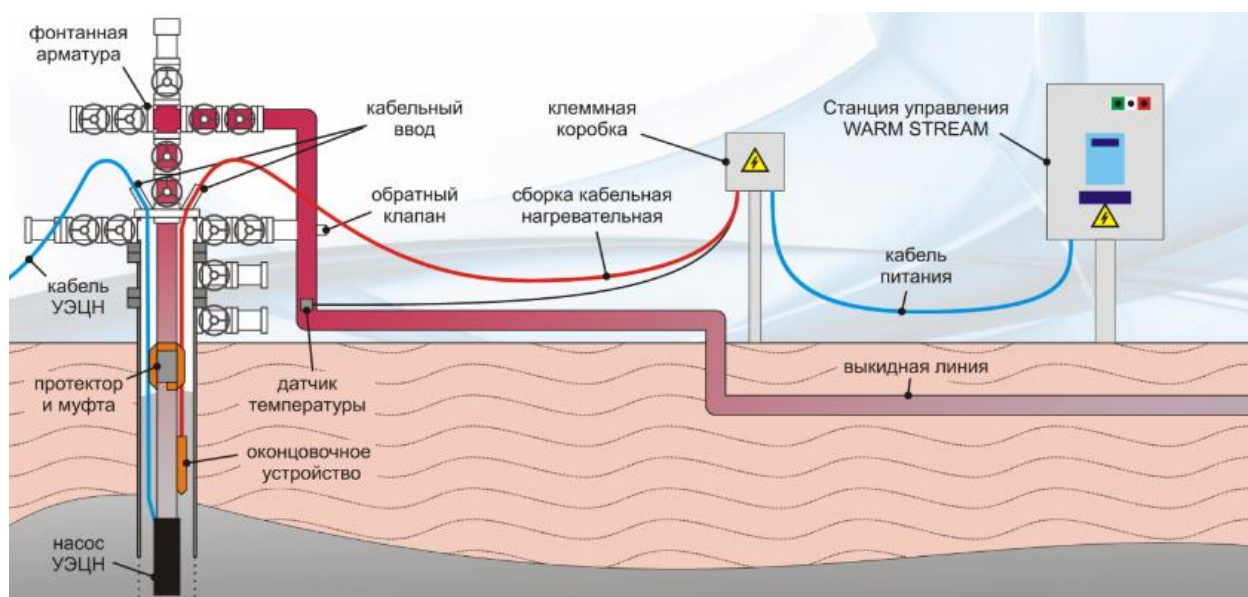
Рисунок 30 - Термоэлектрическая установка Warm Stream-1VPc размещением кабеля снаружи трубы НКТ
