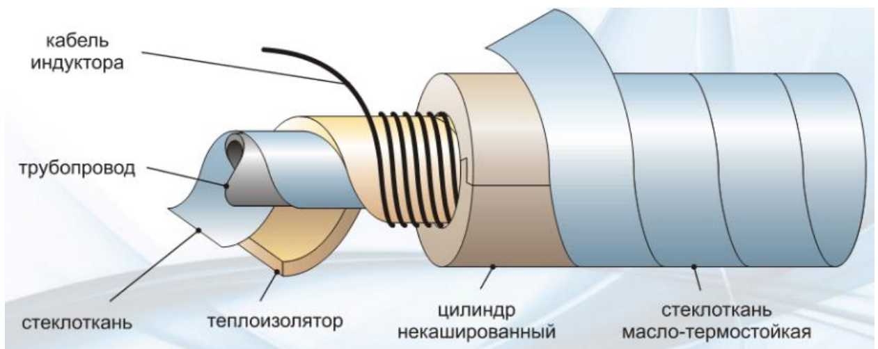
Рисунок 27 – Структурная схема индуктора
