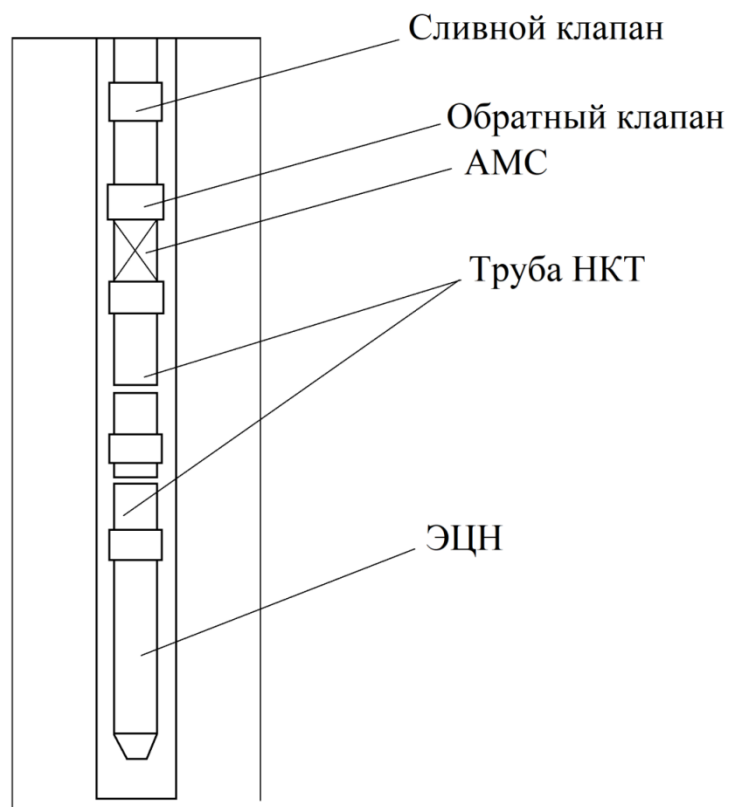
Рисунок 13 - Схема установки магнитного активатора в компоновке УЭЦН
