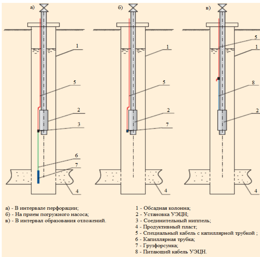
Рисунок 16 – Схема дозирования химического реагента в скважину с применением СПКУ
