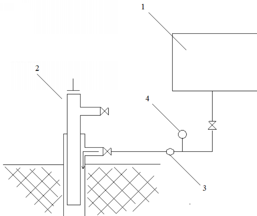
Рисунок 15 – Обвязка дозирующего устройства для подачи реагента в затрубное пространство скважины; 1- установка дозирования реагента, 2 – фонтанная арматура, 3 – обратный клапан, 4 - манометр
