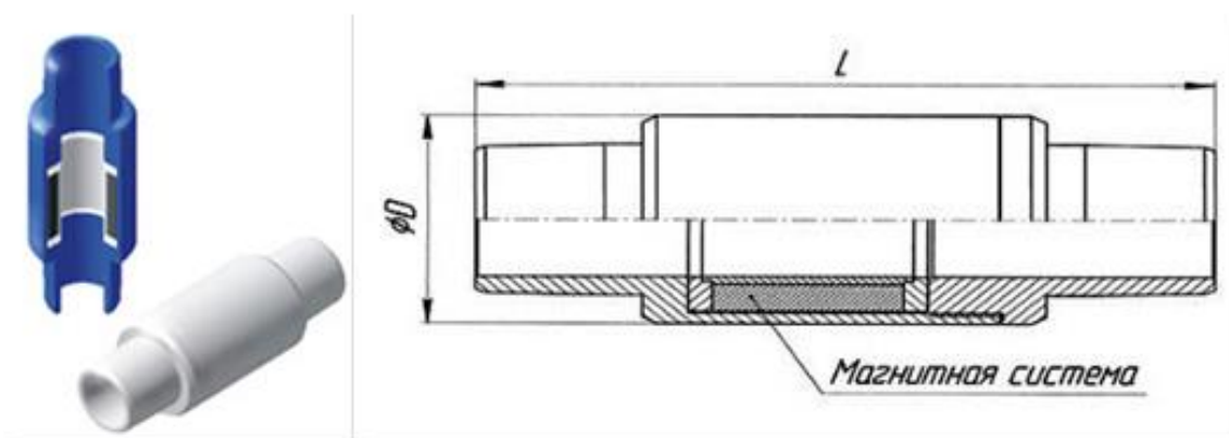
Рисунок 12 - Магнитный активатор АМС-73М
