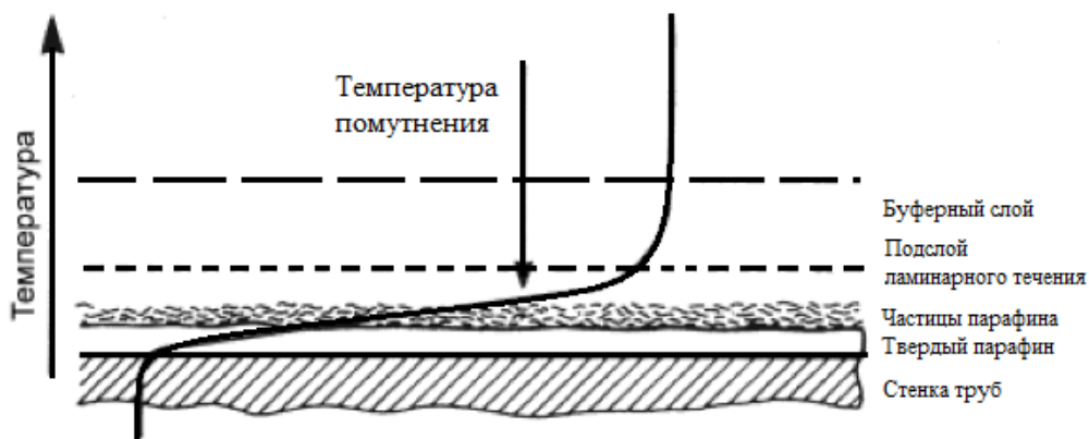
Рисунок 37 – Профиль температуры в продольном сечении трубы
