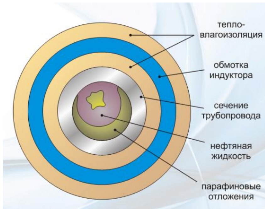
Рисунок 26 – Схема Warm Stream-1VP индукционного типа в разрезе
