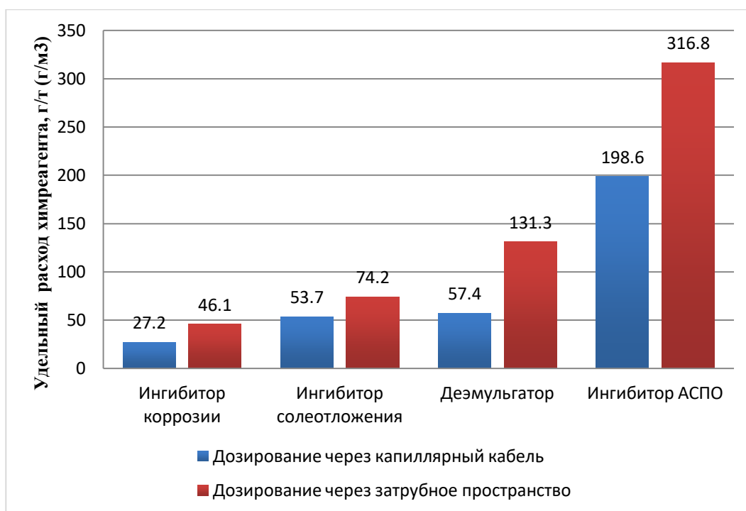
Рисунок 18 – Удельные расходы химических реагентов до и после внедрения технологии дозирования химических реагентов посредством капиллярного устройства
