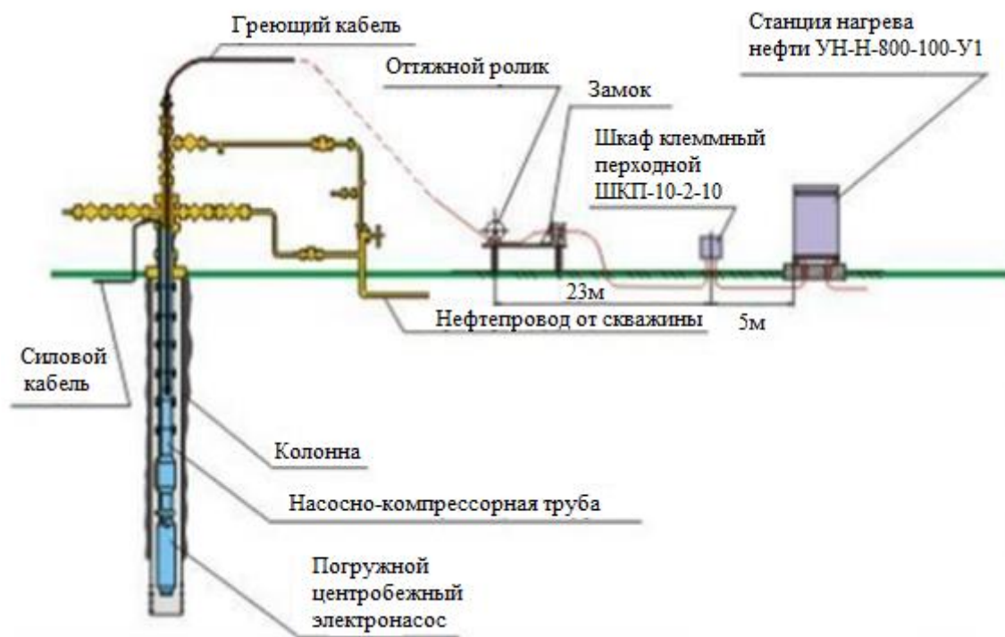
Рисунок 21 – Установка для спуска нагревательного кабеля и депарафинизации
