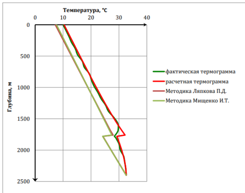
Рисунок 36 – Термограмма скважины Сибирского месторождения
