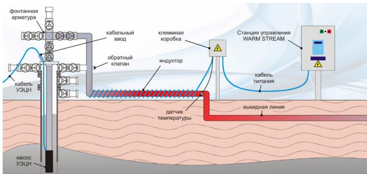
Рисунок 25 -Термоэлектрическая установка Warm Stream-1 VP
