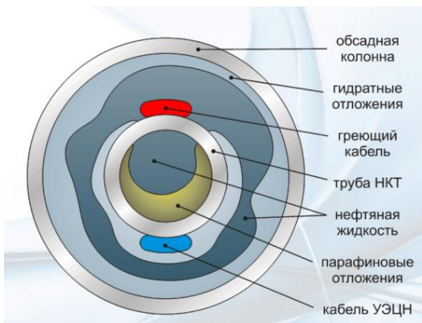
Рисунок 32 – Схема Warm Stream-1VP с размещением кабеля снаружи трубы НКТ в разрезе
