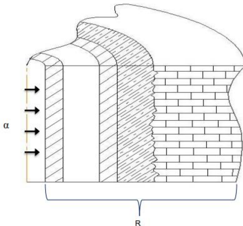
Рисунок 6 - Схема теплопередачи от жидкости стенке скважины
