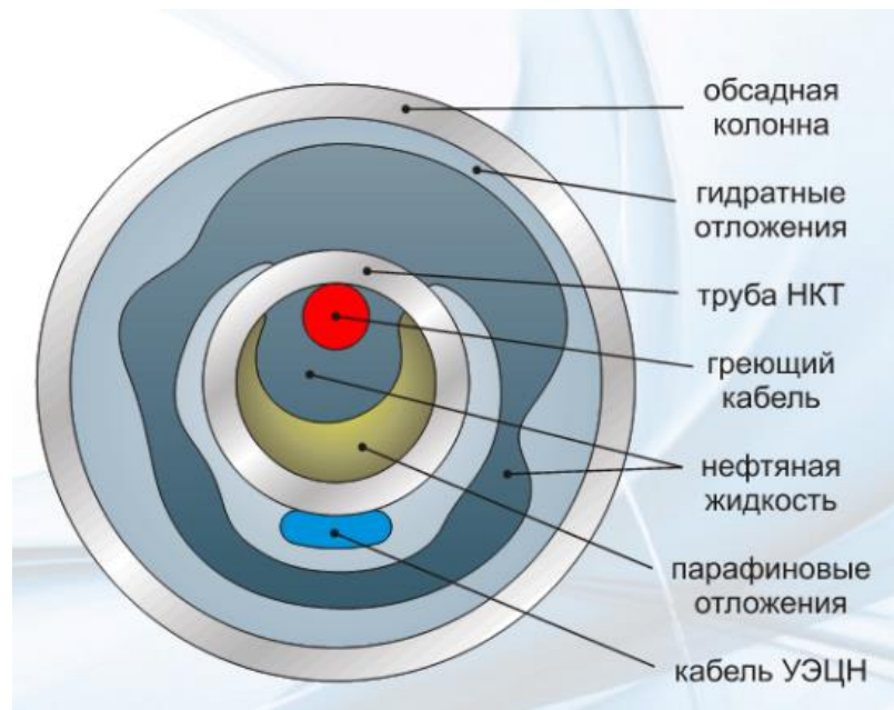
Рисунок 33 – Схема Warm Stream-1VP с размещением кабеля внутри трубы НКТ в разрезе
