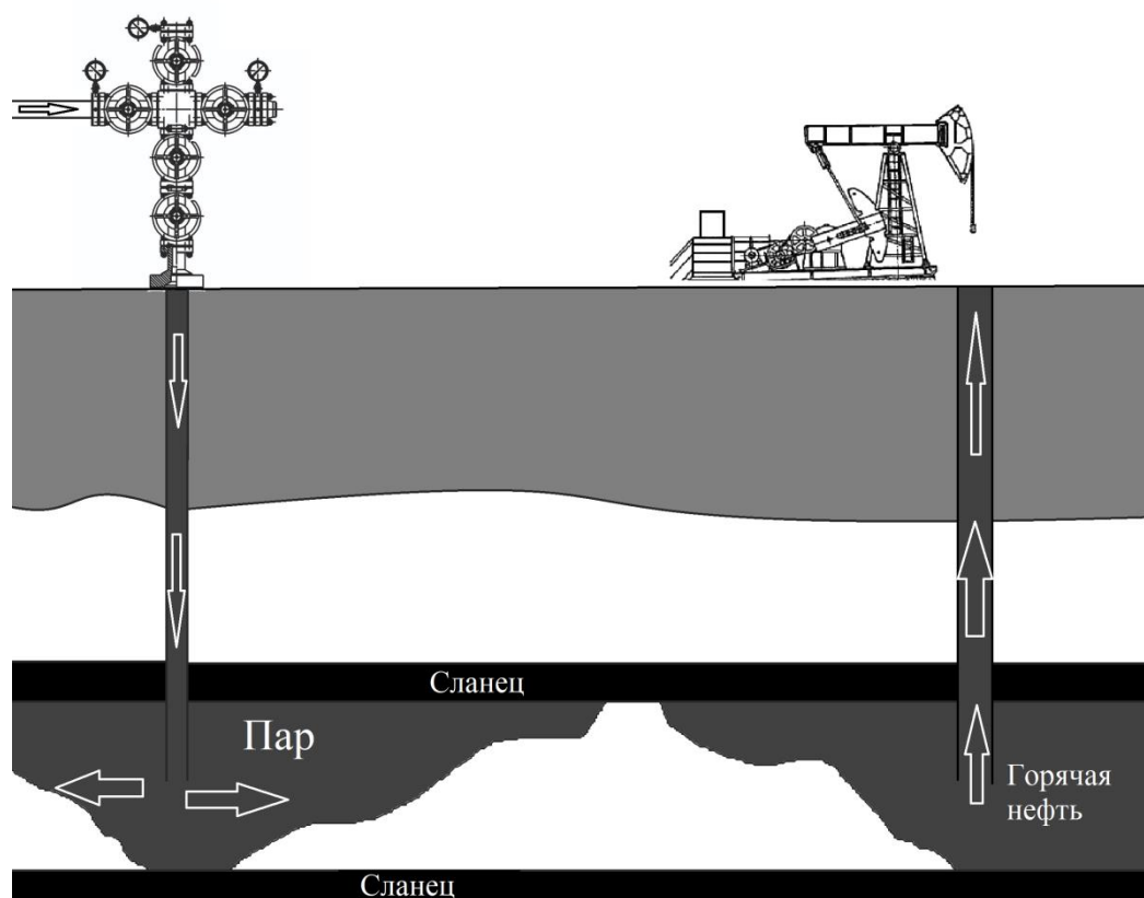
Рисунок 22 – Схема вытеснения и прогрева нефти водяным паром
