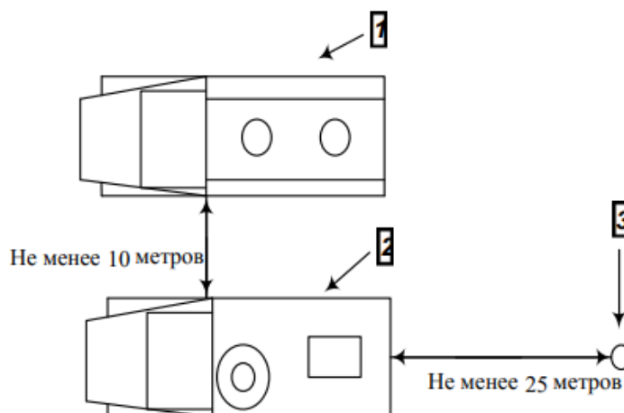
Рисунок 19 – Схема обвязки наземного оборудования (1 – автоцистерна, 2 – агрегат типа АДПМ, 3 – устье скважины)
