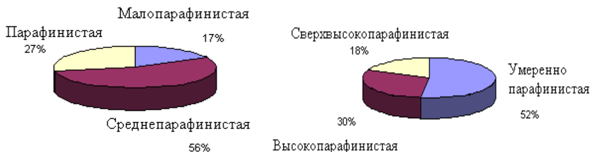
Рисунок 3 - Диаграмма распределение нефтей мира по содержанию парафинов
