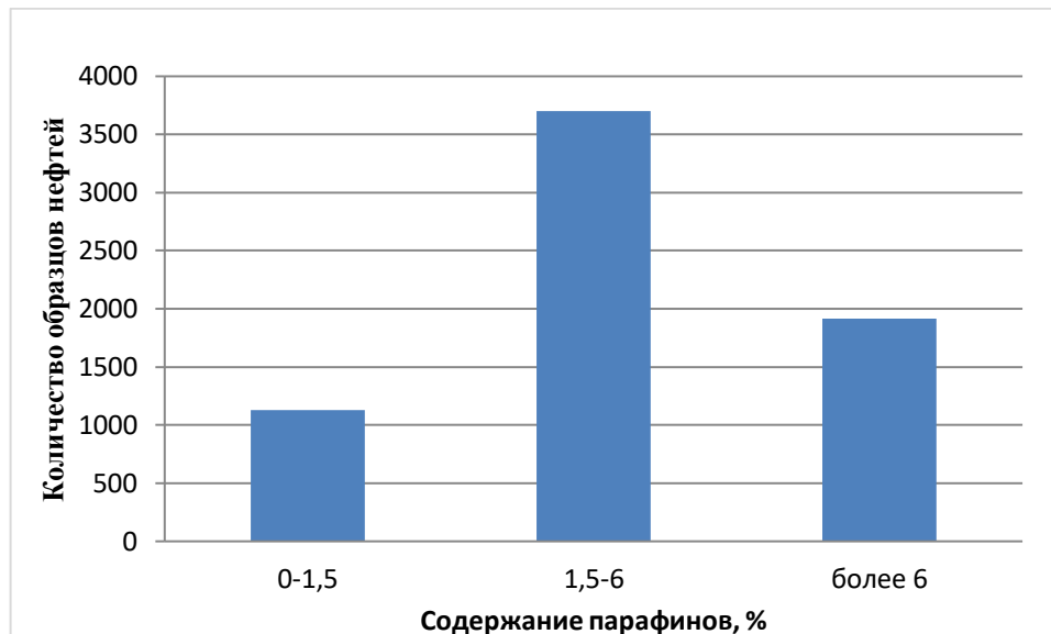
Рисунок 2 - Диаграмма распределение нефтей мира по содержанию парафинов
