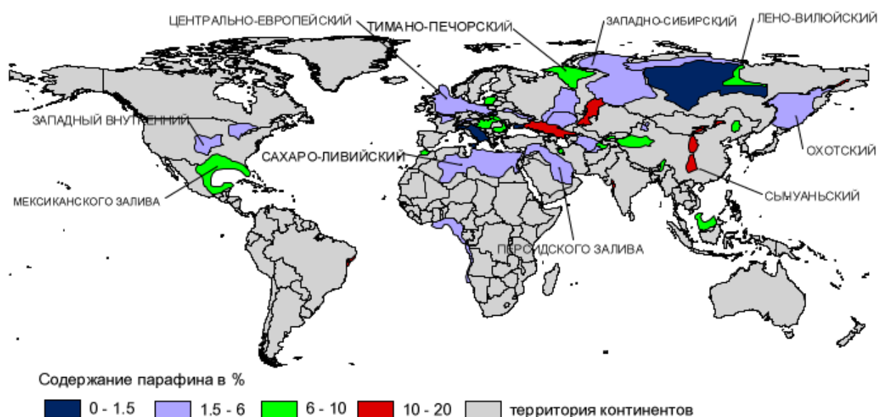
Рисунок 4 - Распределение нефтегазоносных бассейнов с парафинистыми нефтями на территории континентов
