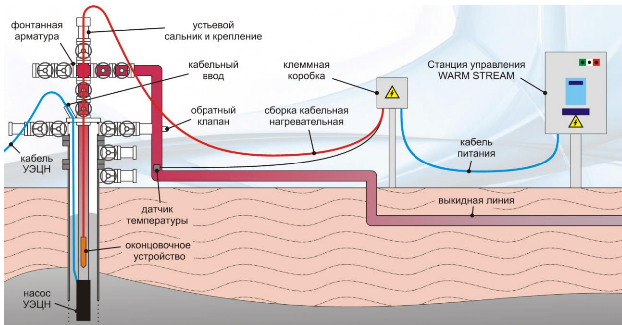
Рисунок 31 - Термоэлектрическая установка Warm Stream-1 VPc размещением кабеля внутри трубы НКТ
