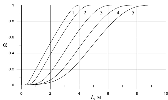
Рис. 7. Распределение степени термического разложения полиурната аммония при разном массовом расходе исходного вещества
