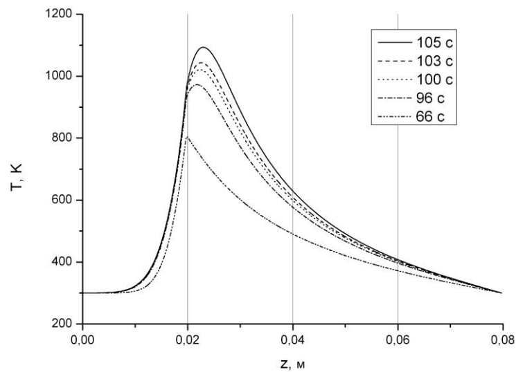
Рис. 9 Распределение температуры в системе “слой ЛГМ-газовая смесь” до и в момент зажигания при q_s=15000 \text{ Вт/м}^2
