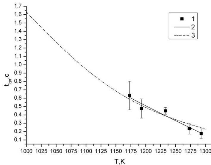
Рис. 4. Зависимость времени задержки зажигания ЛГМ от начальной температуры частицы: 1 – экспериментальные точки, 2 – аппроксимирующая прямая, 3 - теоретическая зависимость
