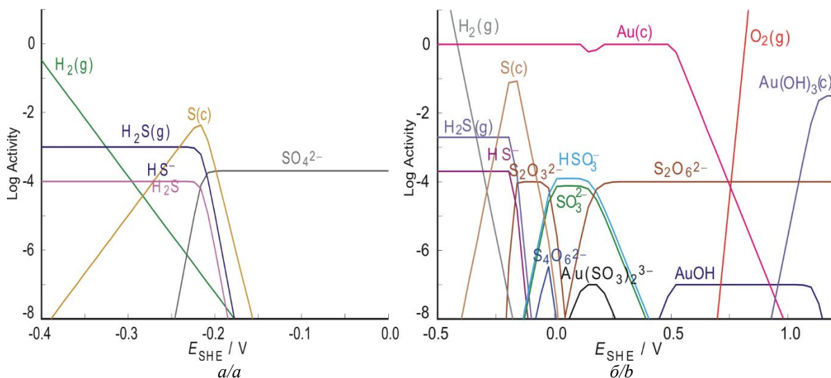
Рис. 4. Расчётные диаграммы «активность–потенциал» а) равновесных ионно-молекулярных форм в системе S–H 2 O и б) метастабильных ионно-молекулярных форм (при отсутствии SO_4^{2-} -ионов) в системе S–Au–H 2 O при pH=7 , [S]_{сум}=1 \cdot 10^{-4} М, [Au]_{сум}=1 \cdot 10^{-7} М, t=25 °С
