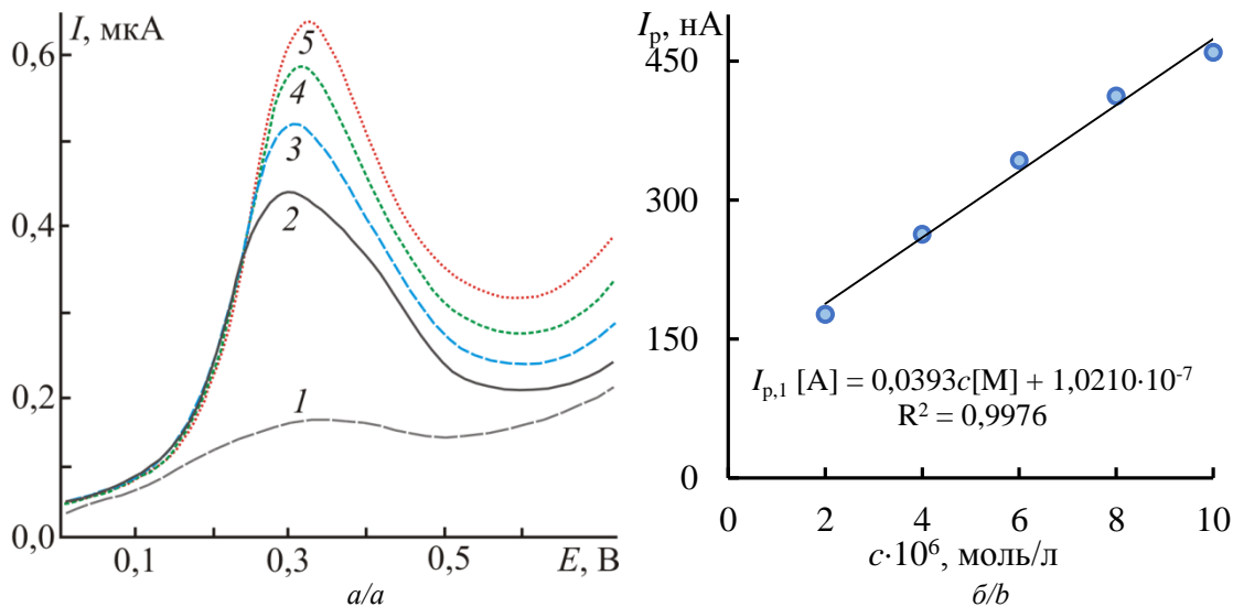
Рис. 3. а) вольтамперограммы модифицированного электрода AuУКЭ в растворах 0,05 М KNO_3 + Na_2S_2O_3 ( E_{нач}=0,0 В, E_{кон}=0,6 В, v=100 мВ/с, pH=7 , деаэрирование растворов азотом) при различных концентрациях тиосульфата натрия, М: 1) фоновая кривая; 2) 2 \cdot 10^{-6} ; 3) 4 \cdot 10^{-6} ; 4) 6 \cdot 10^{-6} ; 5) 8 \cdot 10^{-6} ; б) зависимость тока окисления I_{p,1} при E_{p,1} \approx 0,3 В от концентрации S_2O_3^{2-} -ионов в растворе (фоновый электролит 0,05 М KNO_3 )
