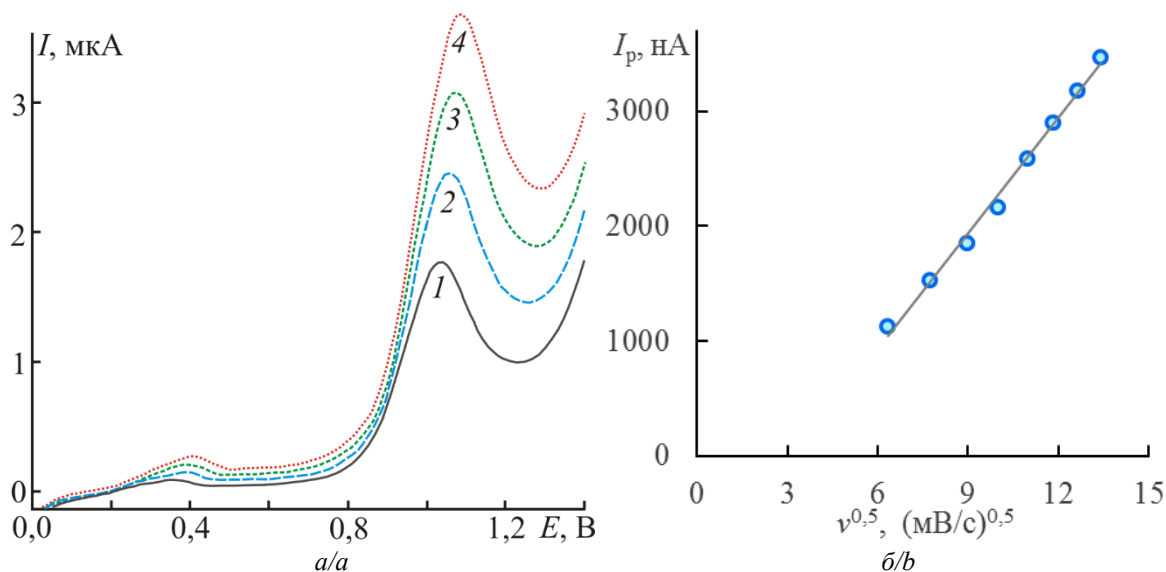
Рис. 5. а) вольтамперограммы модифицированного электрода AuУКЭ в растворе 0,05 \text{ M Na}_2\text{SO}_4 + 1 \cdot 10^{-4} \text{ M Na}_2\text{S}_2\text{O}_3 ( E_{\text{нач}}=0,0 \text{ В} , E_{\text{кон}}=1,4 \text{ В} , \text{pH}=7 , деаэрирование растворов азотом) при различной скорости развертки потенциалов, мВ/с: 1) 40; 2) 60; 3) 80; 4) 100; б) зависимость тока окисления I_{p,2} при E_{p,2} \approx 1,1 \text{ В} от корня квадратного из скорости развертки потенциала в интервале v=40 \dots 180 \text{ мВ/с} (фоновый электролит 0,05 \text{ M Na}_2\text{SO}_4 )
