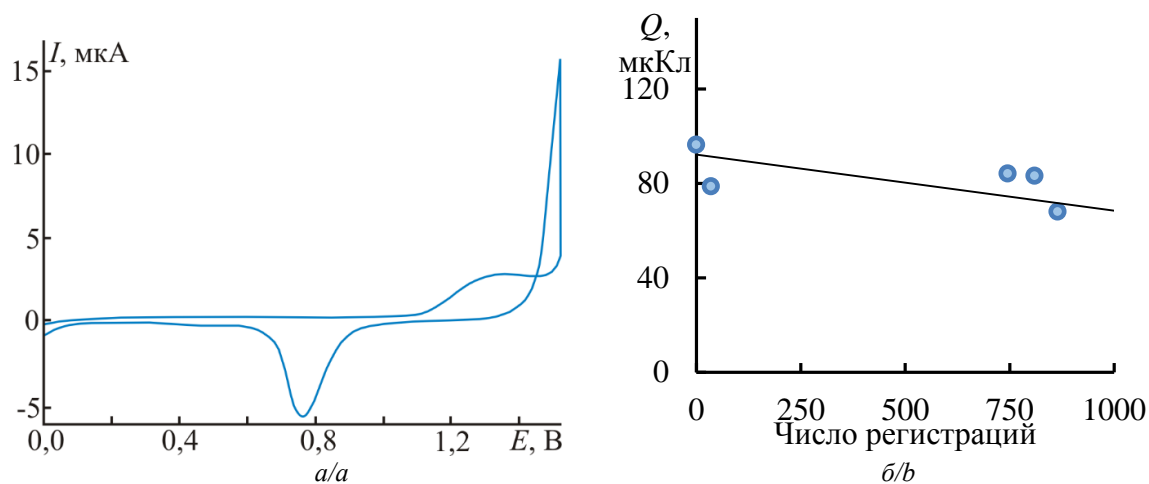
Рис. 6. а) циклическая вольтамперограмма модифицированного электрода AuУКЭ в растворе 0,05 \text{ M H}_2\text{SO}_4 ( E_{\text{нач}}=0,0 \text{ В} , E_{\text{кон}}=1,5 \text{ В} , v=100 \text{ мВ/с} , деаэрирование раствора азотом); б) зависимость количества электричества Q , затраченного на катодное восстановление (гидроксидов Au в интервале потенциалов 1,0 \dots 0,6 \text{ В} , от числа регистраций вольтамперограмм в растворе 0,05 \text{ M Na}_2\text{SO}_4 + 1 \cdot 10^{-4} \text{ M Na}_2\text{S}_2\text{O}_3 без обновления поверхности электрода
