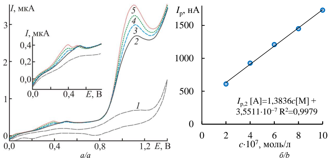
Рис. 2. а) вольтамперограммы модифицированного электрода AuУКЭ в растворах 0,05 М Na_2SO_4 + Na_2S_2O_3 ( E_{нач}=0,0 В, E_{кон}=1,4 В, v=100 мВ/с, pH=7 , деаэрирование растворов азотом) при различных концентрациях тиосульфата натрия, М: 1) фоновая кривая; 2) 2 \cdot 10^{-7} ; 3) 4 \cdot 10^{-7} ; 4) 6 \cdot 10^{-7} ; 5) 8 \cdot 10^{-7} ; на врезке – участки вольтамперограмм в интервале потенциалов 0,0...0,6 В; б) зависимость тока окисления I_{p,2} при E_{p,2} \approx 1,1 В от концентрации S_2O_3^{2-} -ионов в растворе (фоновый электролит 0,05 М Na_2SO_4 )
