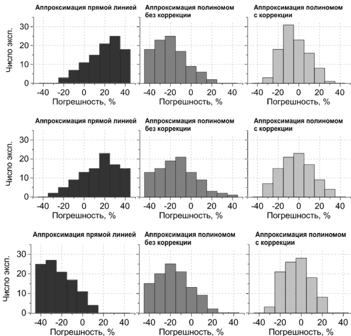
Рис 7. Гистограммы погрешности определения массовой концентрации ионов Zn, As и Cu (сверху-вниз)
