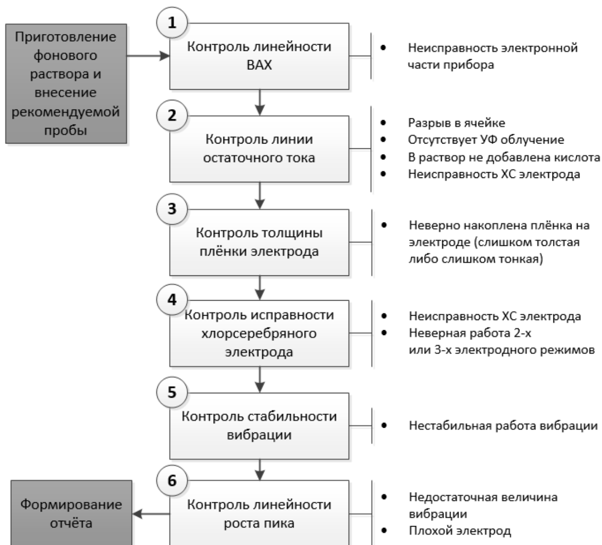
Рис 8. Этапы проверки системы вольтамперного анализа
