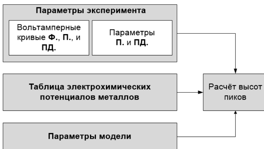
Рис 3. Структурная схема расчёта концентрации химических элементов, методом введено-найдено
