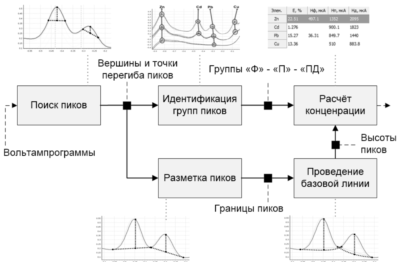
Рис 4. Последовательность автоматизации выделения аналитического сигнала
