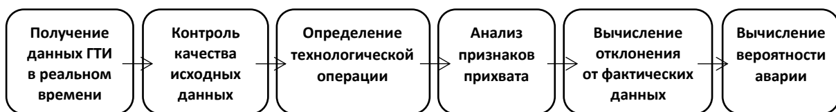
Рис. 2. Блок-схема системы прогнозирования вероятности прихвата
