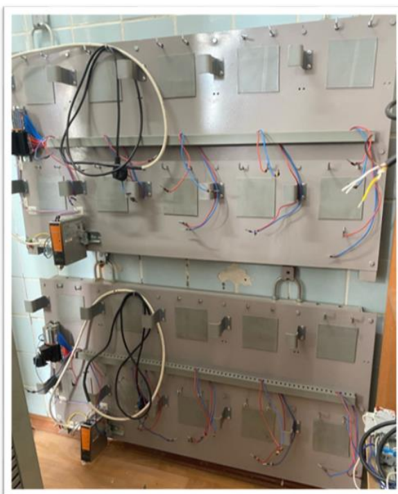
Рисунок 2.11 – Стенд для поверки СИ образца 2019 года
