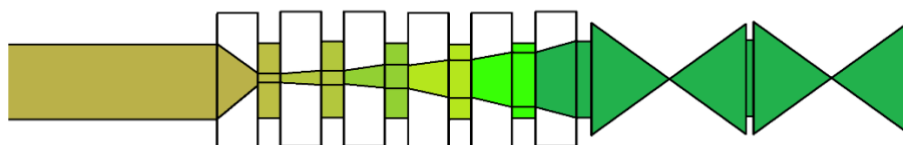
Рисунок 22 – Условная схема многоступенчатого штуцера дискретного регулируемый (ШДР)
