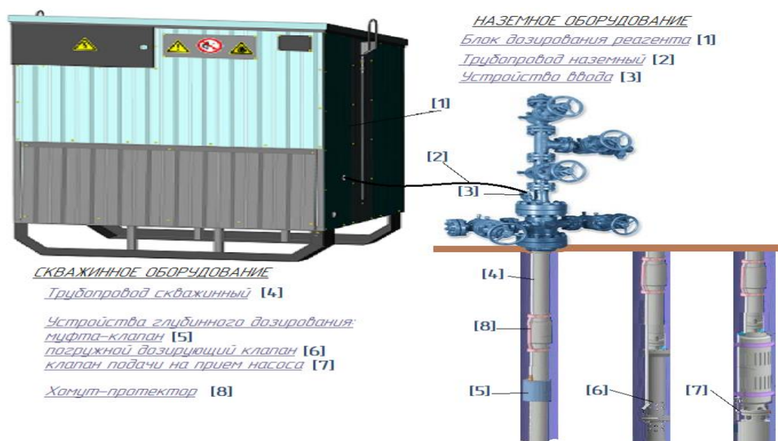
Рисунок 27 – Оборудование подачи реагента, схема обвязки
