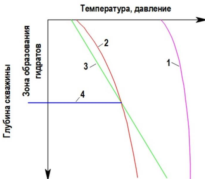
Рисунок 12 – Определение зоны возможного образования гидратов
