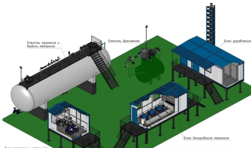
Рисунок 11 – Метанольное хозяйство (склад метанола)
