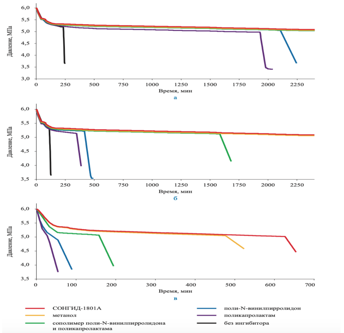
Рисунок 25 – Оценка эффективности ингибиторов по времени задержки начала гидратообразования при температурах а – 10 °С, б – 3 °С, в – (-4) °С
