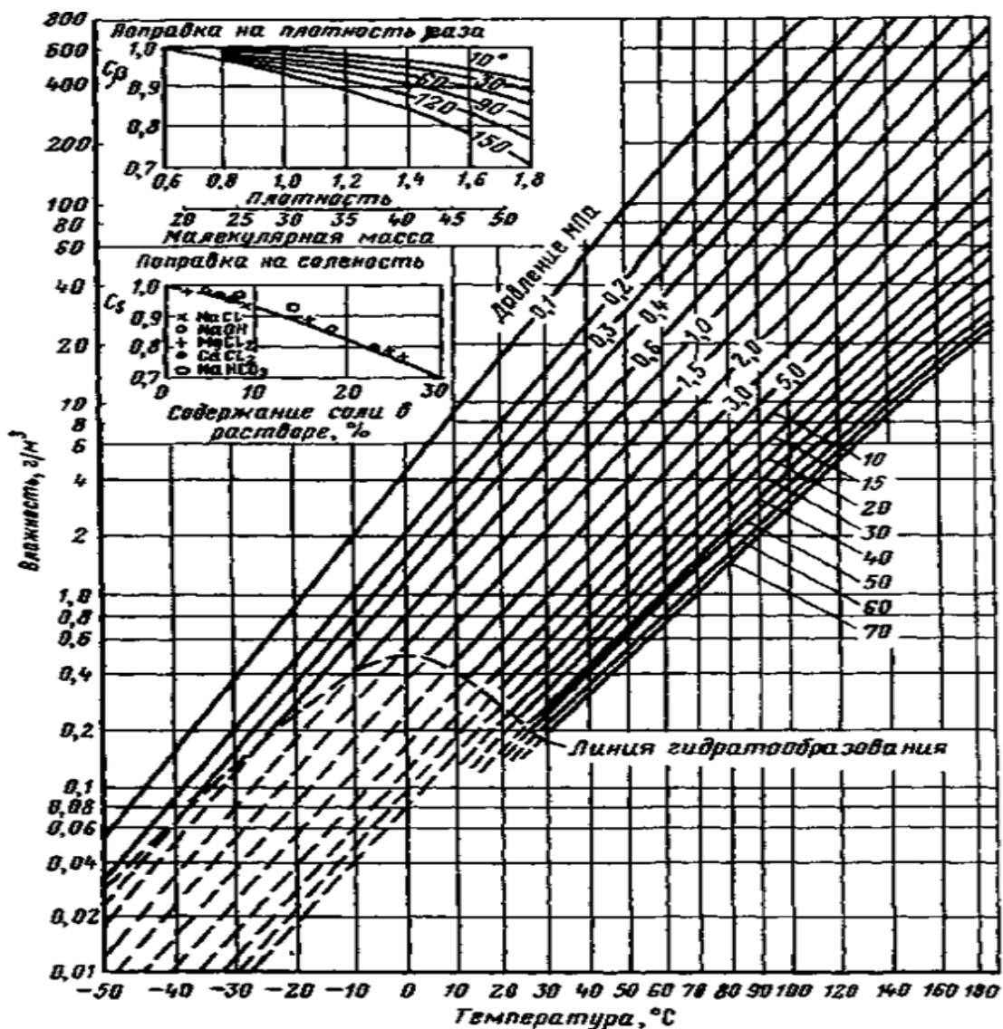
Рисунок 7 – Максимальное содержание водяных паров в природном газе в зависимости от давления и температуры
