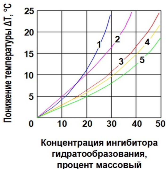
Рисунок 15 – Зависимость снижения температуры гидратообразования от концентрации ингибитора
