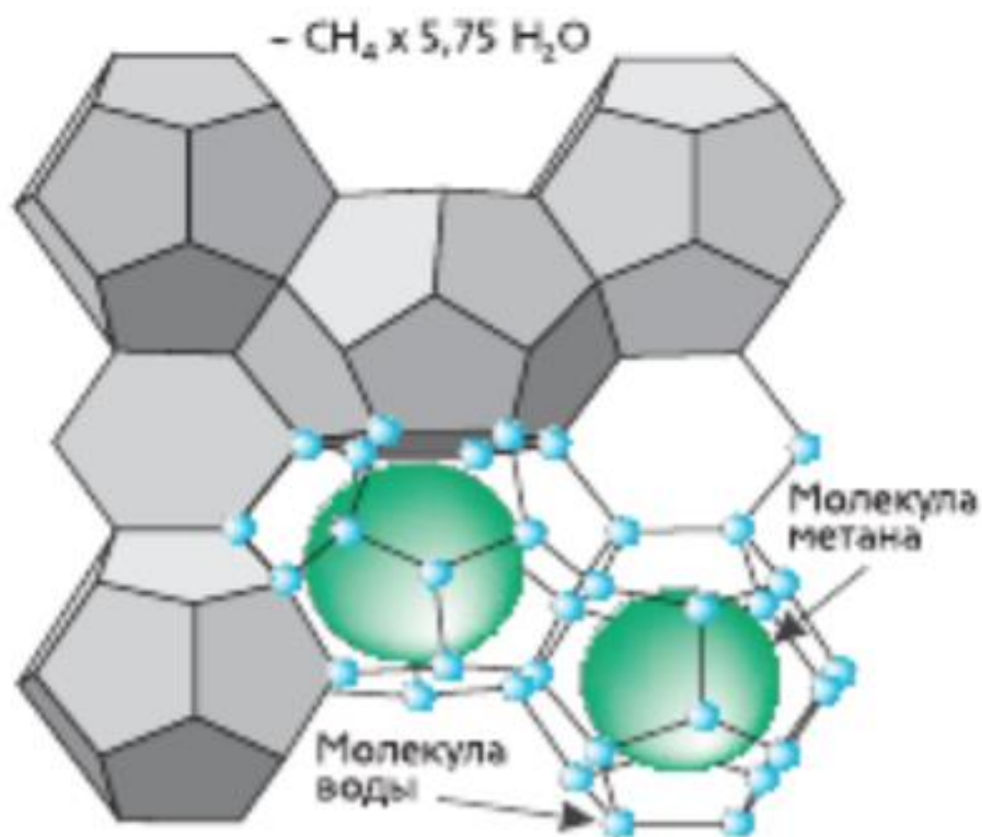
Рисунок 1 – Структура газового гидрата
