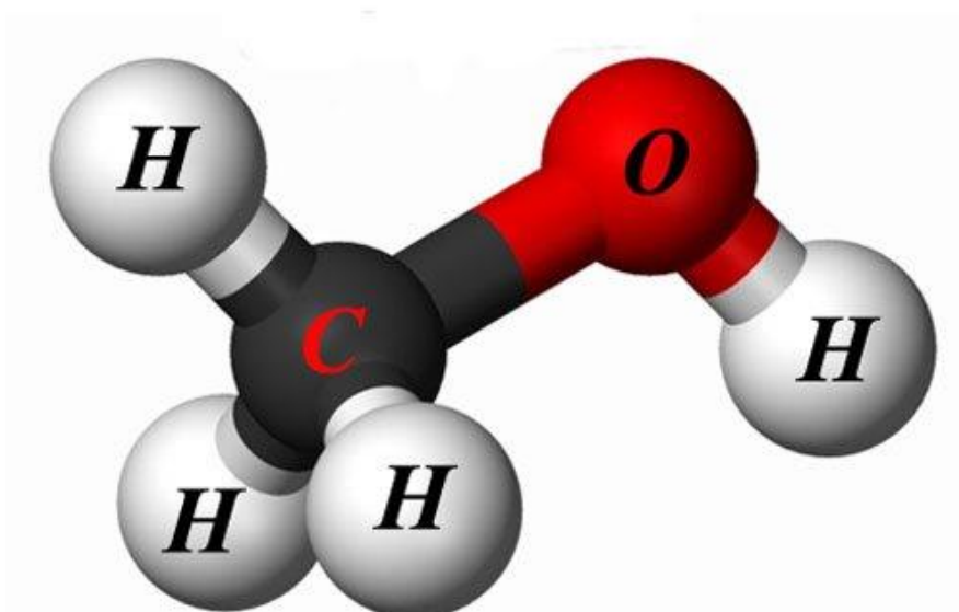
Рисунок 10 – Структура метанола
