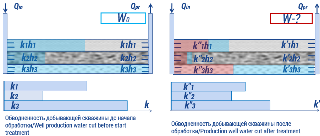
Рис. 1. Модель для описания технологии выравнивания профиля притока
