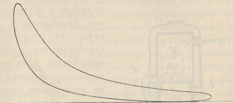
Индикаторная диаграмма двигателя Тринклера. Нагрузка 14,6 лш. с., число обор. 215, пружина — 1 мм.
