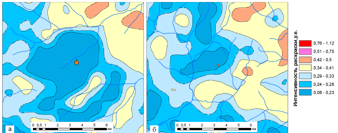
Рис. 6. Проявление рудного поля Светлое (а) и Дюльбакинской площади (б) в поле K/Th отношения
