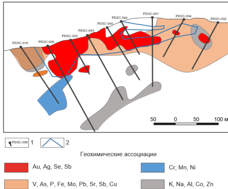
Рис. 5. Карта распределения геохимических ассоциаций по результатам факторного анализа по разведочной линии 7500 (масштаб 1:5 000).
