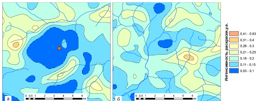
Рис. 7. Проявление рудного поля Светлое (а) и Дюльбакинской площади (б) в поле KU/ThTh отношения
