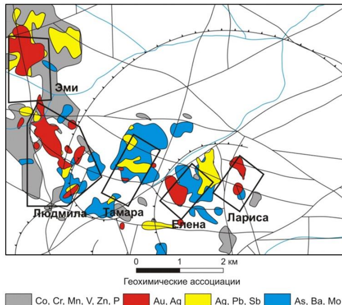
Рис. 3. Карта распределения геохимических ассоциаций по результатам факторного анализа (масштаб 1 : 10 000)
