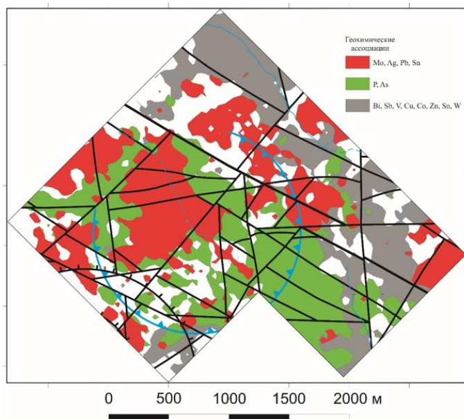
Рис. 10. Распределение геохимических ассоциаций на участке Дюльбаки по данным факторного анализа. Условные обозначения см. на рис. 8 и 9
