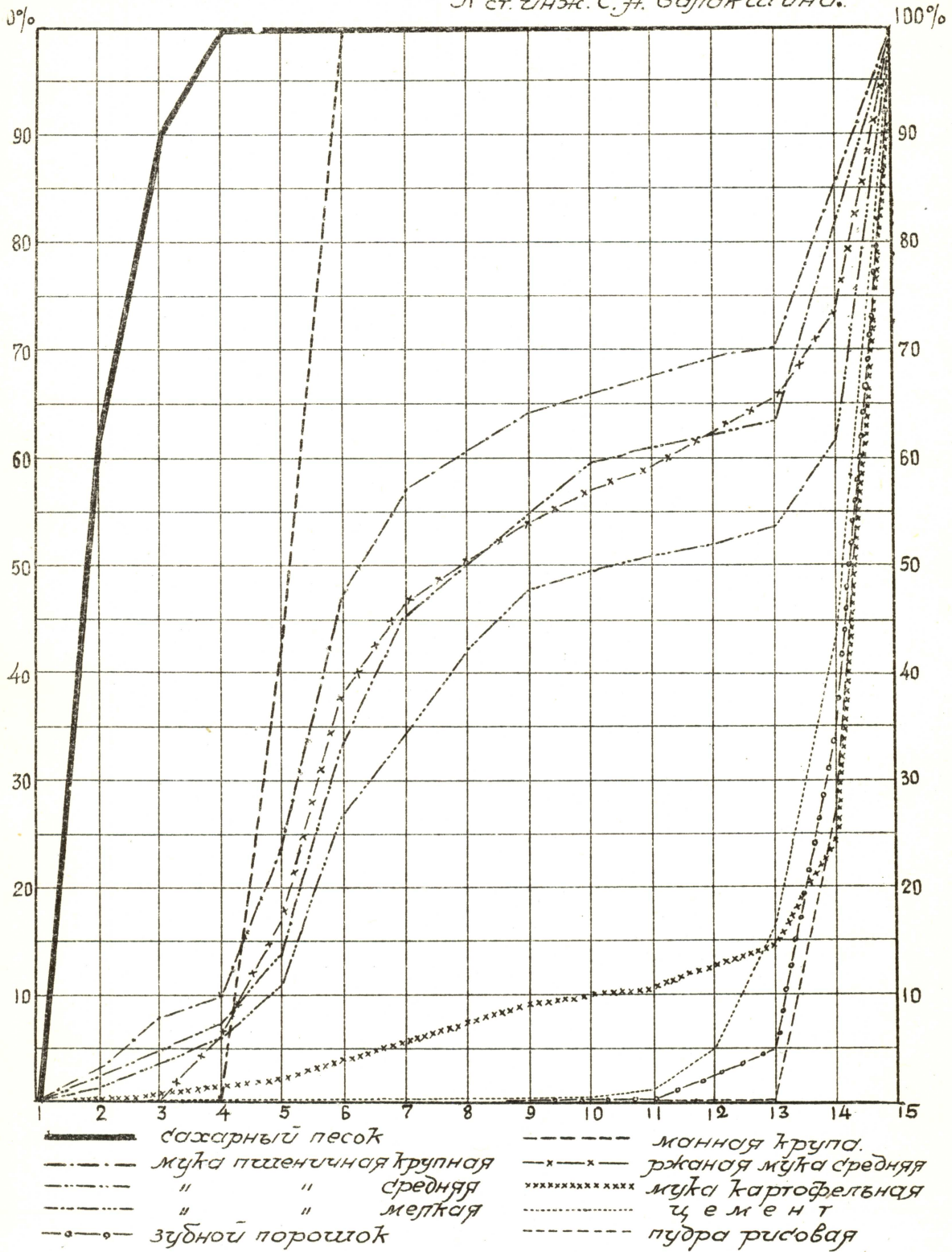
Рис. 13. Куммулятивные кривые крупности полученные гранометром для различных продуктов.
