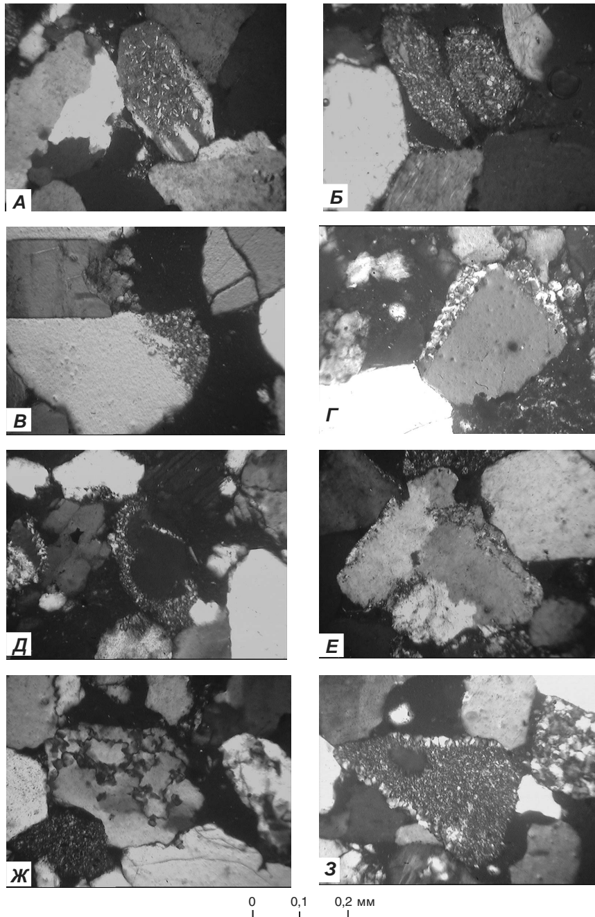
Рис. 1. Особенности изменения обломков в песчаниках: А) реликтовое зерно средне измененного (серицитизированного) плагиоклаза с сохранившимся двойниковым строением; Б) реликты зерен сильно измененного (серицитизированного) плагиоклаза; В) растворение кварцевого зерна в участке, выступающем в свободную пору; Г, Д) растворение и грануляция кварцевых обломков по краям; Е, Ж) растворение кварца, подчеркнутое нефтяным веществом; 3) перекристаллизация обломка кремнистой породы
