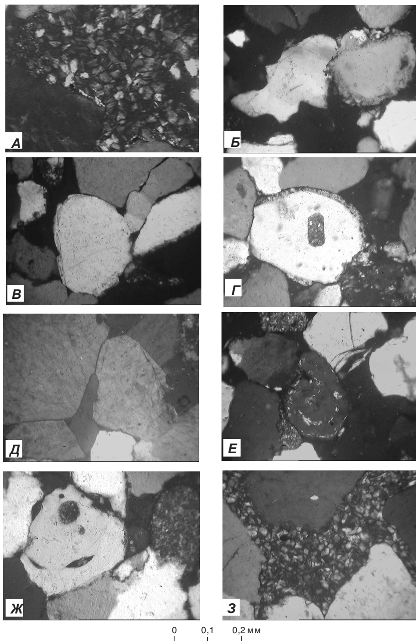
Рис. 3. Особенности цемента песчаников: А) пленочный гидрослюдястый и поровый каолиновый цемент; Б, В) регенерационный кварцевый с пленкой битума на материнском зерне; Г) инкрустационный кварцевый с плохо образованными кристаллами вторичного кварца; Д) регенерационный кварцевый с уничтожением пор; Е) регенерационный полевошпатовый с каймой, отделенной чешуйками слюды; Ж) регенерационный кварцевый с каймой, "законсервировавшей" капли нефти; 3) поровый крупнопакетный каолиновый
