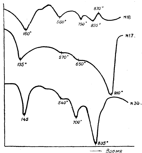
Рис. 3. Дифференциальные кривые нагревания. № 16—туфогенный алевролит, № 17 — мергель (обизвесткованный алевролит), № 30 — глинистая фракция известковистой глины коры выветривания. Все образцы отобраны из скважины 682.
