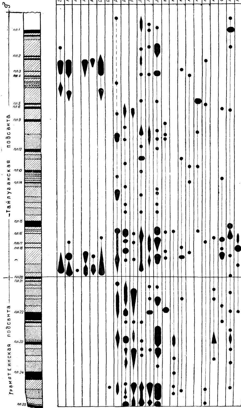
Рис. 2. Распределение органических остатков в отложениях ерунаковской свиты по Северо-Талдинской разведочной линии
