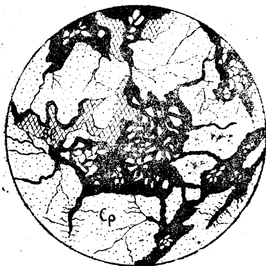
Рис. 12. Замещение ковеллина первой генерации (белый) халькозином (черный). Ср—халькопирит; Sl—сфалерит. Ув. 375.
