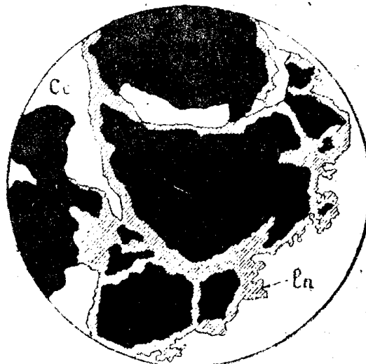
Рис. 15. Лимонит (ln) по пириту (черный) и по халькозину. Белый — халькозин. Ув. 300.
