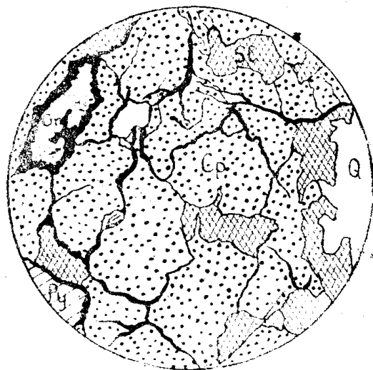
Рис. 4. Сетчатая структура замещения халькопирита (Cp) халькозином (черный). Sl—сфалерит; Gp—галенит; Py—пирит; Q—жильный минерал. Ув. 180.
