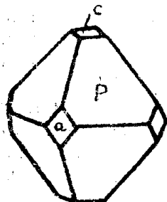
Рис. 1. Кристалл апофиллита P—(111); а—(100); с—(001).
