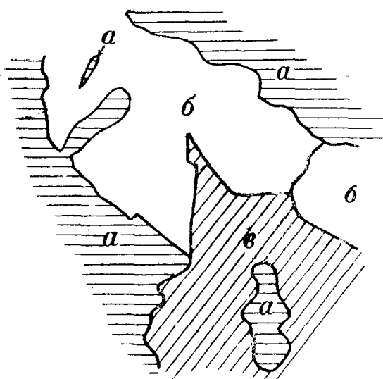
а - ферберит б - кварц в - антимонит
