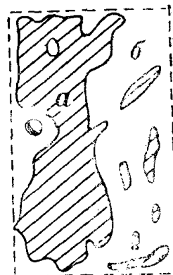
а - ферберит б - кварц
