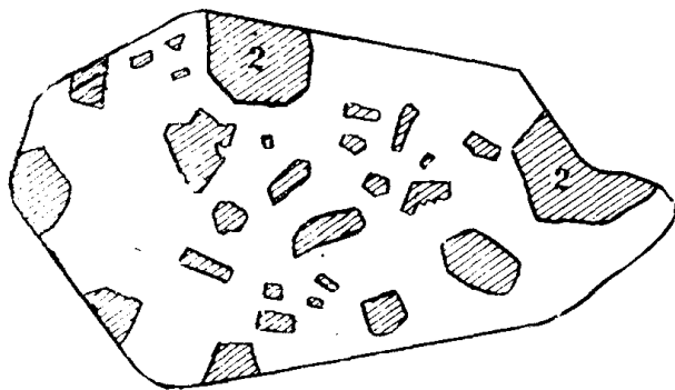
Ф. 5 Руда брекчиевидной текстуры 1-кварц с антимонитом; 2 обломки юрских сланцев с включением арсено- пирита; нат. вел. Херелизто
