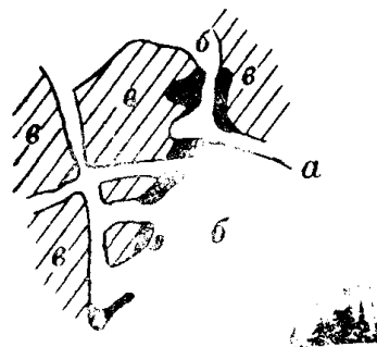
а - ферберит б - кварц в - обломки кремнистого сланца
