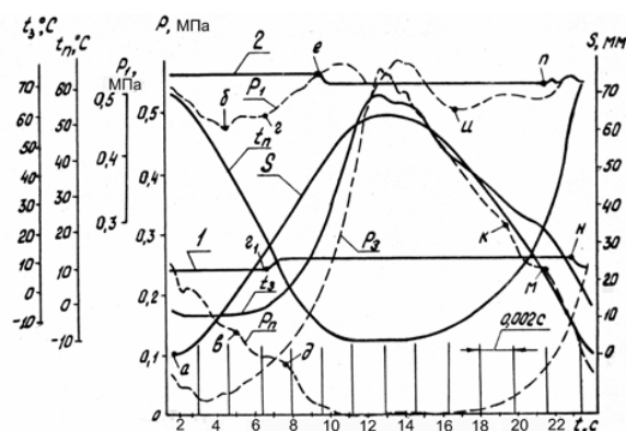
Рис. 2. Осциллограмма работы ударного узла: 1-2 – переключение клапанов передней и задней камер; P_3 , P_n , P_1 – давление воздуха в камерах; t_3 и t_n – температура воздуха в камерах; S – перемещение поршня
