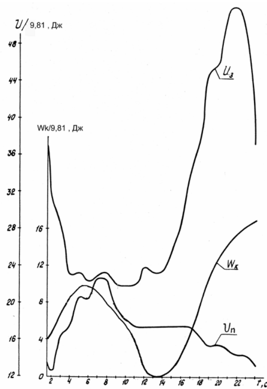
Рис. 7. Зависимость полной внутренней энергии сжатого воздуха в цилиндре и кинетической энергии поршня от времени: U_3 , U_n — в задней и передней камерах цилиндра; W_k — кинетическая энергия поршня
