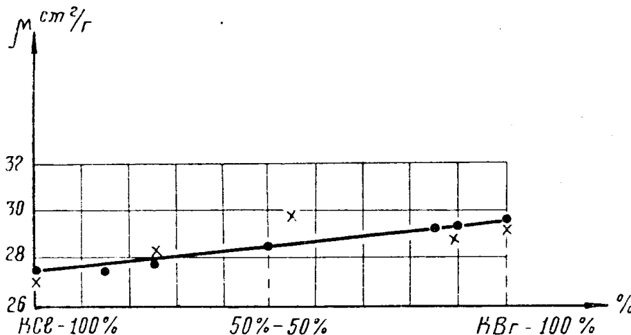
Рис. 1. Зависимость массового коэффициента ослабления \beta -излучения от химического состава твердых растворов KCl-KBr .
