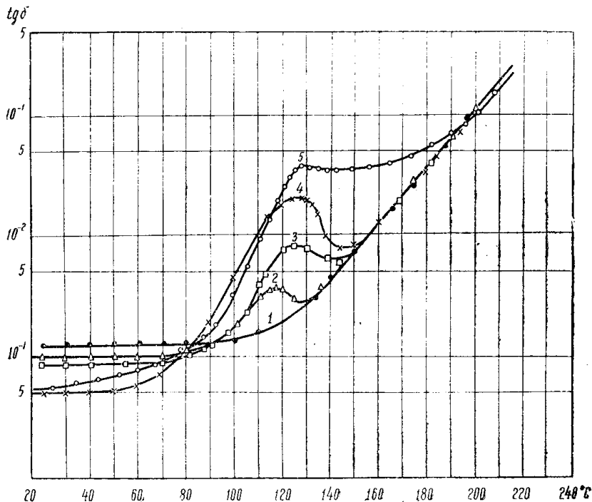
Рис. 1. Температурные зависимости \text{tg } \delta при 1000 гц для 1 — необлученных кристаллов КВг, облученных рентгеновскими лучами: 2 — 1,3 \cdot 10^{20} эв/см 3 , 3 — 5,2 \cdot 10^{20} эв/см 3 , 4 — 1,6 \cdot 10^{21} эв/см 3 , 5 — облученных протонами ( 2,0 \cdot 10^{23} эв/см 3 ).
