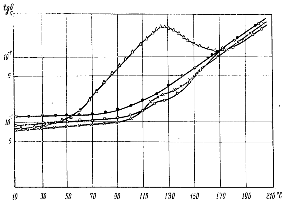
Рис. 2. Зависимости \text{tg} \delta от температуры при 100 гц для ●—●—●—●— необлученных кристаллов КJ; облученных рентгеновскими лучами ○—○—○—○— 1,3 \cdot 10^{21} эв/см 3 ×—×—×—×— 2,6 \cdot 21^{21} эв/см 3 , —△—△—△—△— облученных протонами ( 2,5 \cdot 10^{23} эв/см 3 ). (Цифрами указаны значения энергии излучения, поглощенной кристаллом).
