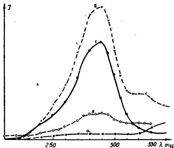
Рис. 2. Спектры возбуждения \text{NaCl}\cdot\text{Ce} : 1 — незакаленный 2 — после закалки от 450^\circ\text{C} , 3 — после облучения рентгеновскими лучами, а) \text{NaCl} ; фильтр УФС — 3.
