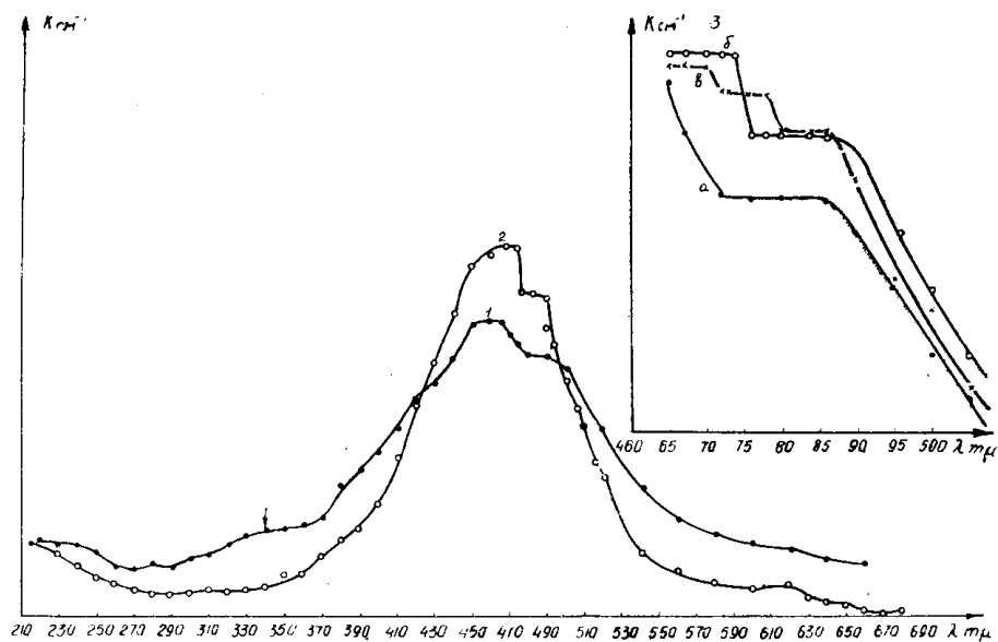
Рис. 3. Спектры поглощения кристаллов, облученных рентгеновскими лучами: 1 — \text{NaCl}\cdot\text{Sr}\cdot\text{Ce} , 2 — \text{NaCl}\cdot\text{Ce} , 3. — длинноволновая часть F -полосы после действия F -света: а — сразу после облучения, б — после действия F -света 10 мин, в — после действия F -света 30 мин.
