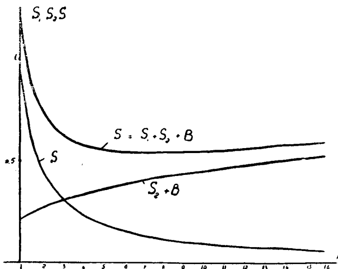
Рис. 1. Зависимость стоимости замены модулей и ее составляющих от количества модулей.
